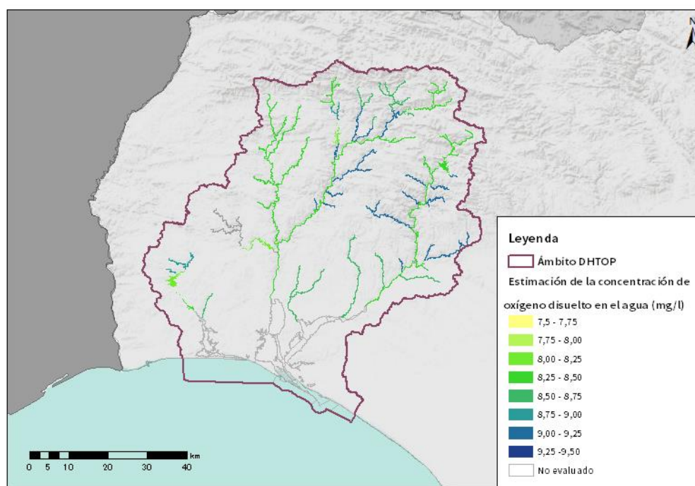
Figura nº 22. Estimación de la concentración de oxígeno disuelto en el agua (mgO 2 /l) calculada en función de la temperatura y la altitud en el mes de agosto
