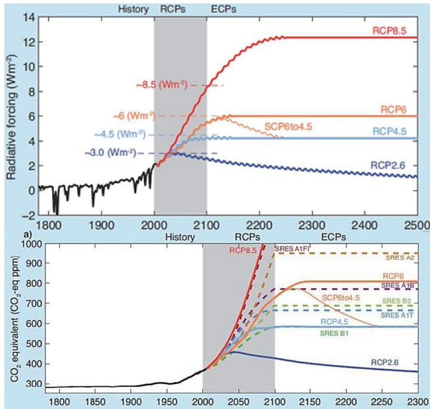
Figura nº 1. Escenarios de emisiones, con indicación del forzamiento radiativo (arriba) y la concentración de CO 2 equivalente en la atmósfera (debajo) (Fuente: IPCC, 2013)
