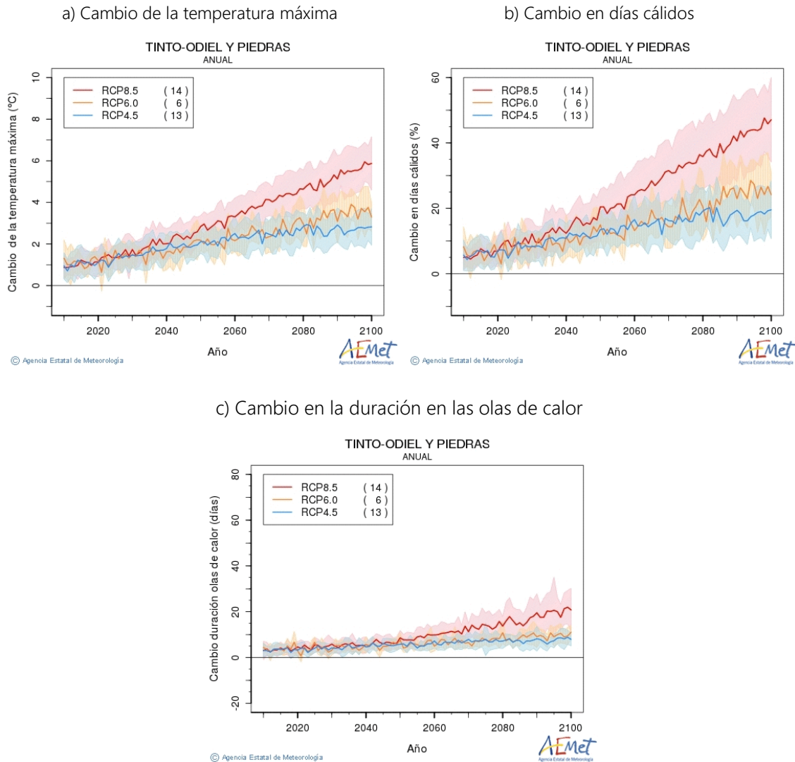
Figura nº 2. Gráficos de evolución anual de temperatura máxima (a), cambio en el número de días cálidos (b) y olas de calor (c) en la DHTOP a lo largo del siglo XXI (Fuente: AEMET, 2021).
