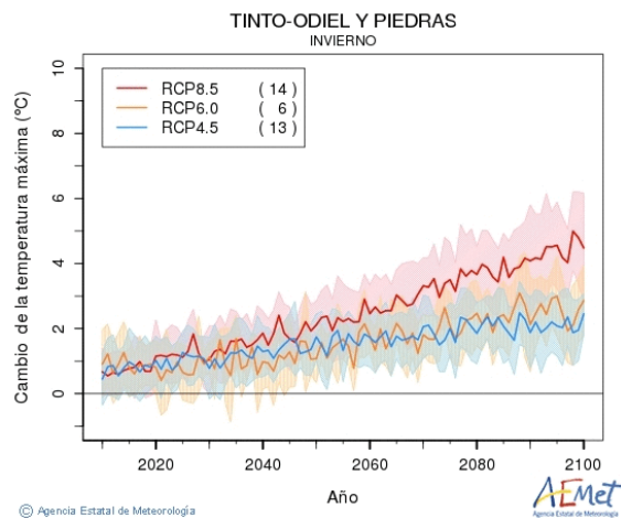
Figura nº 3. Gráficos de evolución temperatura máxima estacional en la DHTOP a lo largo del siglo XXI: primavera (a), verano (b), otoño (c) e invierno (d) (Fuente: AEMET, 2021)
