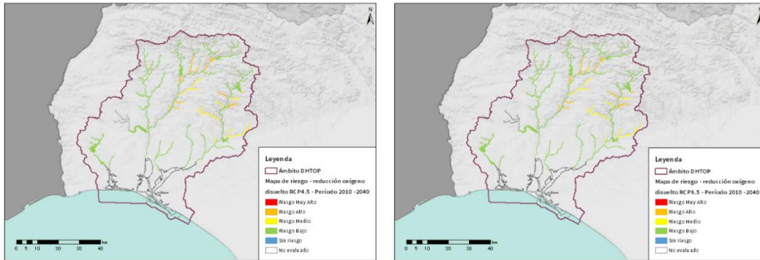
Figura nº 24. Mapa del riesgo de reducción del oxígeno disuelto para el corto plazo, 2010-2040. Escenarios RCP4.5 y RCP8.5.
