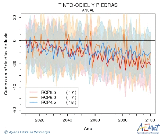
Figura nº 6. Gráficos de evolución anual de precipitación (a), cambio en precipitaciones intensas (b), cambio en periodos secos (c) y cambio en el número de días de lluvia (d) en la DHTOP a lo largo del siglo XXI (Fuente: AEMET, 2021).
