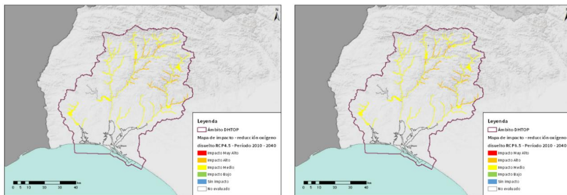
Figura nº 23. Mapa del impacto potencial sobre el oxígeno disuelto a corto plazo, 2010-2040. Escenarios RCP4.5 y RCP8.5.
