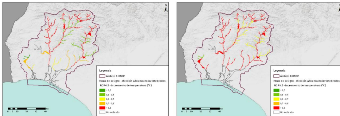
Figura nº 27. Mapa de peligro. Incremento esperado de la temperatura del agua para el corto plazo (2010-2040). Escenarios RCP4.5 y RCP8.5.
