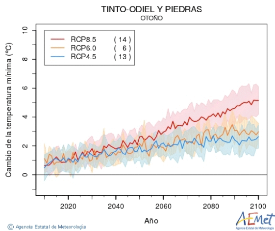
Figura nº 5. Gráficos de evolución temperatura mínima estacional en la DHTOP a lo largo del siglo XXI: primavera (a), verano (b), otoño (c) e invierno (d) (Fuente: AEMET, 2021)
