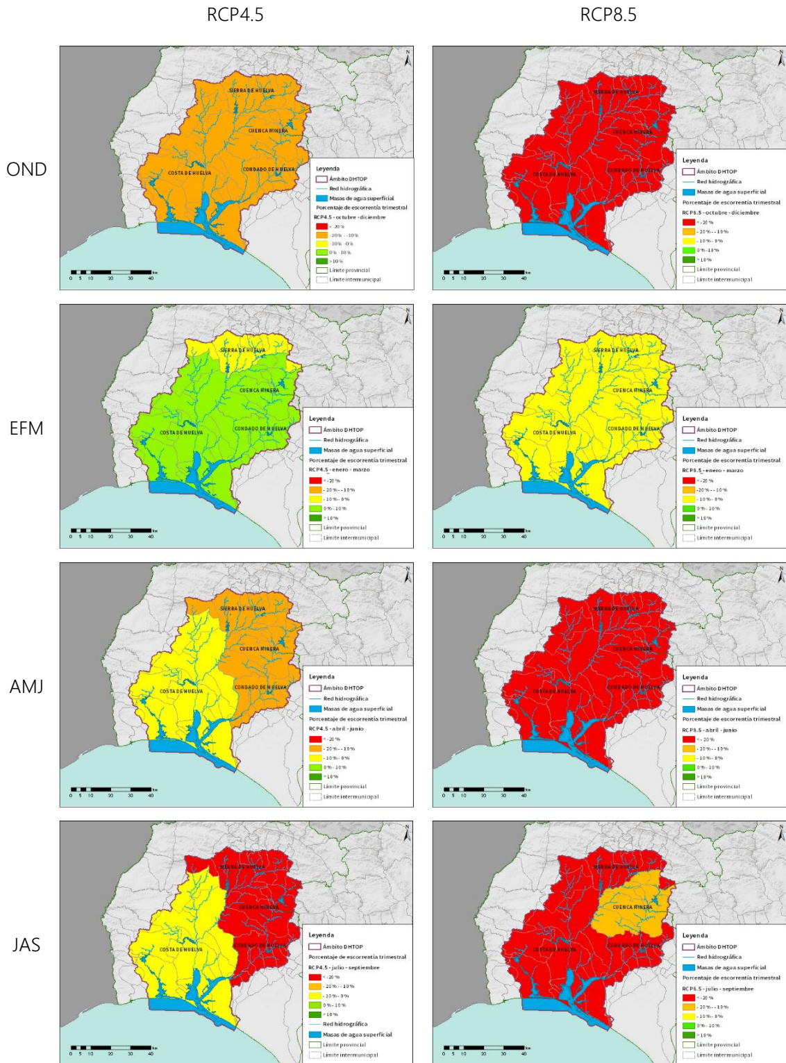
Figura nº 11. Porcentaje de cambio de la escorrentía trimestral (OND, EFM, AMJ, JAS) por sistema en la DHTOP para el horizonte 2039. Escenario RCP4.5 (izquierda) y RCP8.5 (derecha). Los colores reflejan la gradación del cambio
