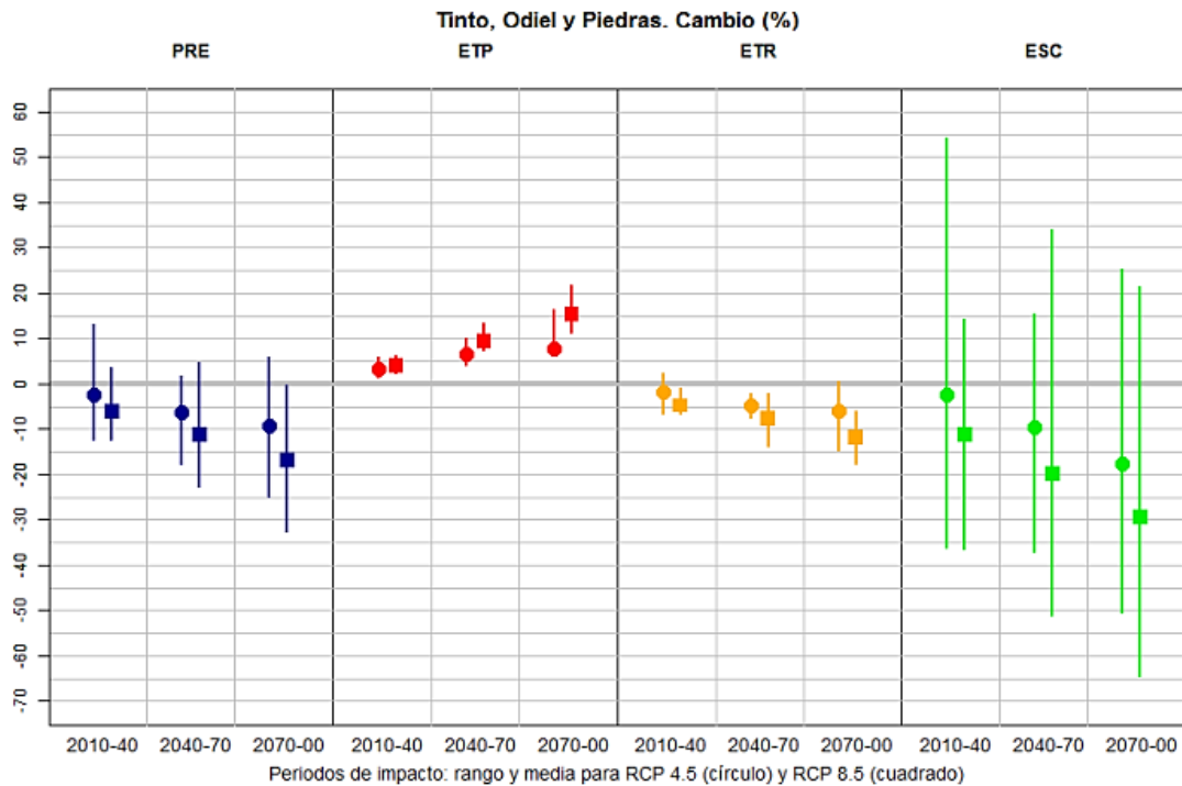
Figura nº 8. Cambio (%) en las principales variables hidrológicas en los tres PI respecto al PC para la DHTOP. Rango y media de resultados para RCP 4.5 (círculos) y RCP 8.5 (cuadrados). Fuente: CEDEX, 2017
