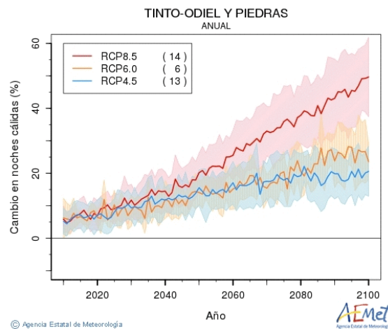
Figura nº 4. Gráficos de evolución anual de temperatura mínima (a), número de días de heladas (b) y noches cálidas (c) en la DHTOP a lo largo del siglo XXI (Fuente: AEMET, 2021)
