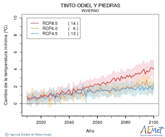
Figura nº 5. Gráficos de evolución temperatura mínima estacional en la DHTOP a lo largo del siglo XXI: primavera (a), verano (b), otoño (c) e invierno (d) (Fuente: AEMET, 2021)
