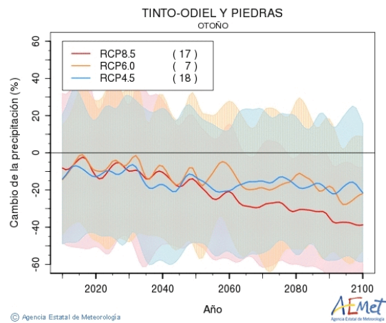
Figura nº 7. Gráficos de evolución precipitación estacional en la DHTOP a lo largo del siglo XXI: primavera (a), verano (b), otoño (c) e invierno (d) (Fuente: AEMET, 2021).
