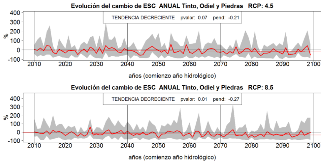
Figura nº 9. Tendencia del \Delta (%) escorrentía del año 2010 al 2099 para los RCP4.5 (arriba) y RCP8.5 (abajo) en la DHTOP (CEH, 2017).
