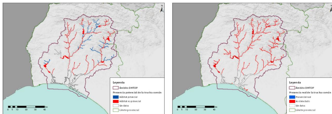
Figura nº 17. Mapa de Exposición. Hábitat potencial calculado con el límite termal de 21,8°C (izquierda) y adaptación de la presencia de la trucha común a las masas de agua superficiales (MMA, 2001) (derecha)
