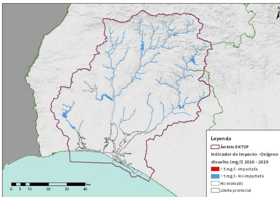
Figura nº 25. Estado actual del indicador O 2
