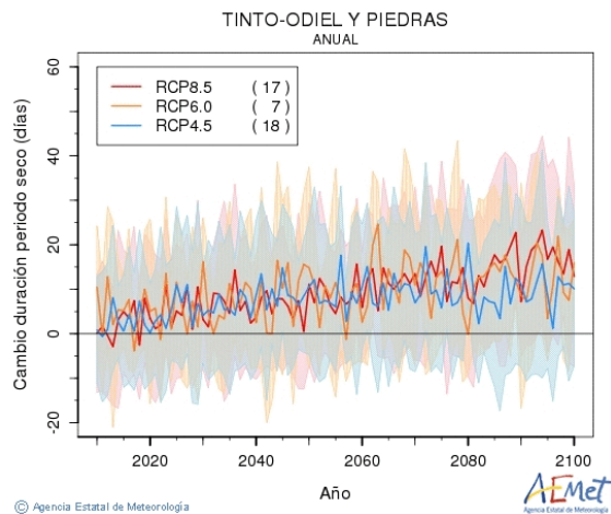
Figura nº 6. Gráficos de evolución anual de precipitación (a), cambio en precipitaciones intensas (b), cambio en periodos secos (c) y cambio en el número de días de lluvia (d) en la DHTOP a lo largo del siglo XXI (Fuente: AEMET, 2021).
