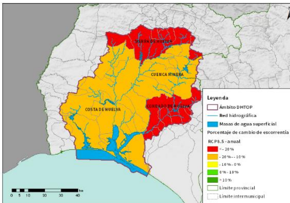
Figura nº 10. Porcentaje de cambio de la escorrentía medio anual por sistema en la DHTOP para el horizonte 2039. Escenario RCP4.5(izquierda) y RCP8.5 (derecha). Los colores reflejan la gradación del cambio
