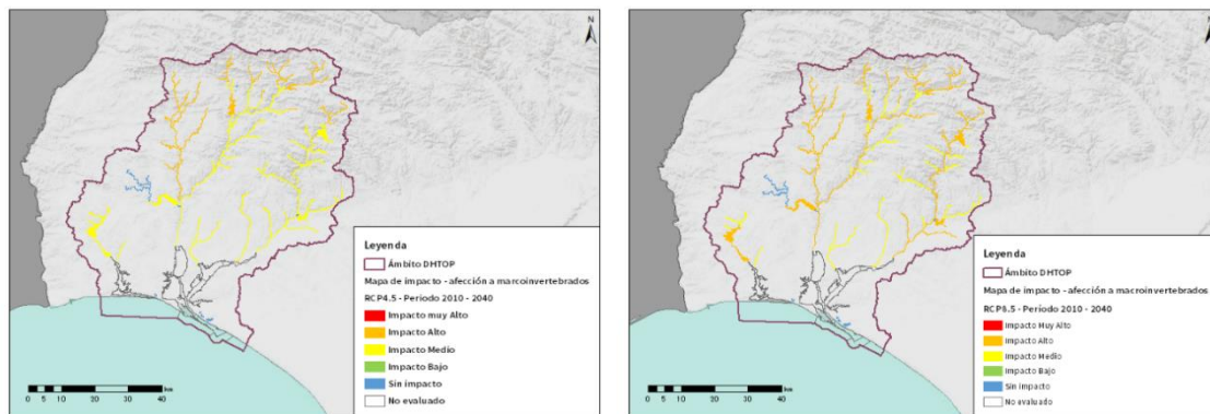
Figura nº 28. Mapa del impacto potencial sobre los macroinvertebrados según para el corto plazo (2010-2040). Escenarios RCP4.5 y RCP8.5.
