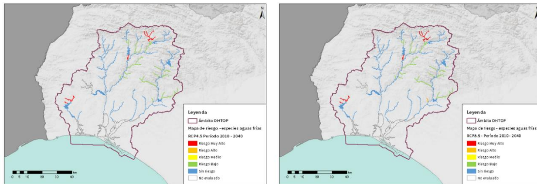
Figura nº 20. Mapa de riesgo de pérdida de hábitat para especies de aguas frías para el corto plazo, 2010-2040. Escenarios RCP4.5 y RCP8.5
