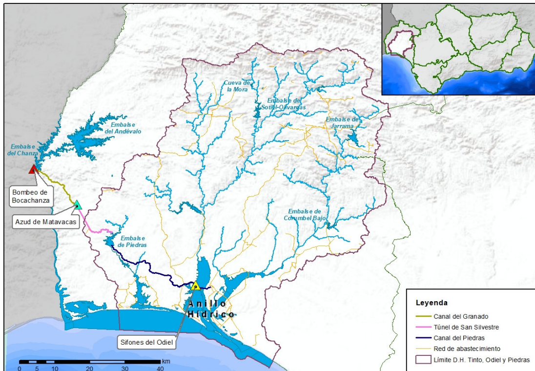
Figura nº 6. Principales infraestructuras para el abastecimiento.
