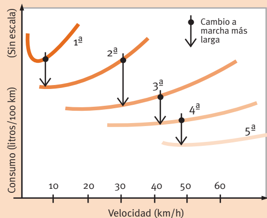
Consumo en función de la velocidad para las diferentes marchas de la caja de cambios
