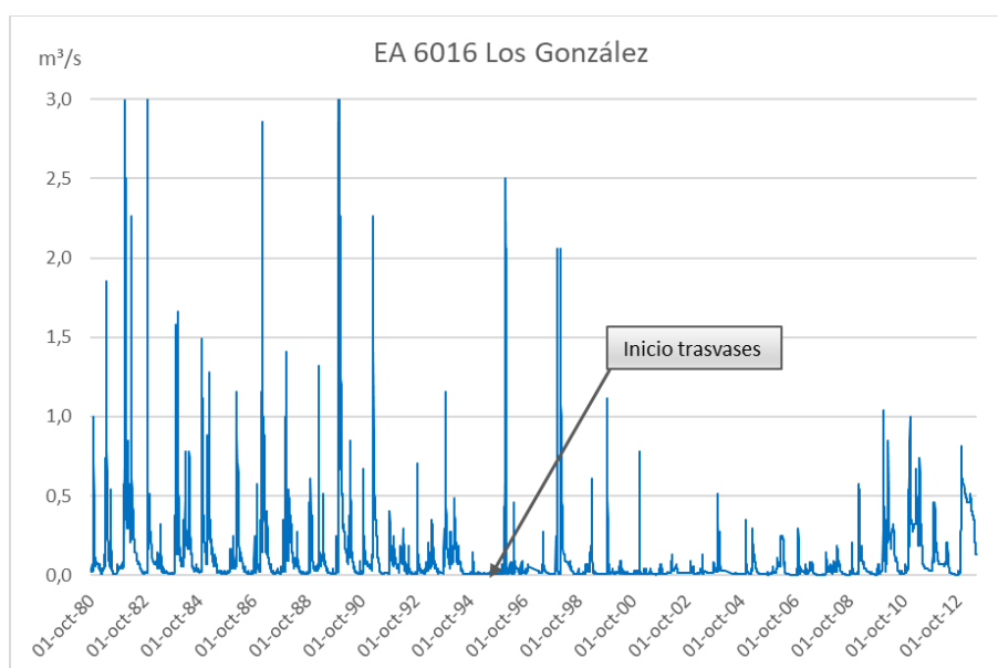
Figura nº 7. Afección al régimen de avenidas en el río Bermuza (masa de agua ES060MSPF0621030 Alcaucín-Bermuza) en la estación de aforos 6016 Los González tras la entrada en funcionamiento de los trasvases internos del Sistema Viñuela
