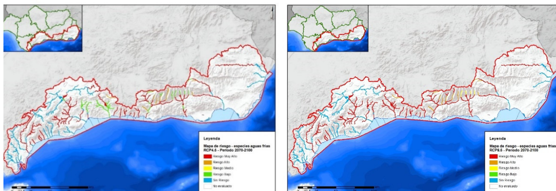
Figura nº 5. Mapas de riesgo sobre la pérdida de hábitat para especies de aguas frías para los dos escenarios de emisiones RCP4.5 (izquierda) y RCP8.5 (derecha), y los tres PI (2010-2040 arriba, 20140-2070 medio y 2017-2100 abajo)
