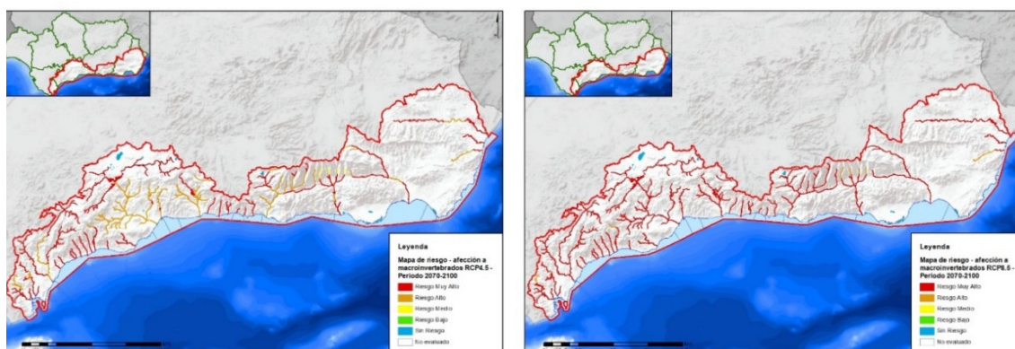
Figura nº 7. Mapas de riesgo en los macroinvertebrados para los dos escenarios de emisiones RCP4.5 (izquierda) y RCP8.5 (derecha), y los tres PI (2010-2040 arriba, 2040-2070 medio y 2070-2100 abajo)
