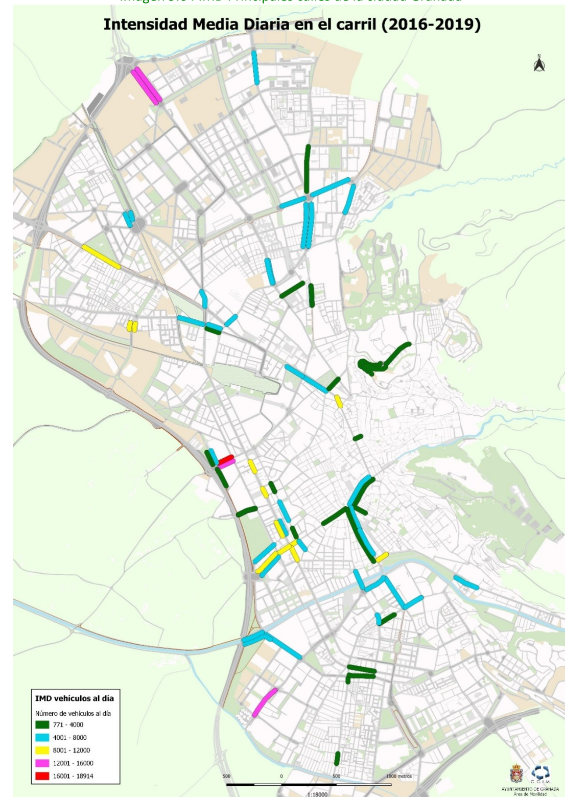
Imagen 9.64 IMD Principales calles de la ciudad Granada
