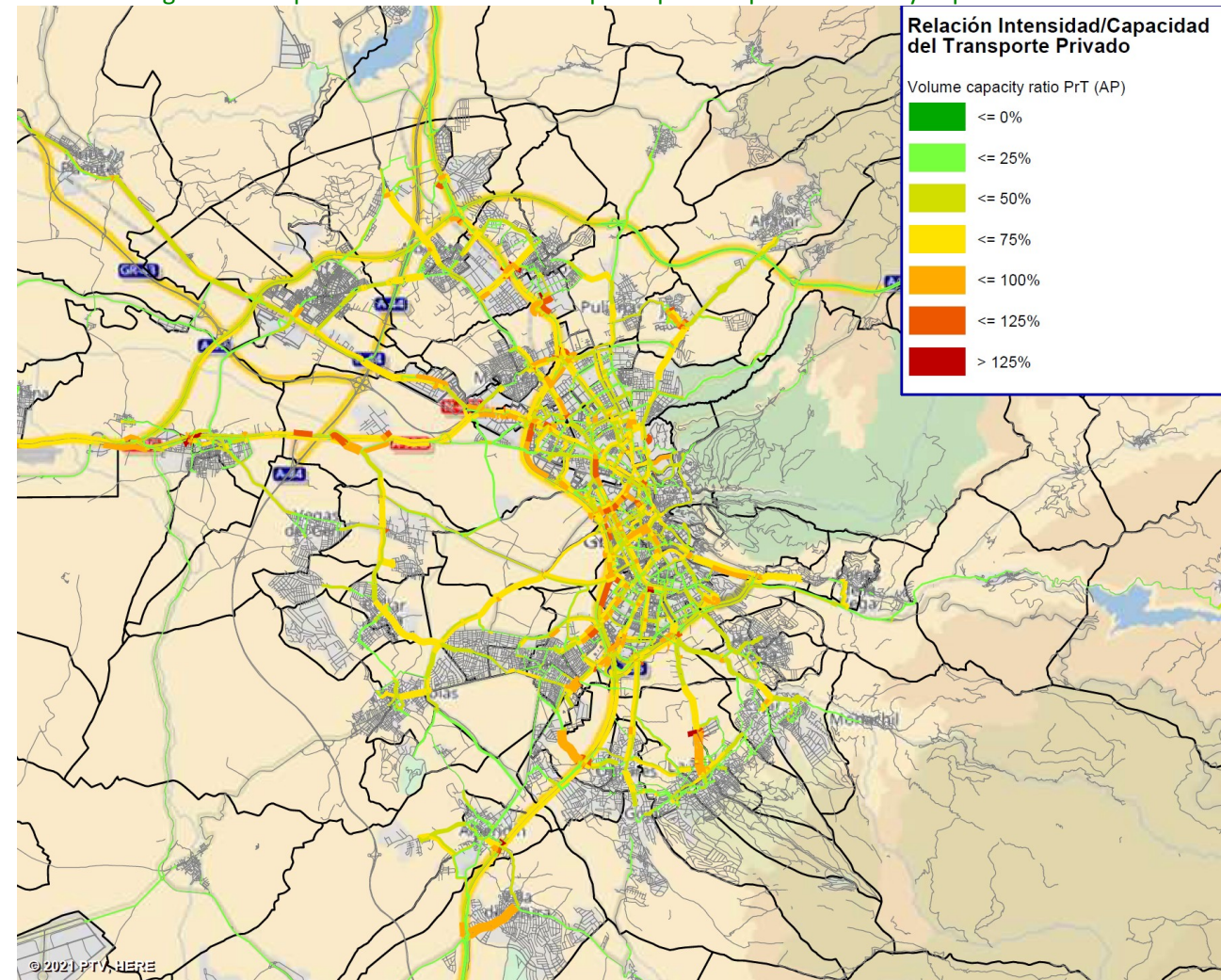
Imagen 9.65 Capacidad del viario en transporte privado para Granada y la primera corona.
