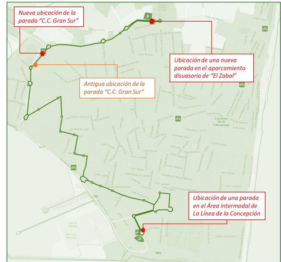
Figura 12.26: Modificaciones en la línea 2 de La Linea de la Concepción. (LL2)
