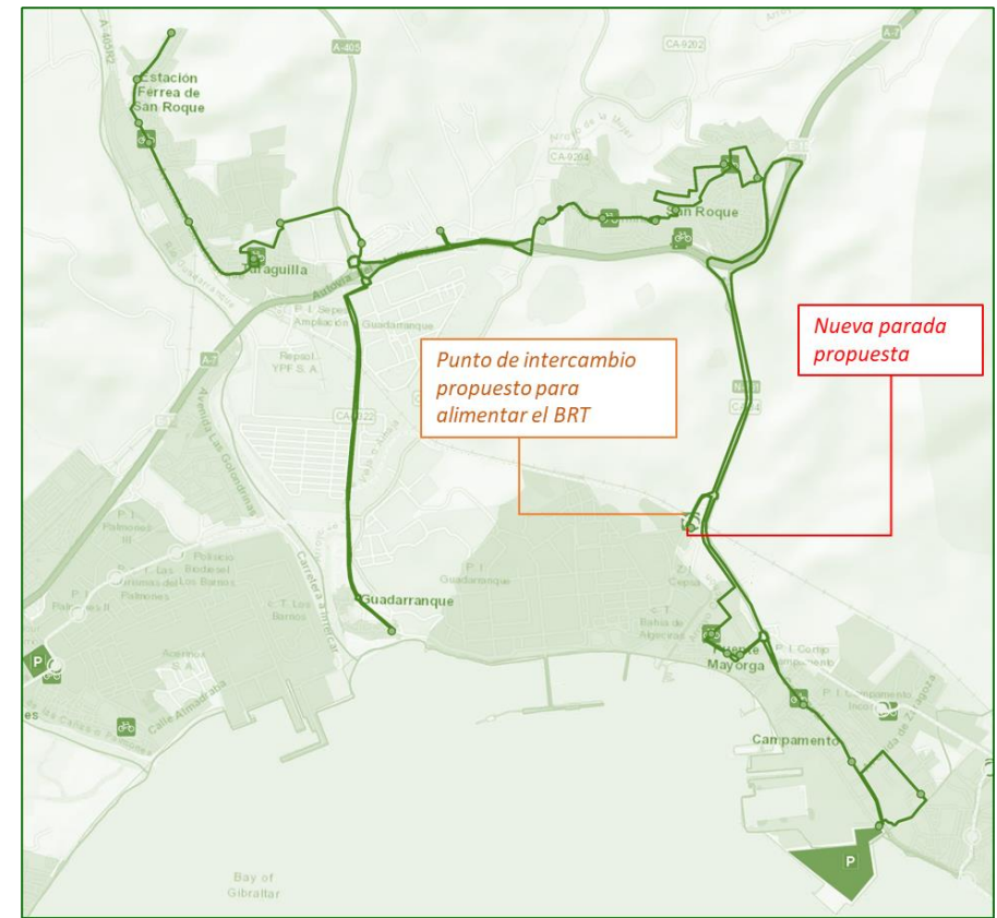
Figura 12.20: Modificaciones en la línea 4 de San Roque. (SR4)
