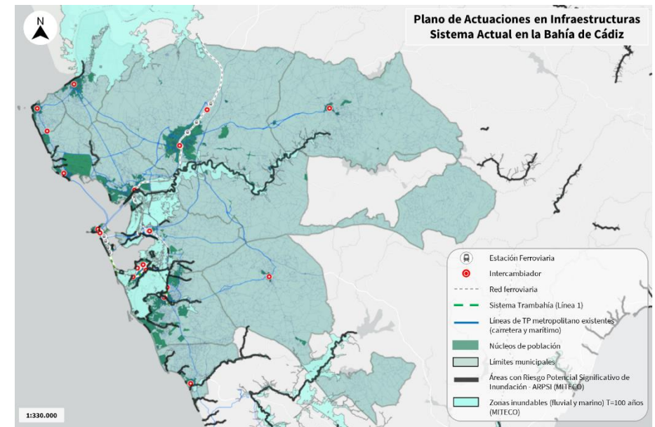
Figura 128: Infraestructuras de transporte sobre ARPSI y ZI de origen fluvial y marino (T=100 años)
