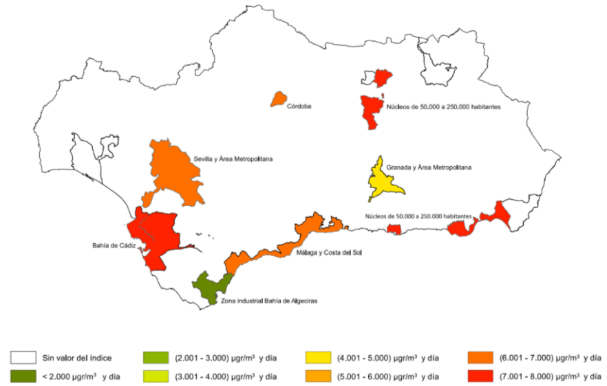
Figura 136: Índice de concentración media anual de ozono. 2022
