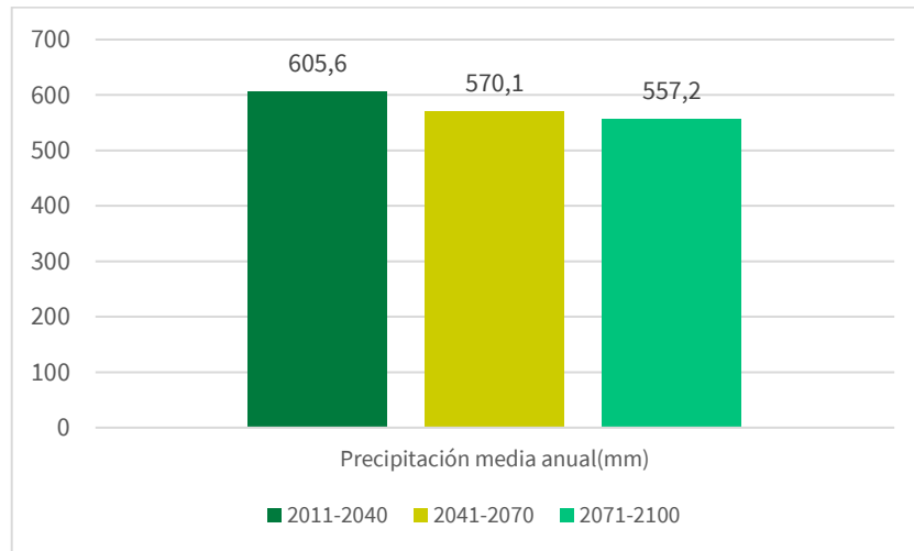
Figura 125: Evolución de la precipitación media anual (mm) en el ámbito del PTMBC.
