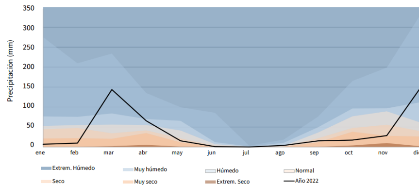
Figura 114: Evolución mensual de las precipitaciones en Andalucía. 2022
