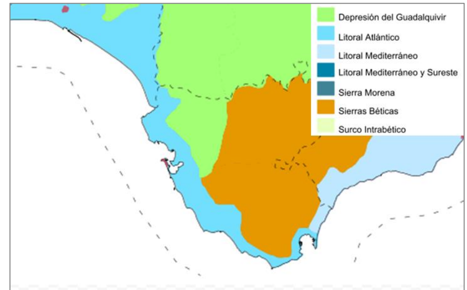
Figura 35: Regiones climáticas en la Bahía de Cádiz.
