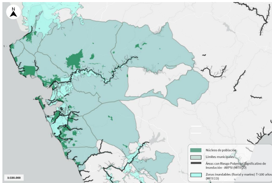
Figura 127: ARPSI y ZI de origen fluvial y marino (T=100 años)
