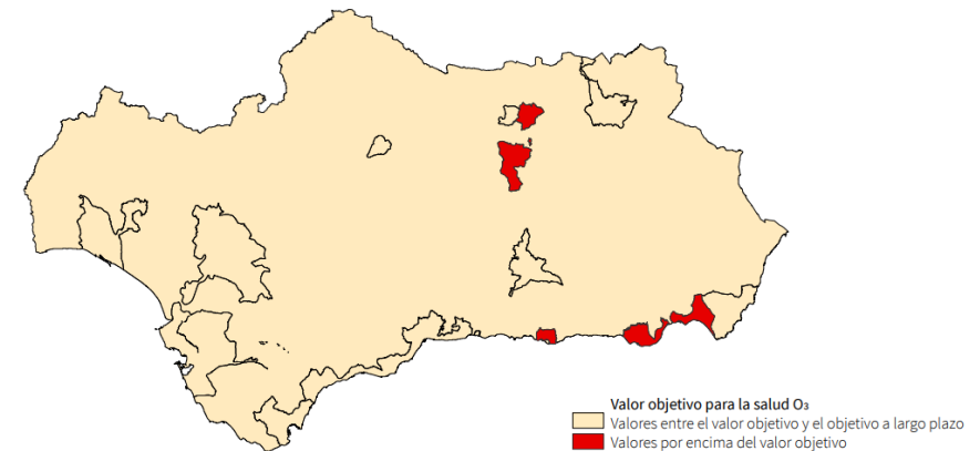
Figura 129: Evaluación del valor objetivo de ozono para la protección e la salud. 2022
