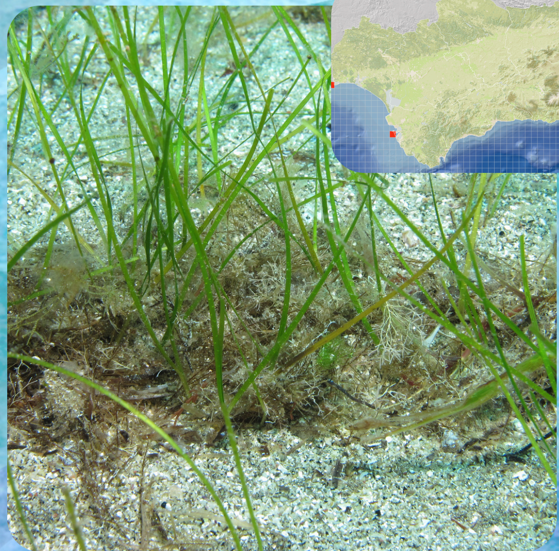
Zostera marina
