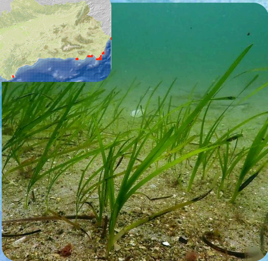
Zostera noltei
