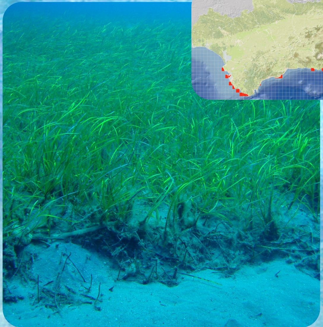
Cymodocea nodosa
