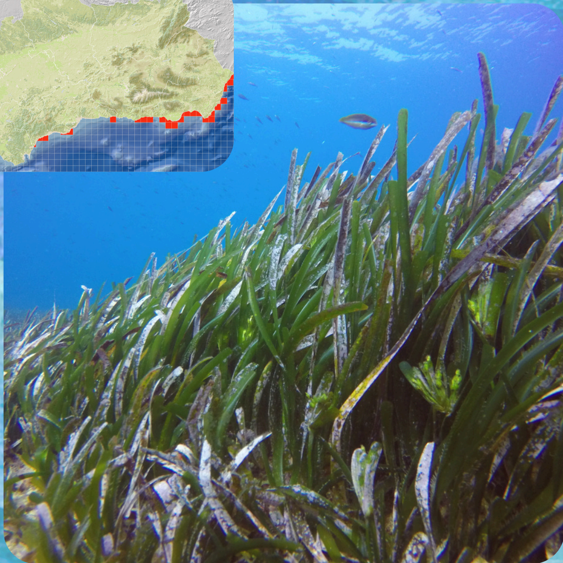
Posidonia oceanica
