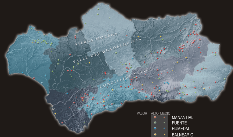
Mapa de tipos de surgencias significativas de Andalucía (Inventario provisional y abierto)
