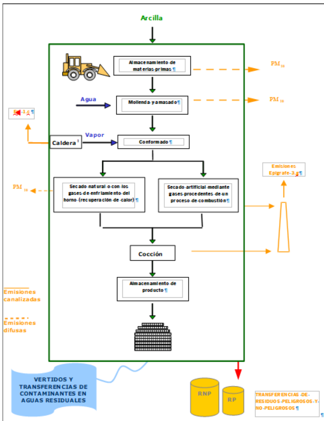
Figura 1. Diagrama del proceso de fabricación y emisiones asociadas
