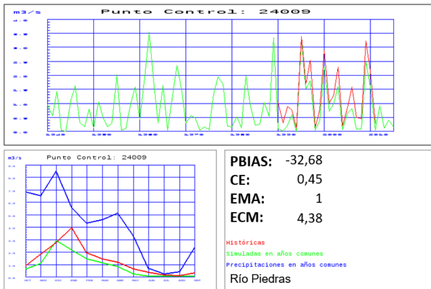
Figura nº 30. Contraste de las entradas al embalse de Piedras en el río Piedras
