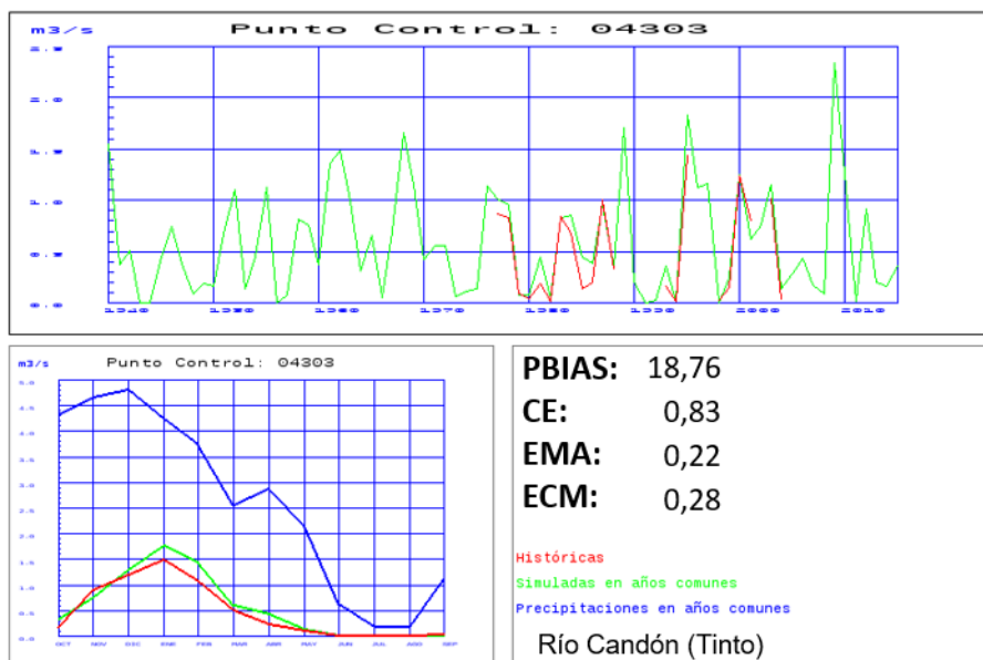
Figura nº 31. Contraste de los caudales anuales y medios mensuales en el río Candón
