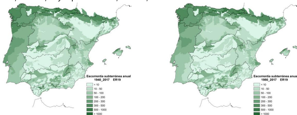
Figura nº 53. Distribución espacial de la escorrentía subterránea anual (mm): izquierda 1940/41-2017/18, derecha 1980/81-2017/18
