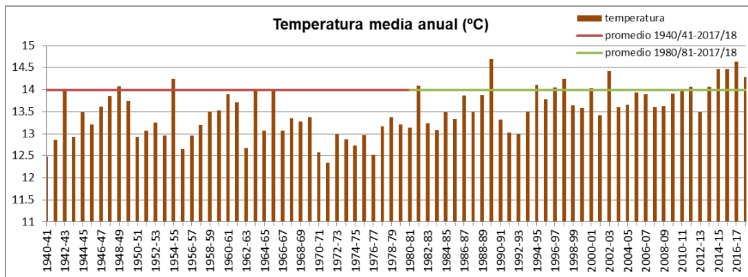
Figura nº 39. Serie de temperatura media anual en España
