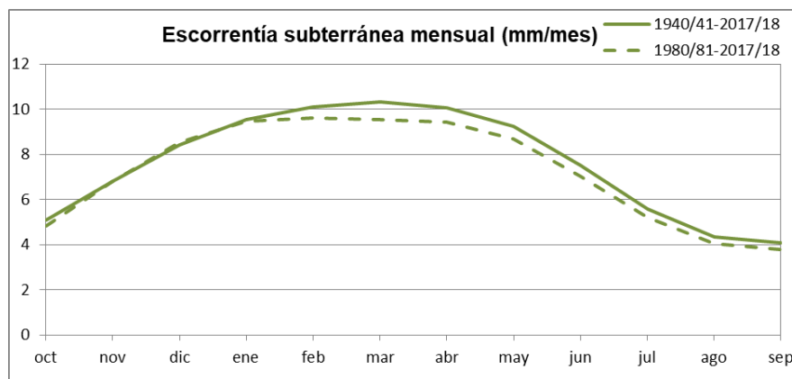
Figura nº 55. Serie de promedios mensuales de escorrentía subterránea en la Península y Baleares, 1940/41-2017/18 y 1980/81-2017/18
