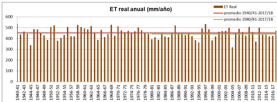
Figura nº 45. Serie de evapotranspiración real anual en la Península y Baleares
