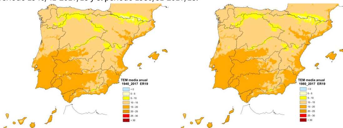
Figura nº 36. Distribución espacial de la temperatura media anual (°C): izquierda 1940/41-2017/18, derecha 1980/81-2017/18
