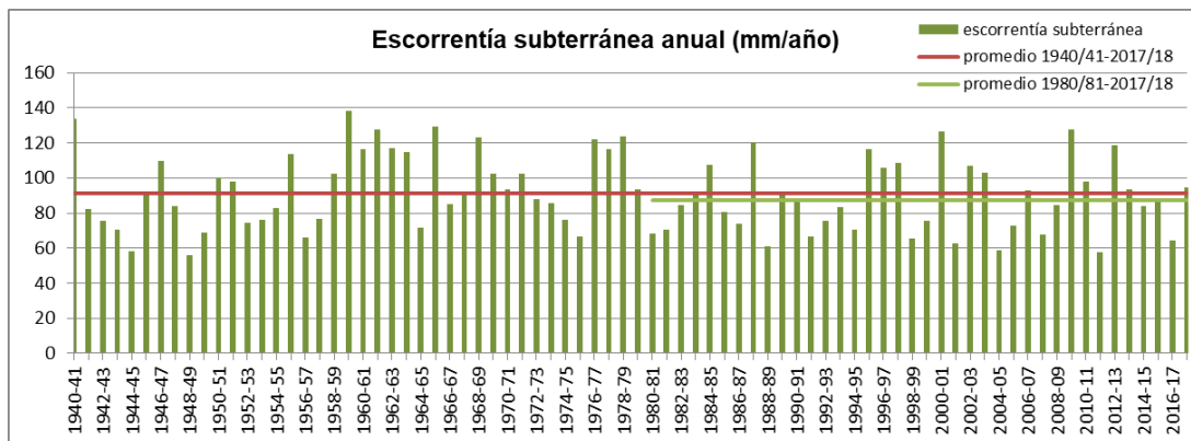
Figura nº 54. Serie de escorrentía subterránea anual en la Península y Baleares
