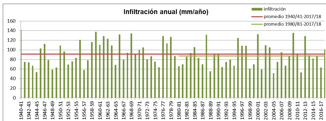
Figura nº 51. Serie de infiltración anual en la Península y Baleares
