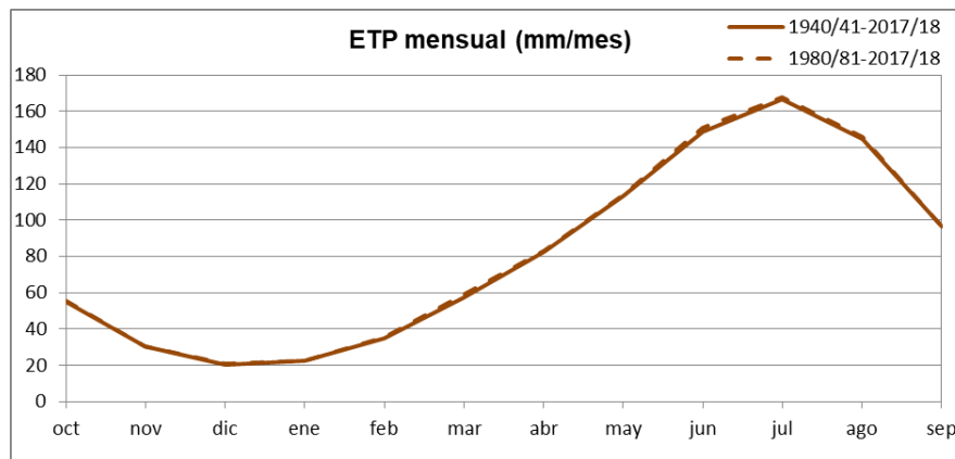
Figura nº 43. Serie de promedios mensuales de evapotranspiración potencial en España, 1940/41-2017/18 y 1980/81-2017/18
