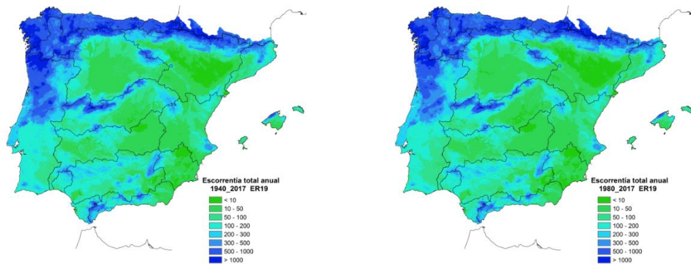
Figura nº 59. Distribución espacial de la escorrentía total anual (mm): izquierda 1940/41-2017/18, derecha 1980/81-2017/18
