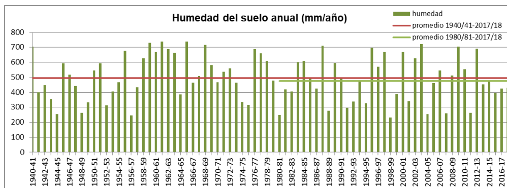
Figura nº 48. Serie de humedad del suelo anual en la Península y Baleares
