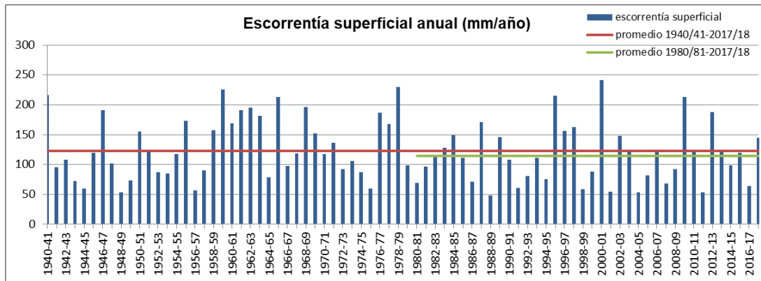
Figura nº 57. Serie de escorrentía superficial anual en la Península y Baleares
