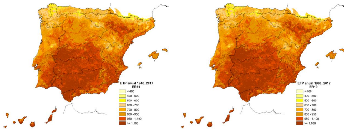
Figura nº 41. Distribución espacial de la evapotranspiración potencial anual (mm): izquierda 1940/41-2017/18, derecha 1980/81-2017/18
