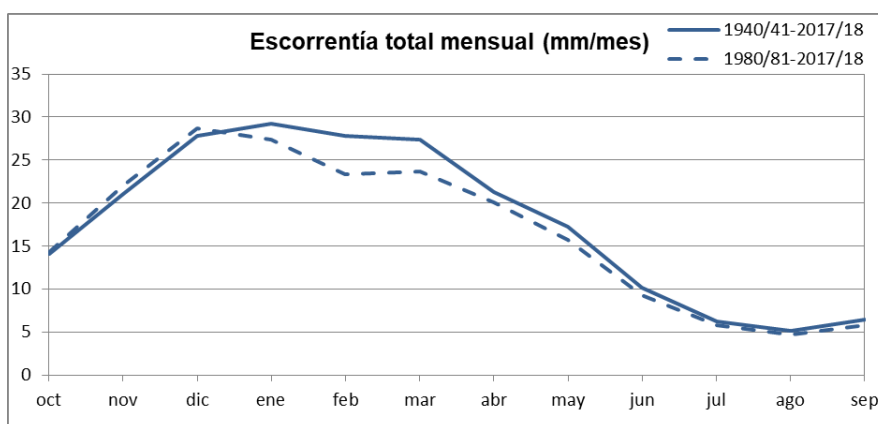
Figura nº 62. Serie de promedios mensuales de escorrentía total en la Península y Baleares, 1940/41-2017/18 y 1980/81-2017/18
