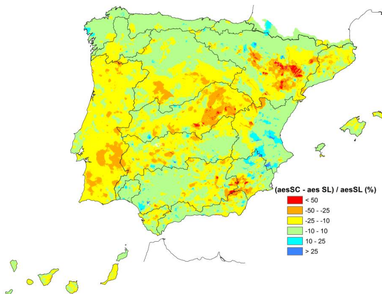
Figura nº 60. Porcentaje de cambio de la escorrentía anual, comparativa de la serie corta respecto de la serie larga
