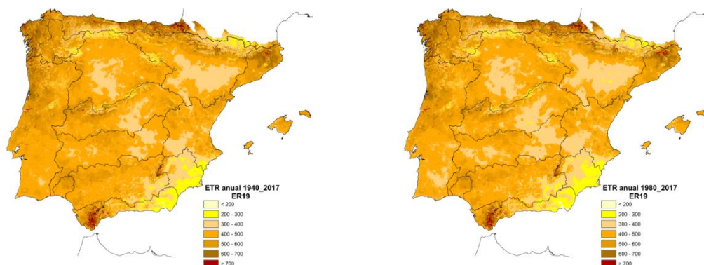
Figura nº 44. Distribución espacial de la evapotranspiración real anual (mm): izquierda 1940/41-2017/18, derecha 1980/81-2017/18
