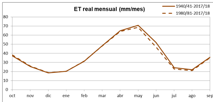
Figura nº 46. Serie de promedios mensuales de evapotranspiración real en la Península y Baleares, 1940/41-2017/18 y 1980/81-2017/18
