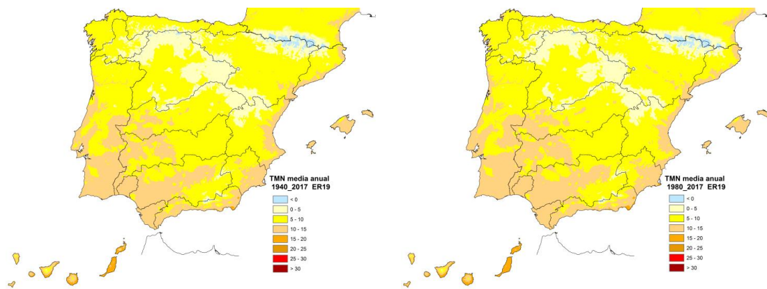
Figura nº 37. Distribución espacial de la temperatura mínima media anual: izquierda 1940/41-2017/18, derecha 1980/81-2017/18
