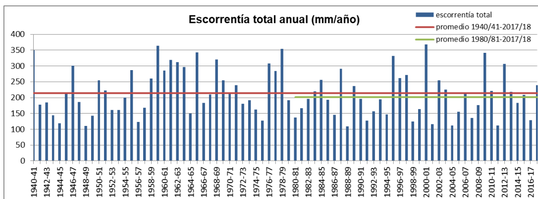
Figura nº 61. Serie de escorrentía total anual en la Península y Baleares
