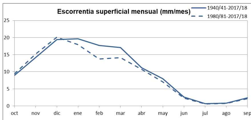
Figura nº 58. Serie de promedios mensuales de escorrentía superficial en la Península y Baleares, 1940/41-2017/18 y 1980/81-2017/18
