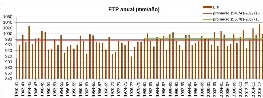
Figura nº 42. Serie de evapotranspiración potencial anual en España
