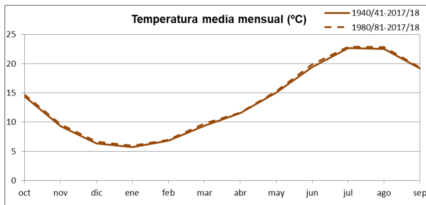
Figura nº 40. Serie de promedios mensuales de temperatura media en España, 1940/41-2017/18 y 1980/81-2017/18
