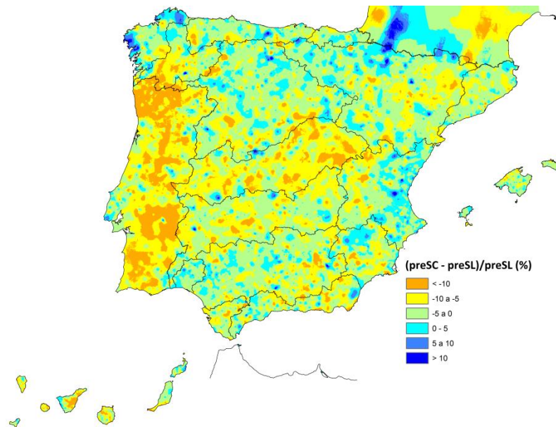
Figura nº 33. Porcentaje de cambio de la precipitación anual, comparativa serie corta respecto de la serie larga
