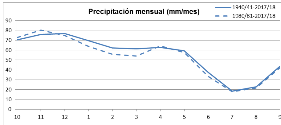
Figura nº 35. Serie de promedios mensuales de precipitación en España, 1940/41-2017/18 y 1980/81-2017/18
