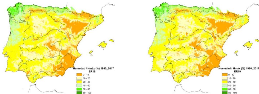
Figura nº 47. Distribución espacial del porcentaje de la humedad de suelo respecto a la humedad máxima en el año medio: izquierda 1940/41-2017/18, derecha 1980/81-2017/18
