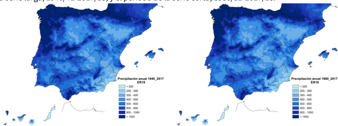
Figura nº 32. Distribución espacial de la precipitación total anual (mm): izquierda 1940/41-2017/18, derecha 1980/81-2017/18
