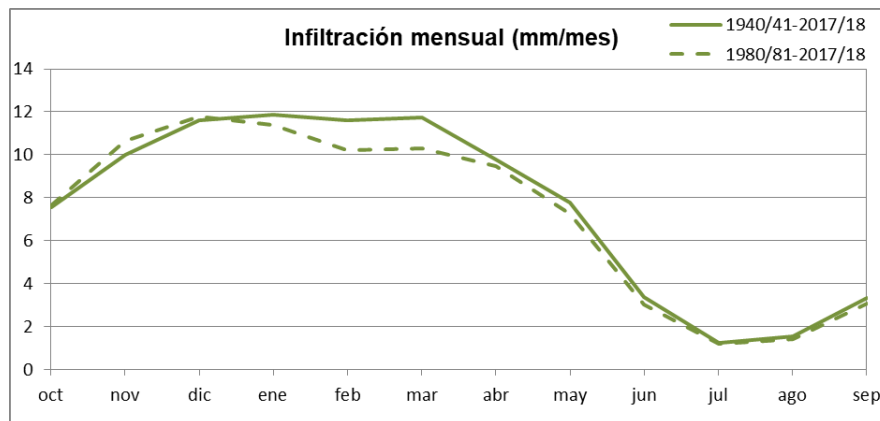
Figura nº 52. Serie de promedios mensuales de infiltración en la Península y Baleares, 1940/41-2017/18 y 1980/81-2017/18
