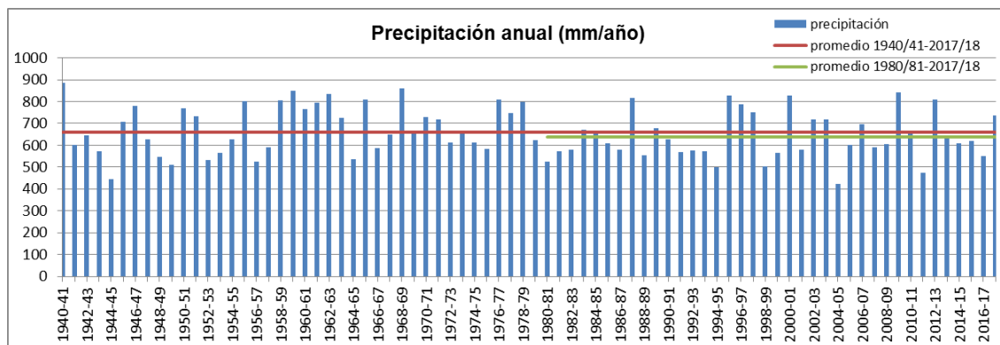
Figura nº 34. Serie de precipitación anual en España
