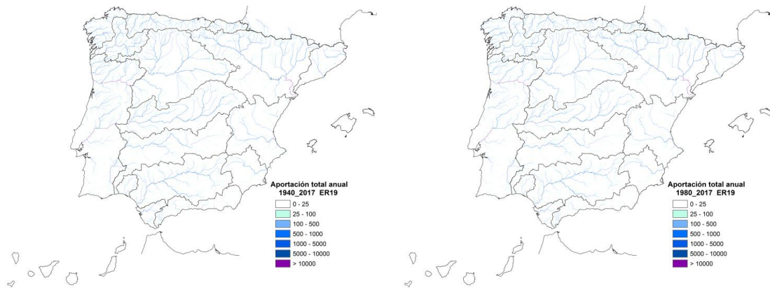
Figura nº 63. Distribución espacial de la aportación total anual (hm 3 /año): izquierda 1940/41-2017/18, derecha 1980/81-2017/18
