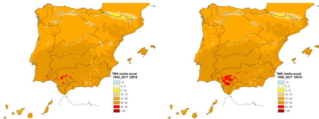
Figura nº 38. Distribución espacial de la temperatura máxima media anual: izquierda 1940/41-2017/18, derecha 1980/81-2017/18
