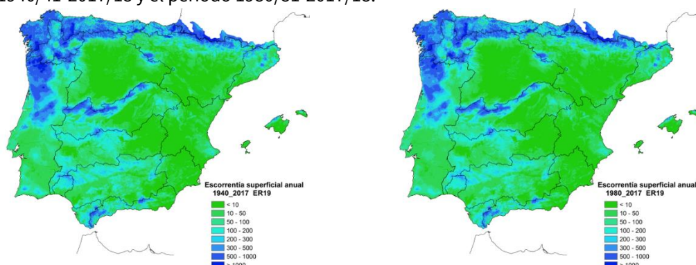
Figura nº 56. Distribución espacial de la escorrentía superficial anual (mm): izquierda 1940/41-2017/18, derecha 1980/81-2017/18
