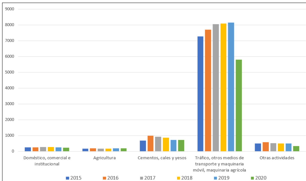
Figura 6.59. Evolución de las emisiones inventariadas de NO x (t/año)
