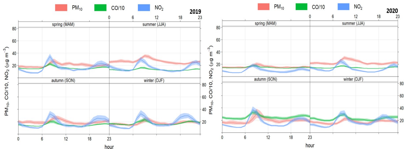
Figura 6.10. Patrón horario estacional para NO 2 , PM 10 y CO en 2019 y 2020. Estación El Atabal
