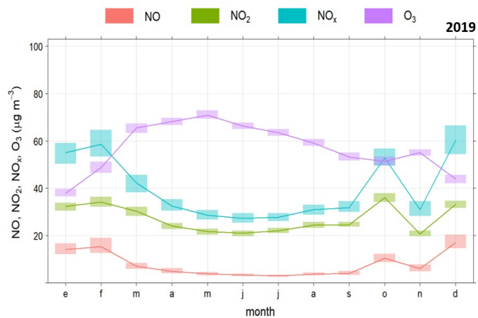
Figura 6.24. Medias mensuales de O 3 , NO x , NO 2 y NO en los años 2019 y 2020. Estación Carranque
