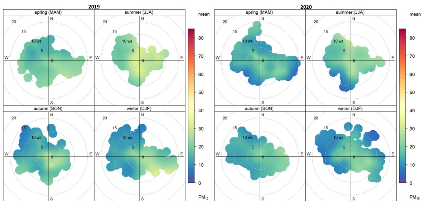
Figura 6.41. Relación entre los niveles horarios de PM_{10} y la velocidad y dirección del viento en 2019 y 2020. Estación Campanillas
