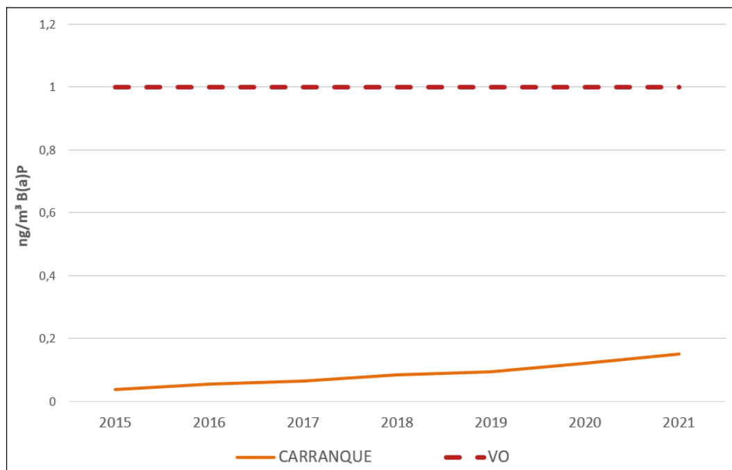
Figura 5.16. Medias anuales de B(a)P (ng/m³) en Málaga y Costa del Sol
