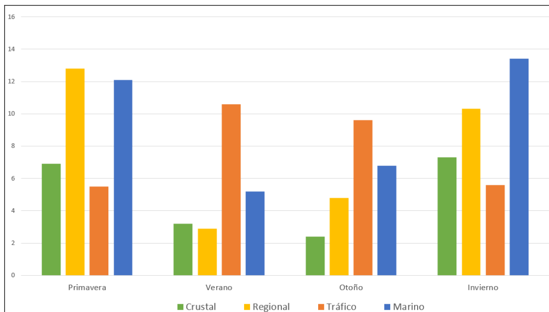
Figura 6.29. Contribución de fuentes por estaciones durante el año 2021 para PM 10 en la estación de Marbella Arco
