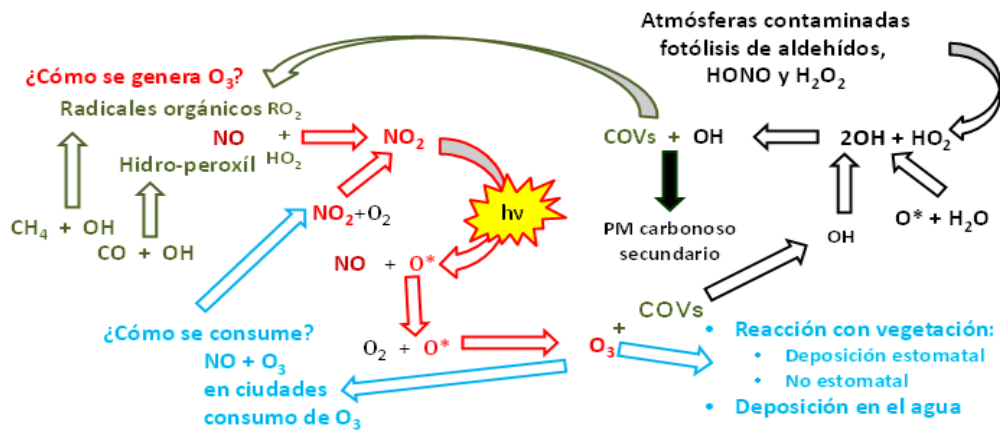
Figura I - 1. Procesos de generación y consumo de O 3 , basado en US-EPA (1996).
