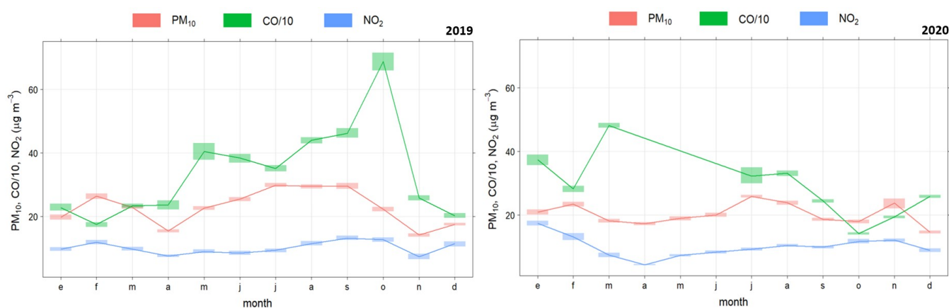
Figura 6.3. Medias mensuales de NO_2 , PM_{10} y CO en los años 2019 y 2020. Estación Campanillas
