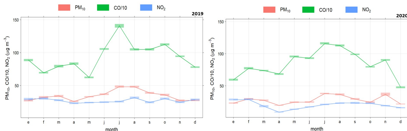
Figura 6.1. Medias mensuales de \text{NO}_2 , \text{PM}_{10} y \text{CO} en los años 2019 y 2020. Estación Marbella Arco
