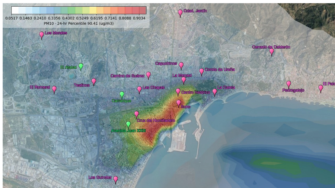
Figura AII.6. Contribución del tráfico marítimo al percentil 90,41 de los valores medios diarios de PM 10 . Escenario 1 (1 crucero + 1 ferry)
