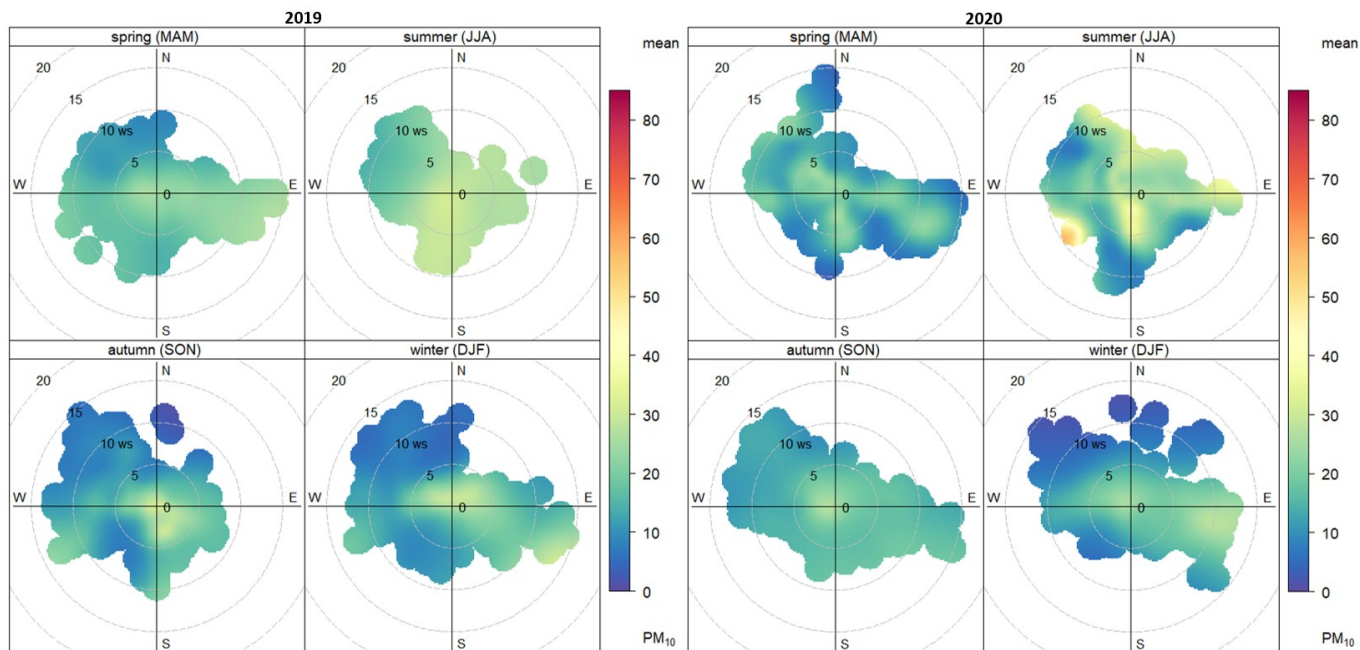
Figura 6.40. Relación entre los niveles horarios de PM_{10} y la velocidad y dirección del viento en 2019 y 2020. Estación Carranque
