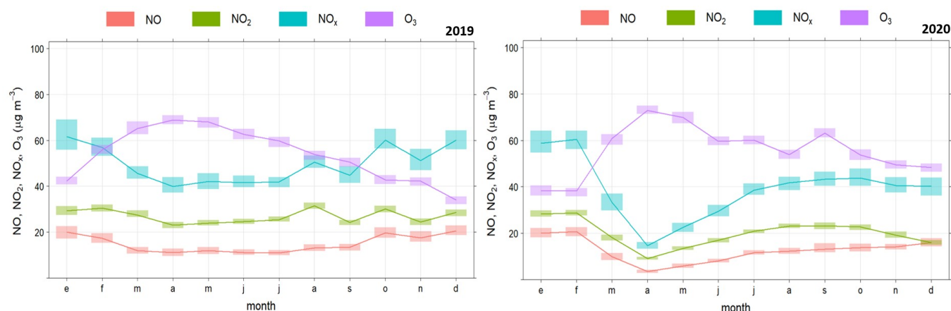
Figura 6.23. Medias mensuales de O 3 , NO x , NO 2 y NO en los años 2019 y 2020. Estación Marbella Arco
