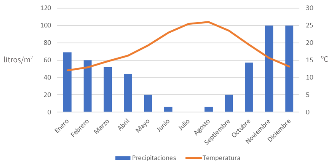
Figura 4.6. Distribución de las precipitaciones y la temperatura media (AEMET)
