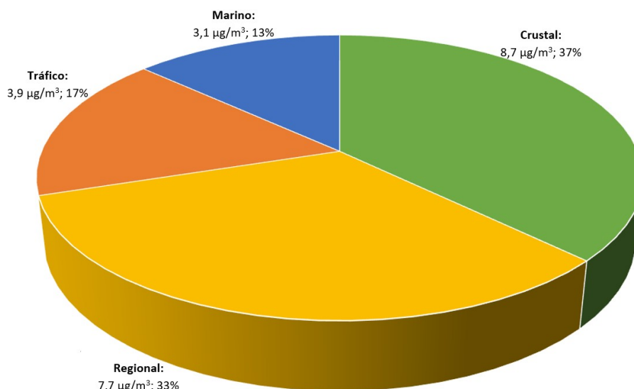
Figura 6.56. Contribución de fuentes en el periodo 2021 para PM 10 en la estación de Carranque
