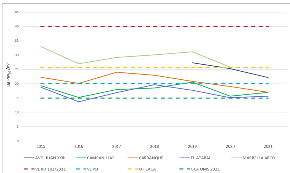
Figura 5.3. Promedio anual de PM_{10} ( \mu g/m^3 ) en Málaga y Costa del Sol
