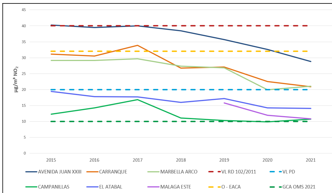
Figura 5.9. Promedio anual de NO 2 (µg/m 3 ) en Málaga y Costa del Sol
