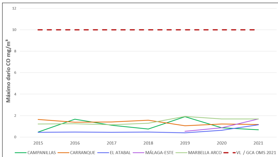
Figura 5.8. Máxima diaria de las medias móviles octohorarias de monóxido de carbono ( \text{mg}/\text{m}^3 ) en Málaga y Costa del Sol
