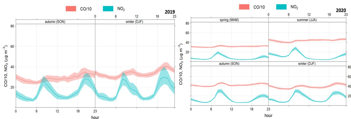
Figura 6.12. Patrón horario estacional para NO 2 y CO en 2019 y 2020. Estación Málaga Este
