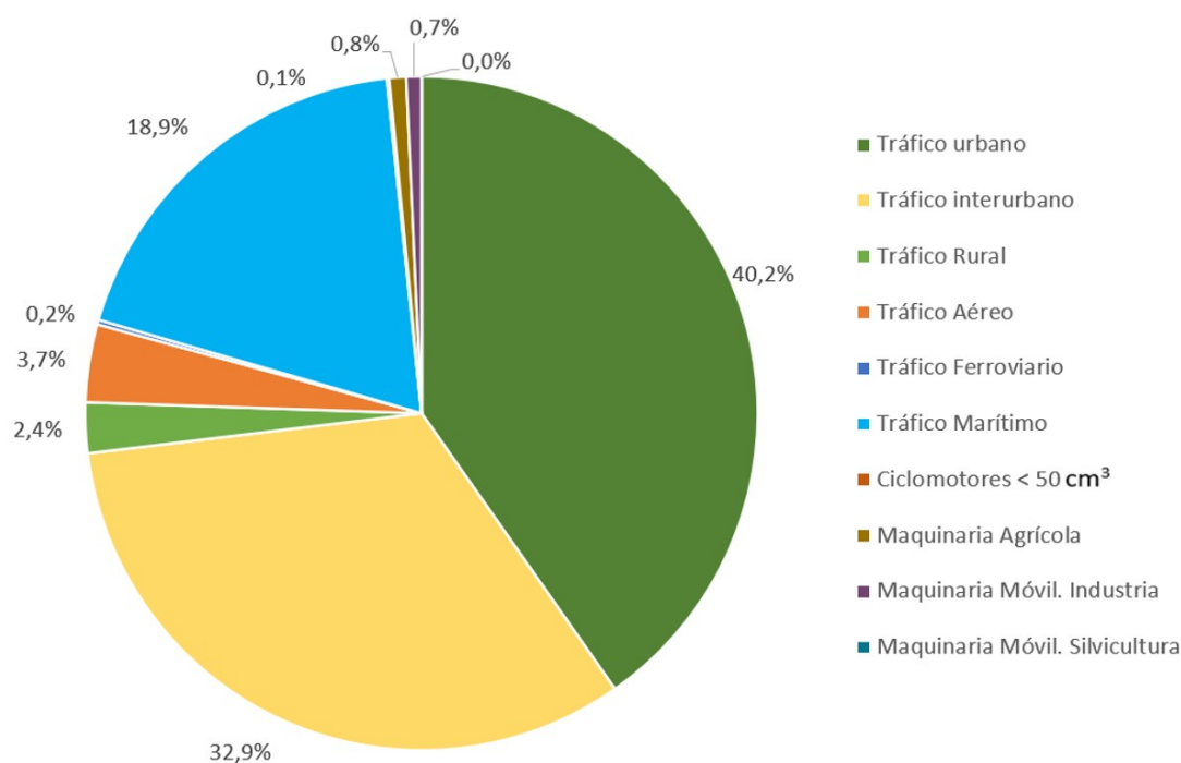
Figura 6.60. Distribución emisiones de NO x (t/año) en subsectores de tráfico en 2020
