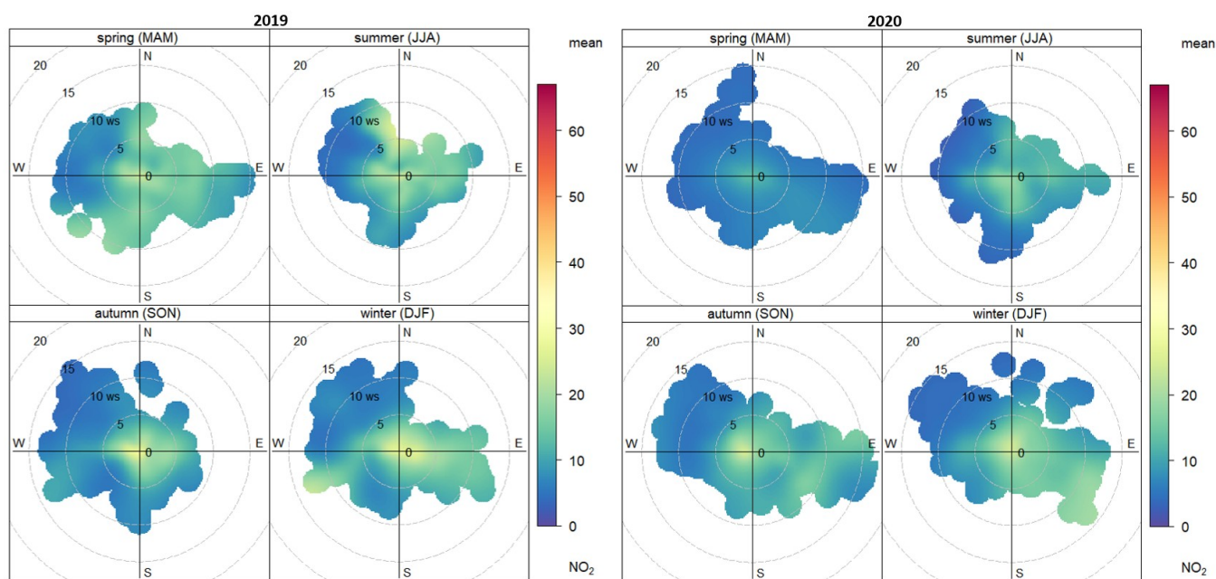
Figura 6.36. Relación entre los niveles horarios de \text{NO}_2 y la velocidad y dirección del viento en 2019 y 2020. Estación El Atabal
