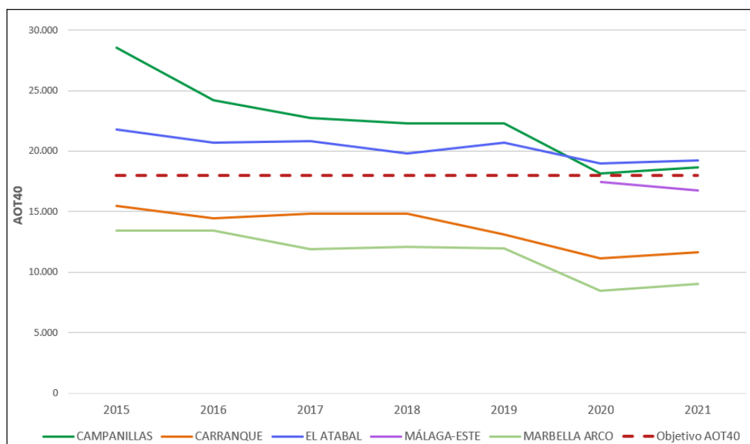
Figura 5.12. AOT40 ( \mu\text{g}/\text{m}^3 \cdot \text{h} ) calculada para Málaga y Costa del Sol
