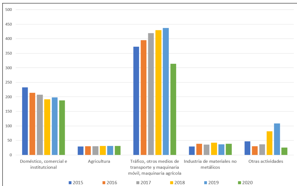
Figura 6.62. Evolución de las emisiones inventariadas de PM 2,5 (t/año)
