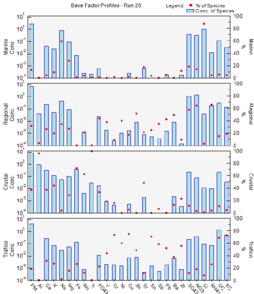
Figura 6.57. Perfil químico de las fuentes de PM 10 (expresado como contribución de elementos mayores y traza en µg/m 3 ) determinadas en la estación de Carranque en el año 2021
