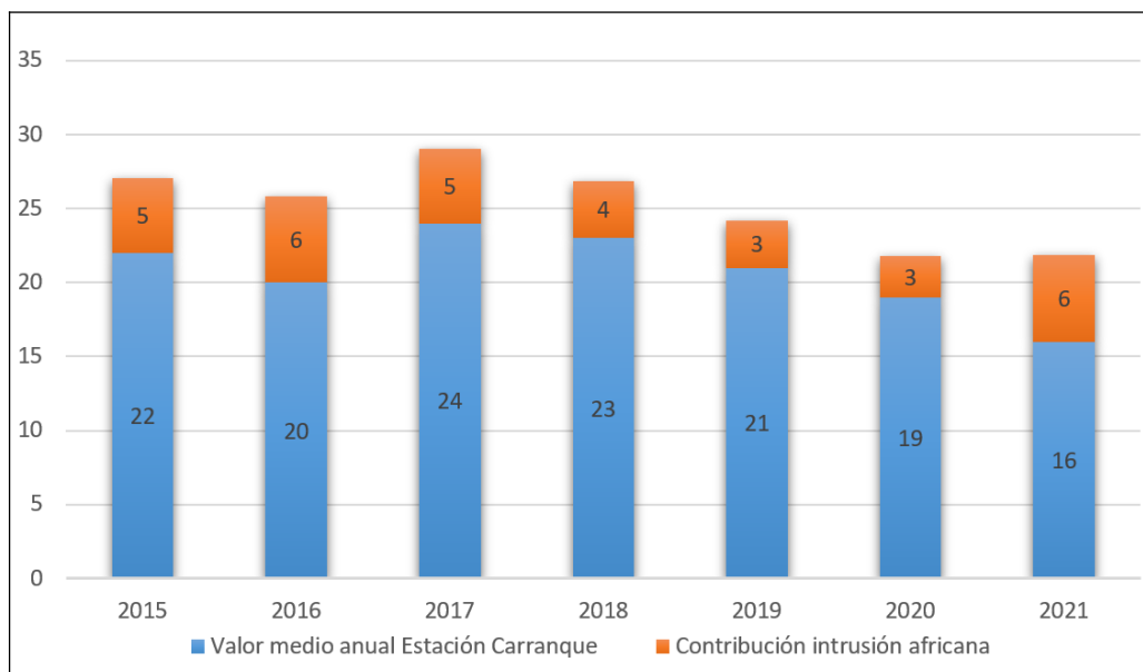
Figura 5.38. Contribución de la carga neta de polvo africano al valor medio anual. Estación Carranque 9
