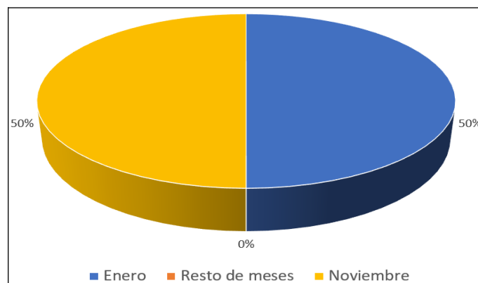
Figura 6.22. Distribución mensual de las superaciones del valor límite diario de PM 10 en el periodo 2015-2020. Estación Avda. Juan XXIII
