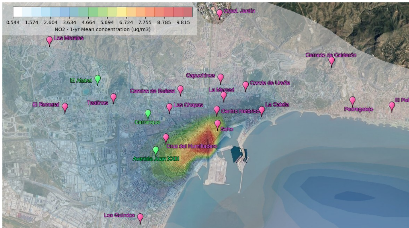
Figura AII.11. Contribución del tráfico marítimo a la media anual de los valores de \text{NO}_2 . Escenario 3 (3 cruceros + 1 ferry)
