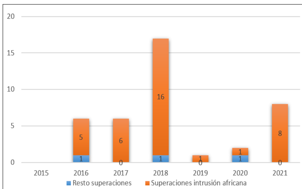
Figura 5.31. Origen y cuantificación del número de superaciones diarias de PM_{10} ( \mu g/m^3 ) en la estación de Campanillas 3
