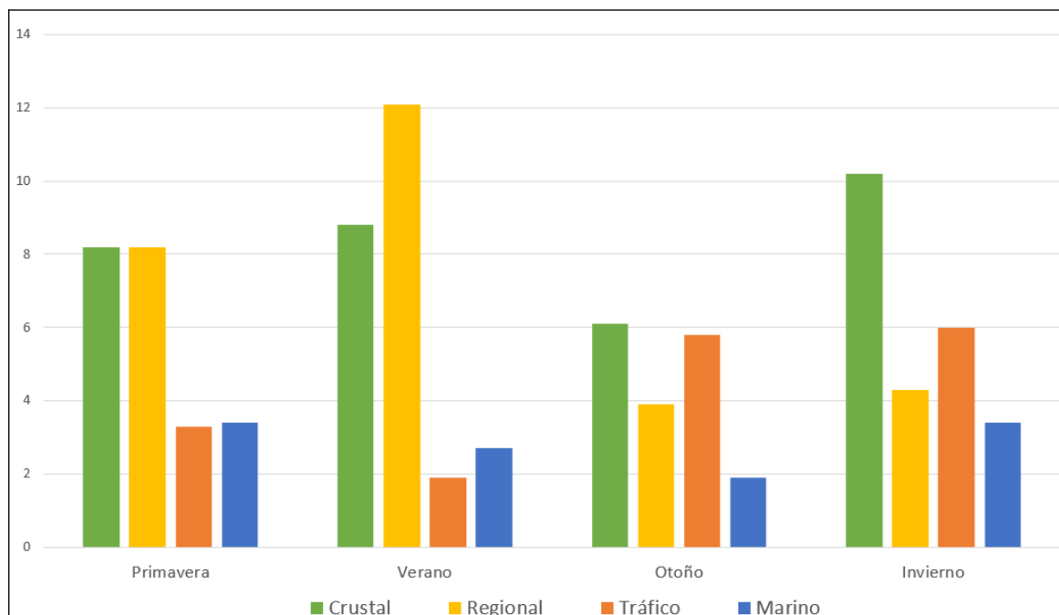
Figura 6.58. Contribución de fuentes por estaciones durante el año 2021 para PM 10 en la estación de Carranque
