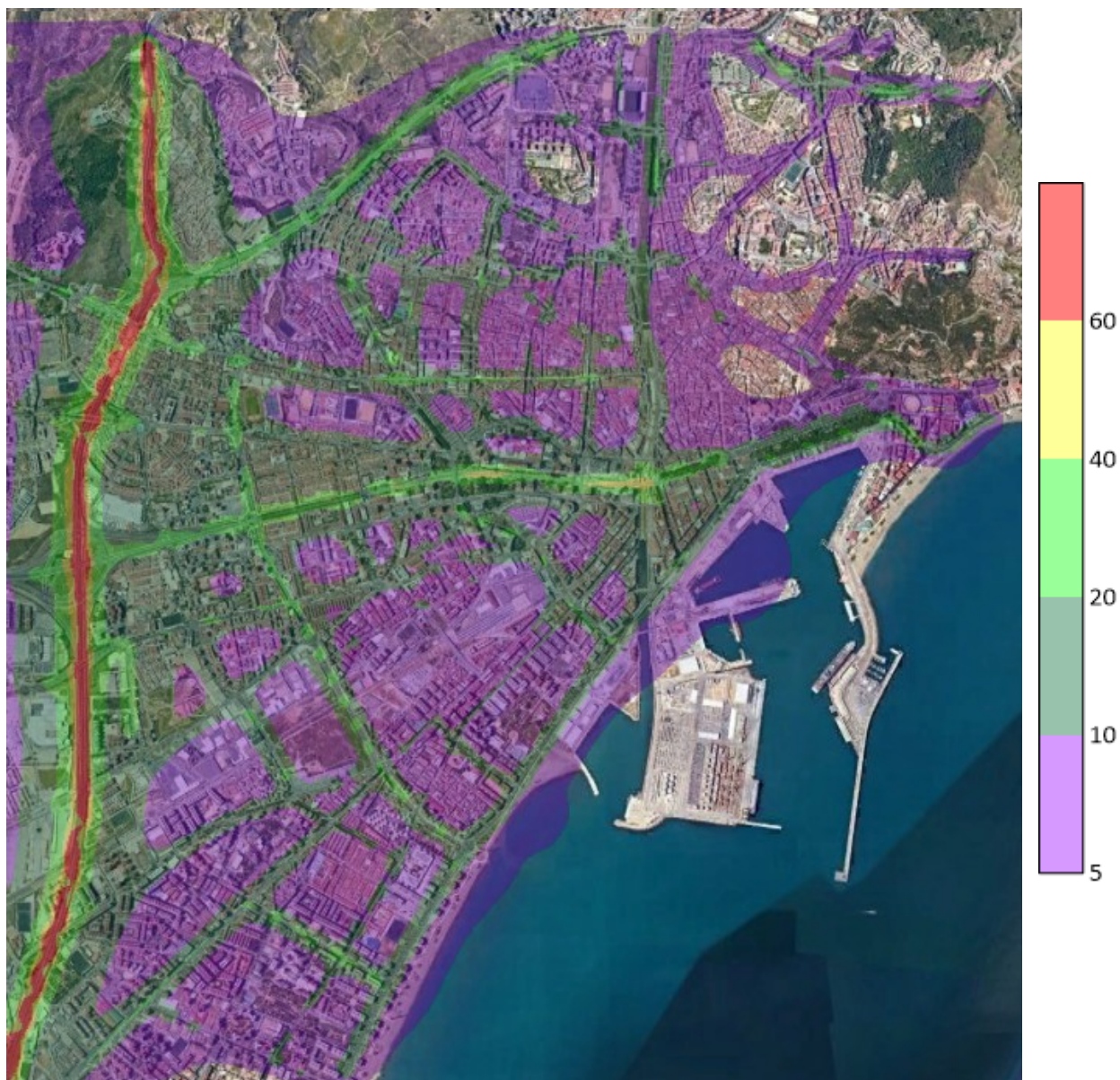
Figura AI.13. Contribución del tráfico a los niveles medios anuales de inmisión de \text{NO}_2 ( \mu\text{g}/\text{m}^3 )
