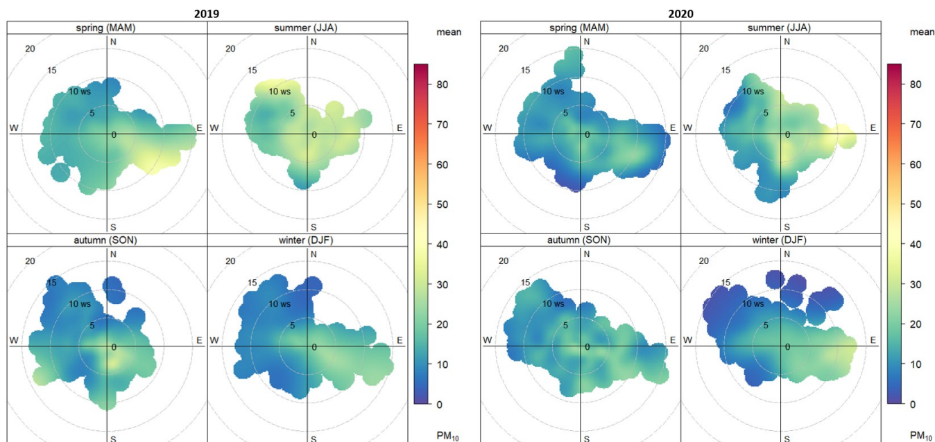
Figura 6.42. Relación entre los niveles horarios de PM_{10} y la velocidad y dirección del viento en 2019 y 2020. Estación El Atabal
