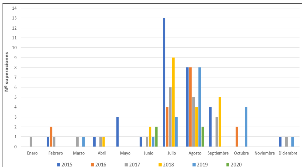
Figura 6.13. Número de superaciones por mes del valor límite diario de PM 10 en el periodo 2015-2020. Estación Marbella Arco
