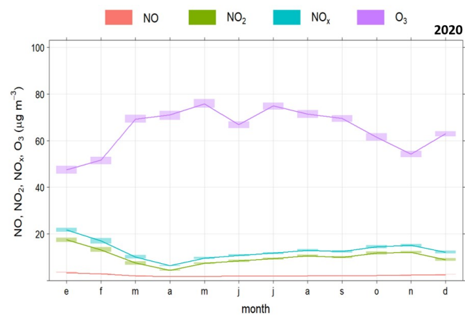
Figura 6.25. Medias mensuales de O 3 , NO x , NO 2 y NO en los años 2019 y 2020. Estación Campanillas
