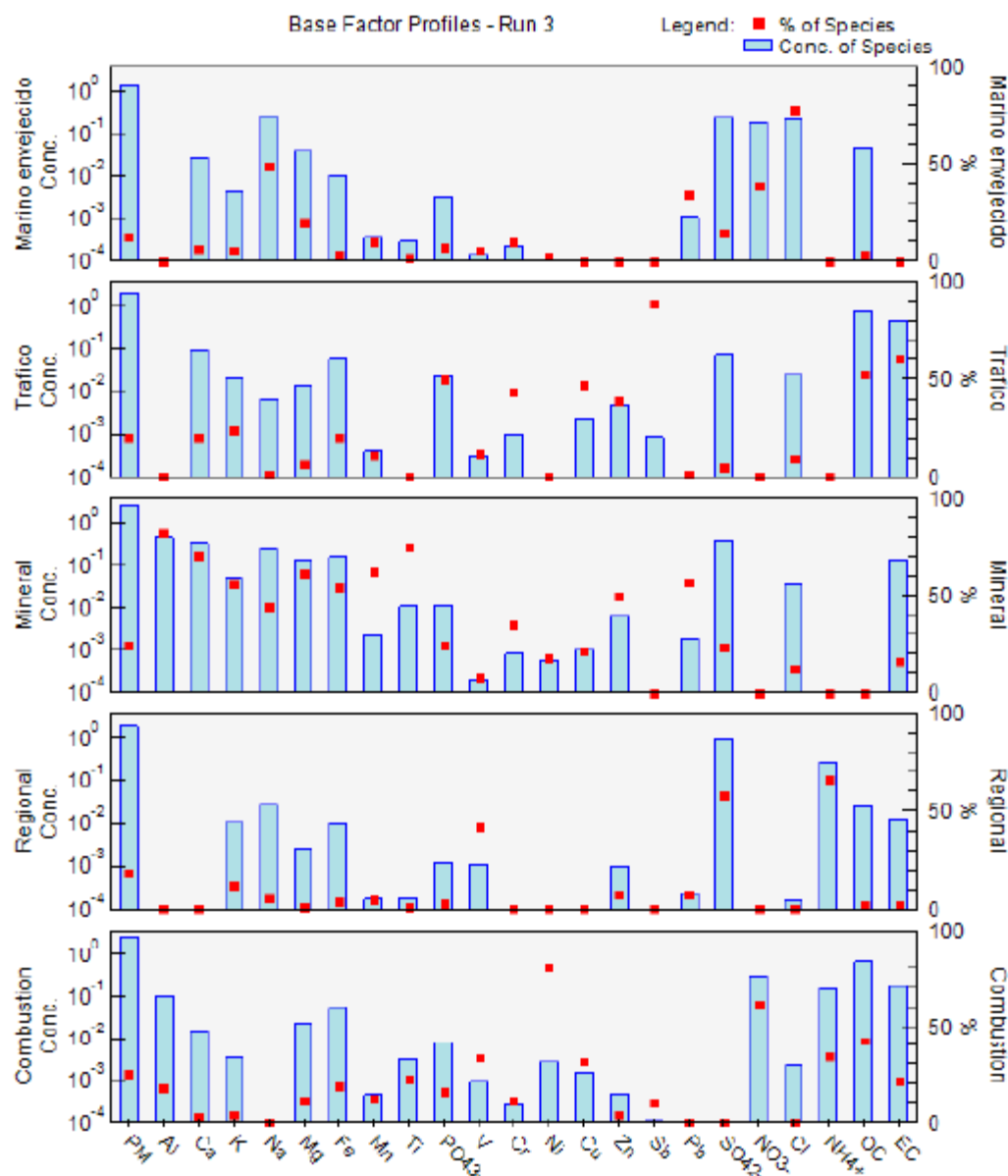
Figura 6.55. Perfil químico de las fuentes de PM_{2.5} (expresado como contribución de elementos mayores y traza en \mu g/m^3 ) determinadas en la estación de Marbella Arco en el año 2021
