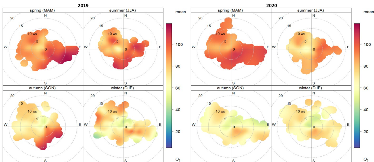
Figura 6.47. Relación entre los niveles horarios de O_3 y la velocidad y dirección del viento en 2019 y 2020. Estación El Atabal
