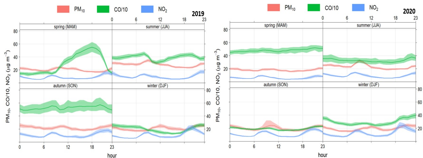
Figura 6.9. Patrón horario estacional para NO 2 , PM 10 y CO en 2019 y 2020. Estación Campanillas
