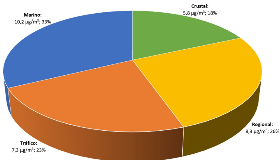
Figura 6.51. Contribución de fuentes en el periodo 2021 para \text{PM}_{10} en la estación de Marbella Arco
