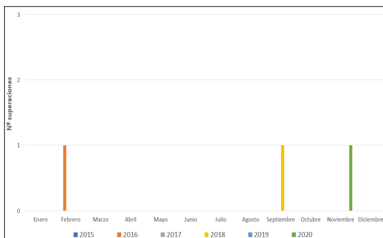
Figura 6.17. Número de superaciones por mes del valor límite diario de PM 10 en el periodo 2015-2020. Estación Campanillas
