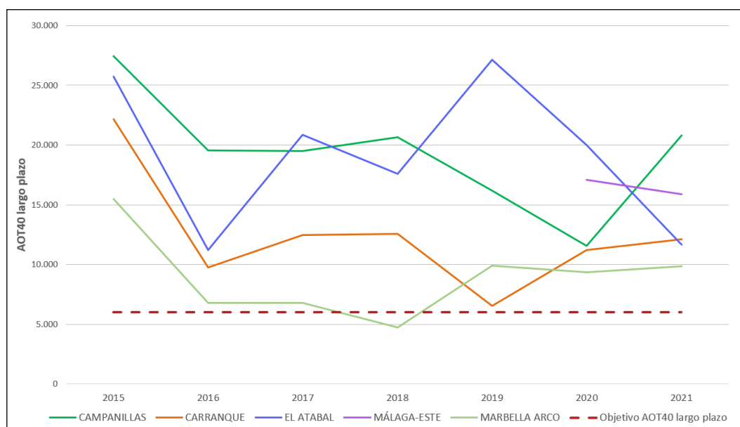
Figura 5.13. AOT40 ( \mu\text{g}/\text{m}^3 \cdot \text{h} ) a largo plazo para Málaga y Costa del Sol
