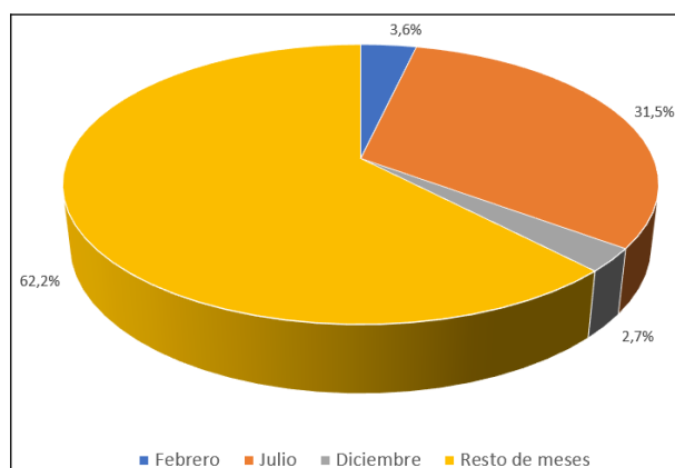
Figura 6.14. Distribución mensual de las superaciones del valor límite diario de PM 10 en el periodo 2015-2020. Estación Marbella Arco
