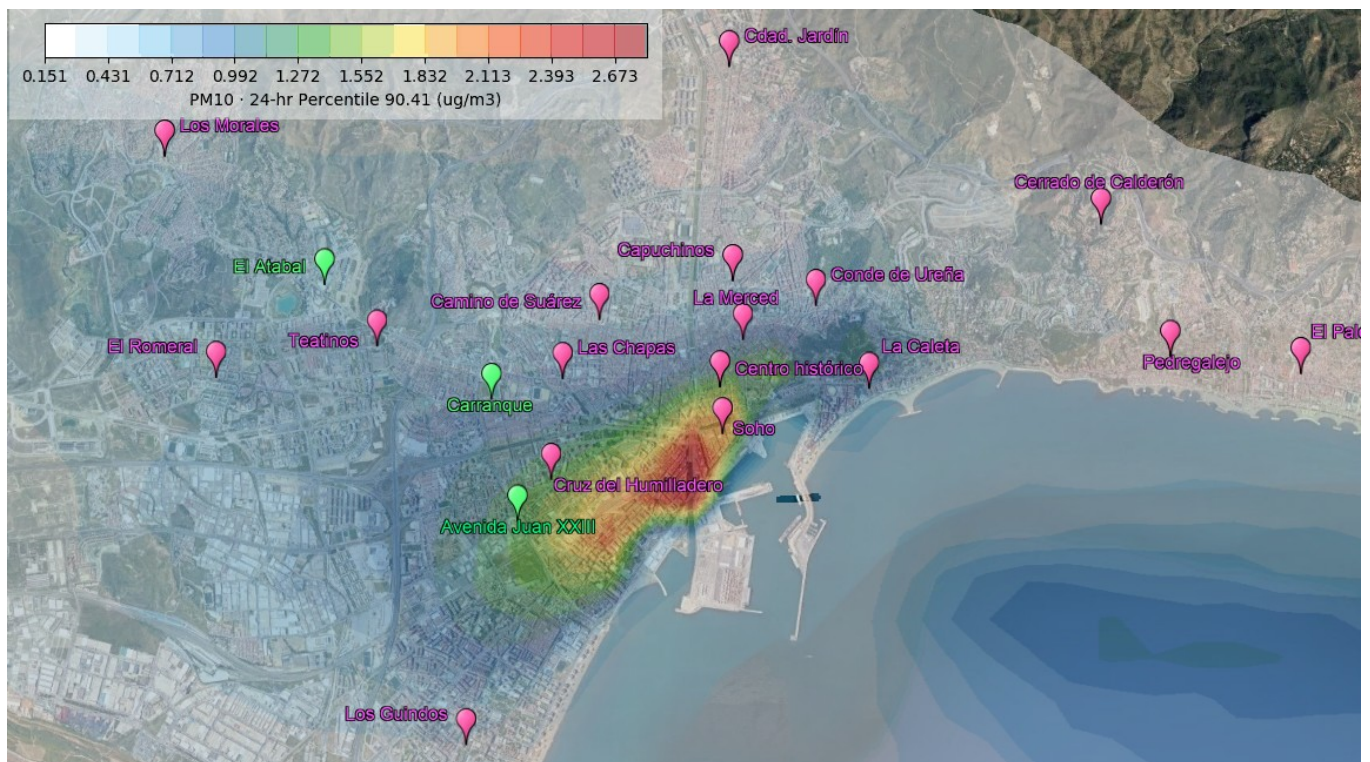
Figura AII.14. Contribución del tráfico marítimo al percentil 90,41 de los valores medios diarios de PM 10 . Escenario 3 (3 cruceros + 1 ferry)
