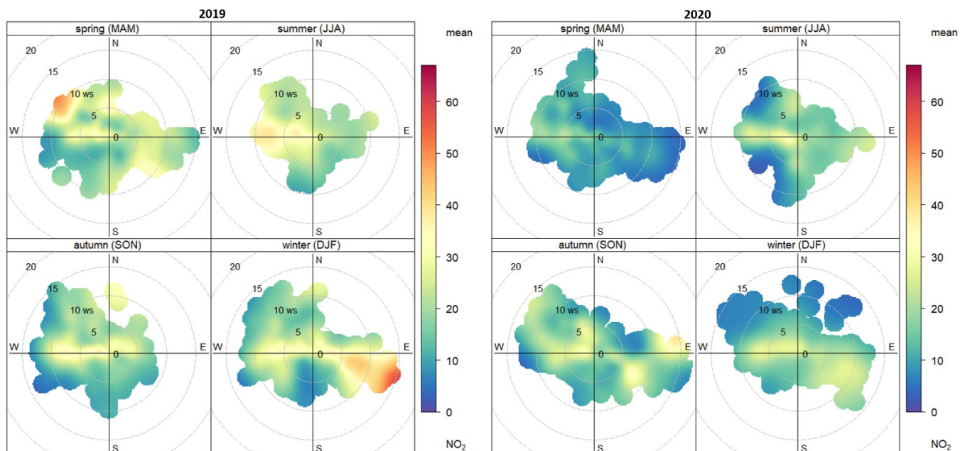
Figura 6.33. Relación entre los niveles horarios de \text{NO}_2 y la velocidad y dirección del viento en 2019 y 2020. Estación Marbella Arco
