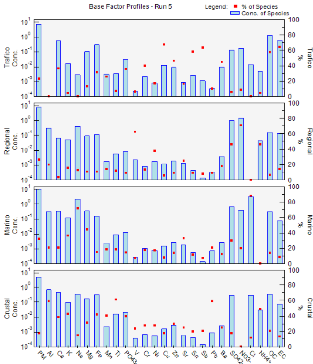
Figura 6.52. Perfil químico de las fuentes de PM 10 (expresado como contribución de elementos mayores y traza en µg/m 3 ) eterminadas en la estación de Marbella Arco en el año 2021
