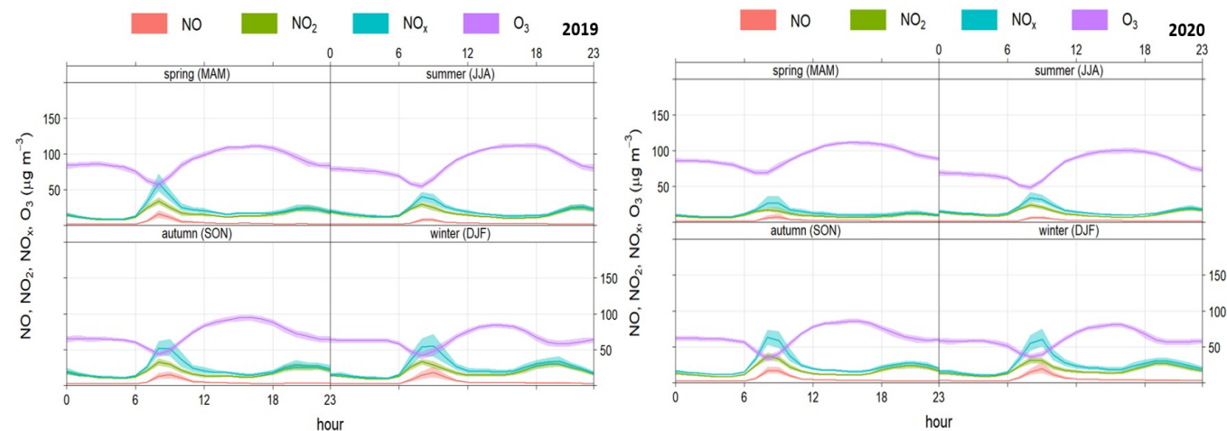
Figura 6.31. Patrón horario estacional para O 3 , NO x , NO 2 y NO en 2019 y 2020. Estación El Atabal
