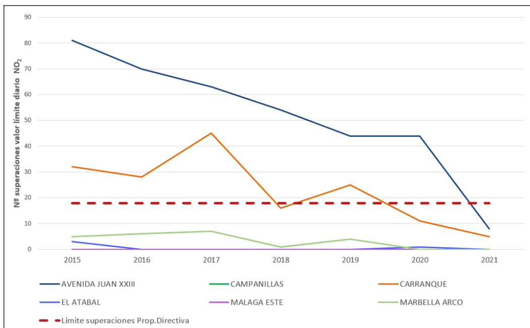
Figura 5.10. Número de superaciones del futuro valor límite diario de NO 2 (propuesta de directiva de calidad del aire) en Málaga y Costa del Sol
