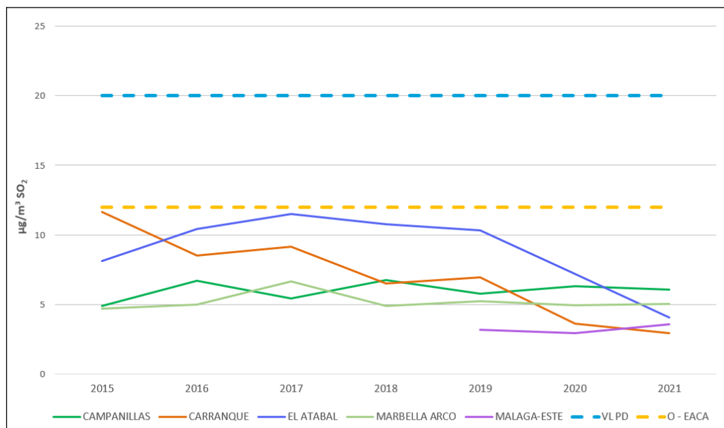
Figura 5.14. Promedio anual de SO 2 (µg/m 3 ) frente al futuro valor límite anual (propuesta de directiva de calidad del aire) en Málaga y Costa del Sol
