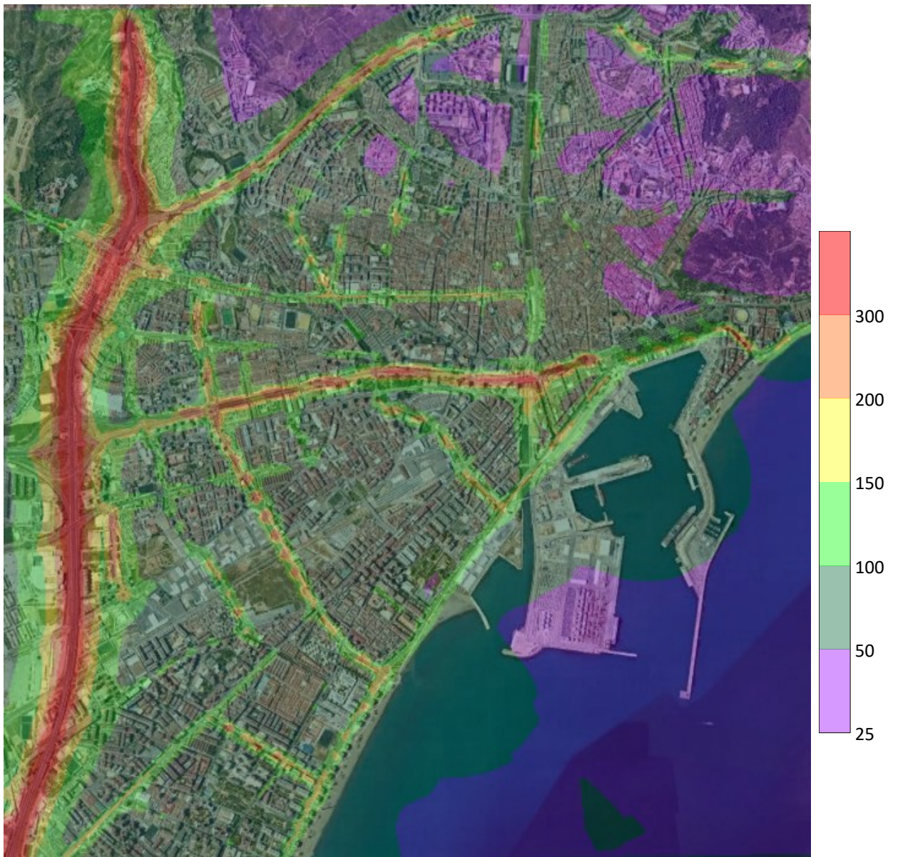
Figura AI.14. Contribución del tráfico al percentil 99,79 de los niveles medios horarios de inmisión de NO 2 (µg/m 3 )
