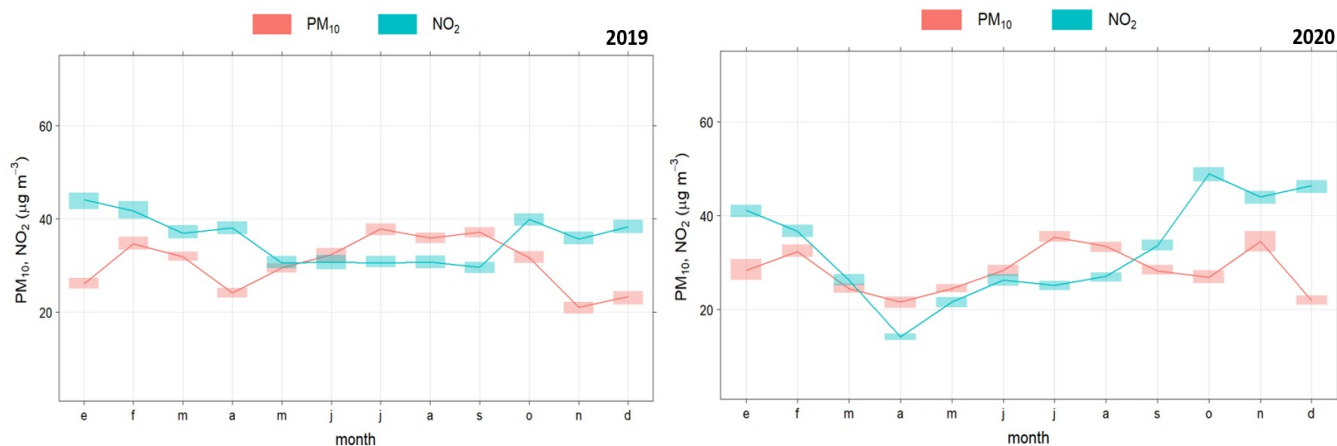
Figura 6.5. Medias mensuales de NO 2 y PM 10 en los años 2019 y 2020. Estación Avda. Juan XXIII
