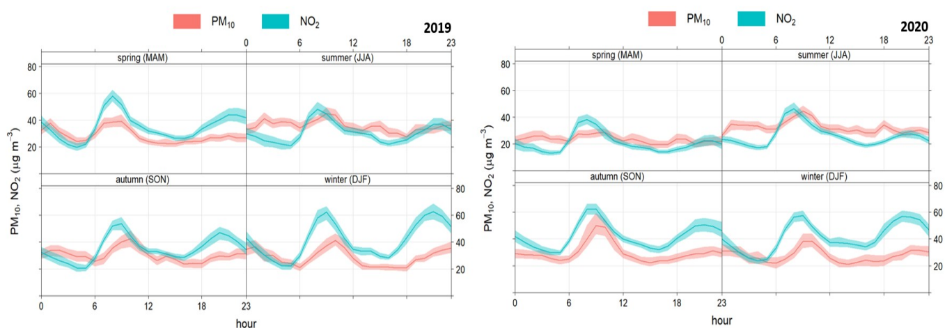
Figura 6.11. Patrón horario estacional para NO 2 y PM 10 en 2019 y 2020. Estación Avda. Juan XXIII
