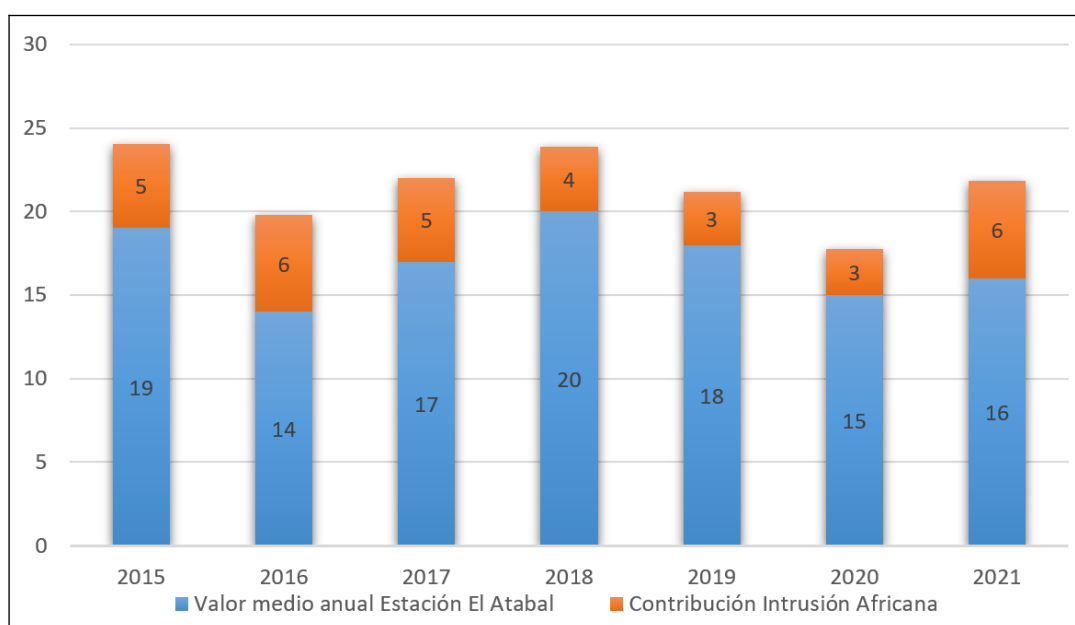
Figura 5.39. Contribución de la carga neta de polvo africano al valor medio anual. Estación El Atabal 10
