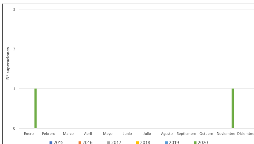
Figura 6.21. Número de superaciones por mes del valor límite diario de PM 10 en el periodo 2015-2020. Estación Avda. Juan XXIII
