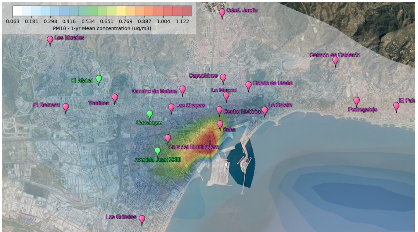
Figura AII.13. Contribución del tráfico marítimo a la media anual de los valores de PM 10 . Escenario 3 (3 cruceros + 1 ferry)
