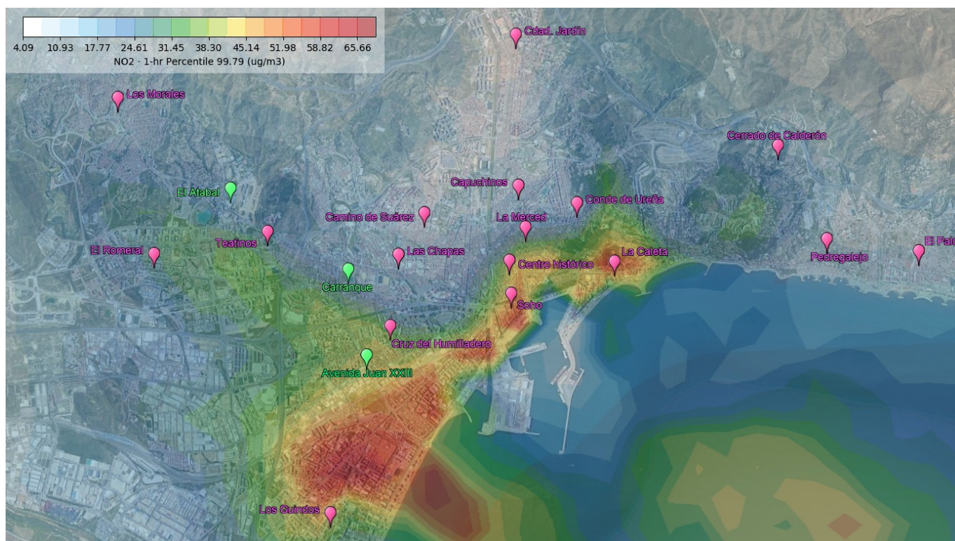
Figura All.4. Contribución del tráfico marítimo al percentil 99,79 de los valores medios horarios de NO 2 . Escenario 1 (1 crucero + 1 ferry)
