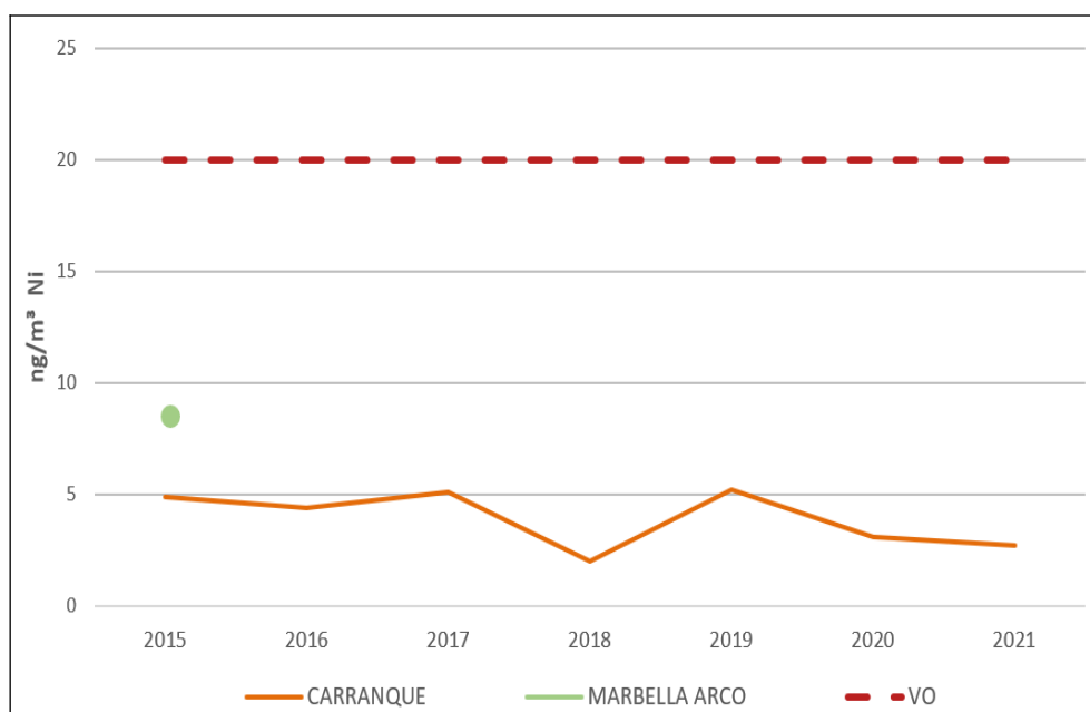
Figura 5.19. Medias anuales de Ni (ng/m³) en Málaga y Costa del Sol
