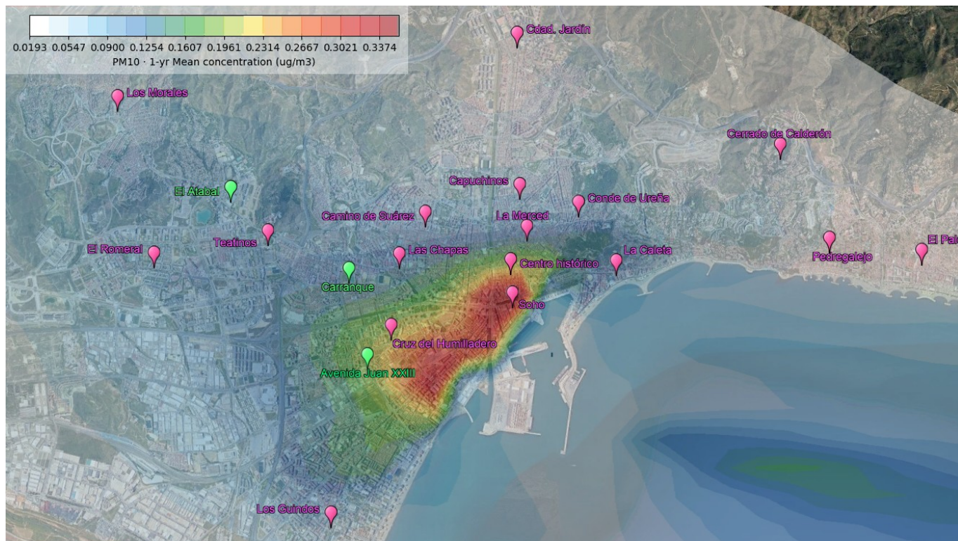
Figura AII.5. Contribución del tráfico marítimo a la media anual de los valores de PM 10 . Escenario 1 (1 crucero + 1 ferry)
