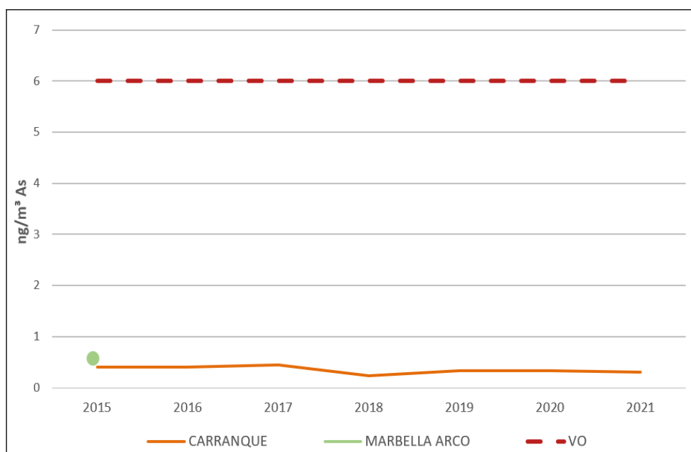
Figura 5.17. Medias anuales de As (ng/m 3 ) en Málaga y Costa del Sol
