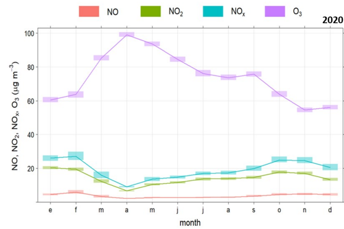
Figura 6.26. Medias mensuales de O 3 , NO x , NO 2 y NO en los años 2019 y 2020. Estación El Atabal
