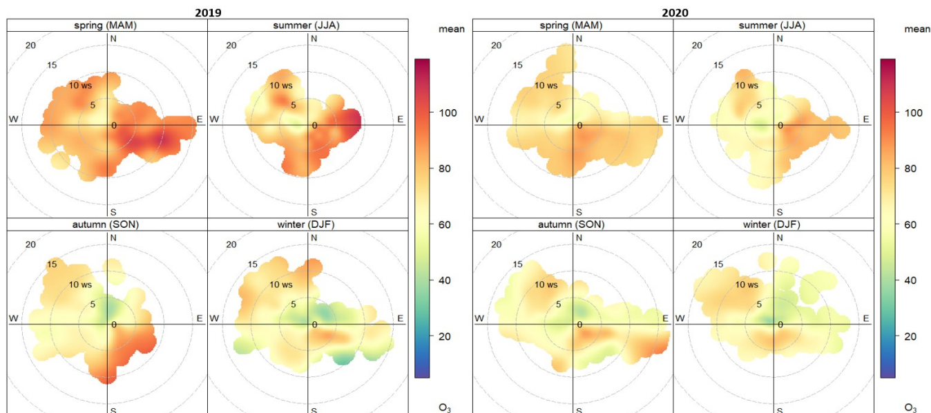
Figura 6.46. Relación entre los niveles horarios de O_3 y la velocidad y dirección del viento en 2019 y 2020. Estación Campanillas
