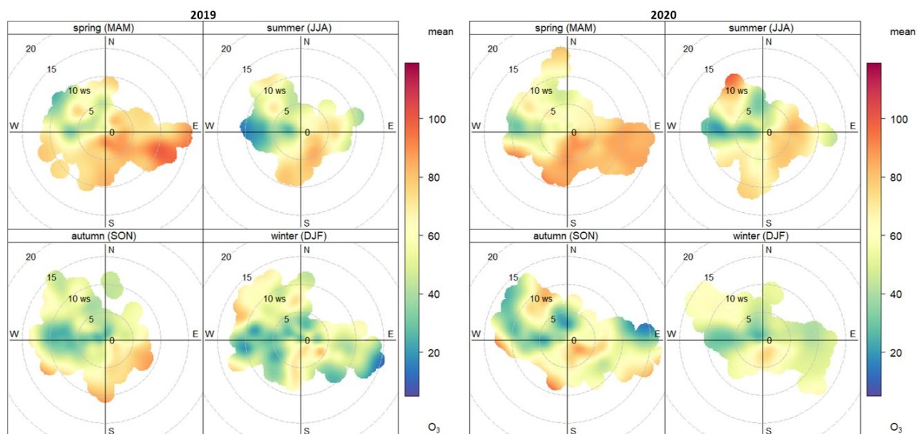
Figura 6.44. Relación entre los niveles horarios de O_3 y la velocidad y dirección del viento en 2019 y 2020. Estación Marbella Arco
