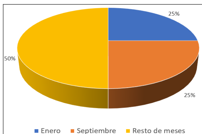
Figura 6.20. Distribución mensual de las superaciones del valor límite diario de PM 10 en el periodo 2015-2020. Estación El Atabal
