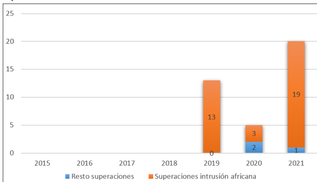
Figura 5.30. Origen y cuantificación del número de superaciones diarias de PM_{10} ( \mu g/m^3 ) en la estación Avda. Juan XXIII 2
