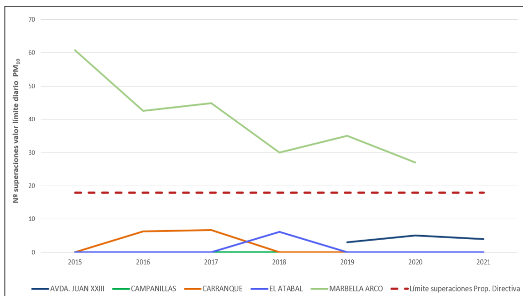
Figura 5.5. Número de superaciones del futuro valor límite diario de PM_{10} (propuesta de directiva de calidad del aire) en Málaga y Costa del Sol
