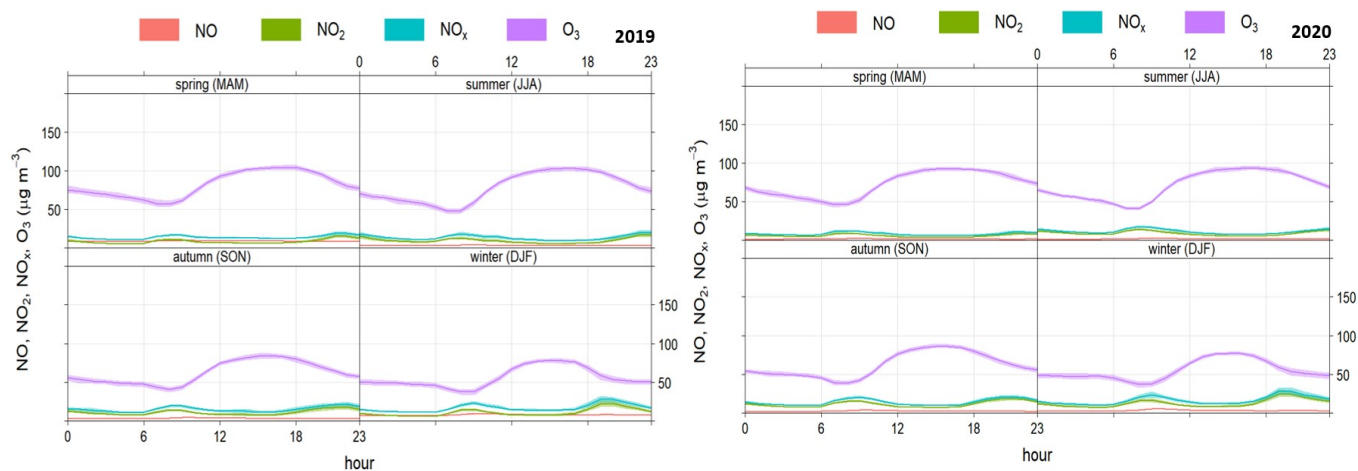
Figura 6.30. Patrón horario estacional para O 3 , NO x , NO 2 y NO en 2019 y 2020. Estación Campanillas
