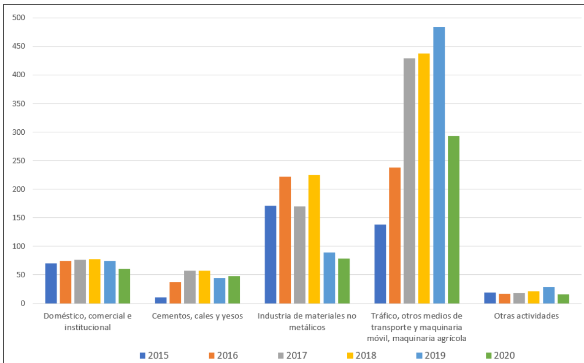
Figura 6.64. Evolución de las emisiones inventariadas de SO 2 (t/año)
