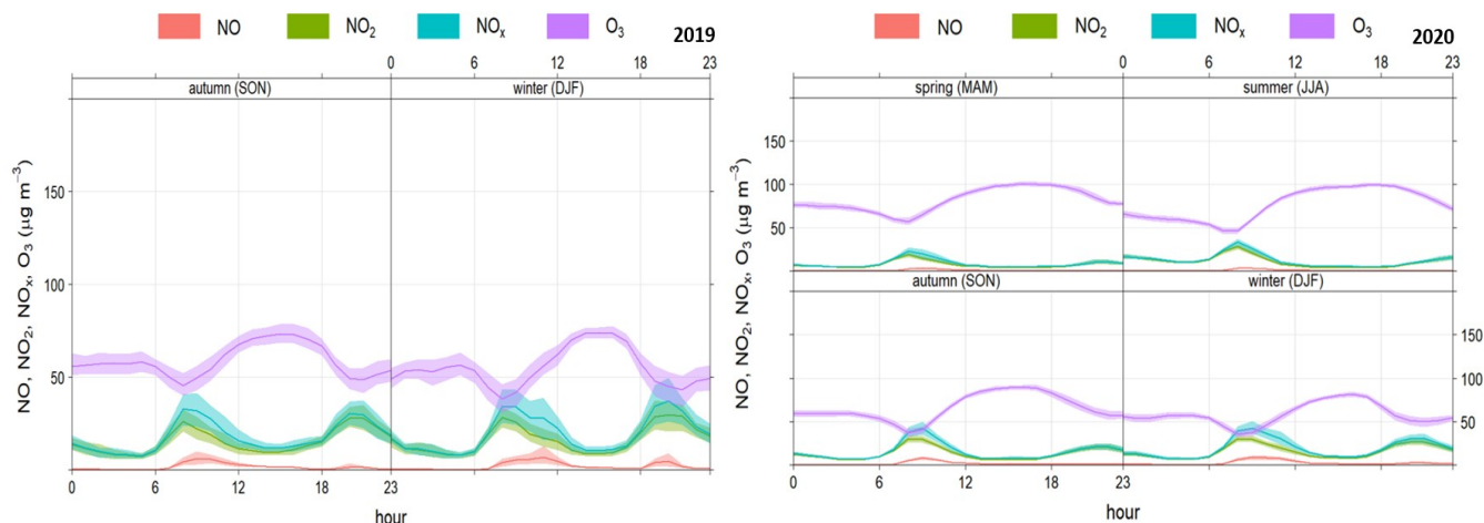
Figura 6.32. Patrón horario estacional para O 3 , NO x , NO 2 y NO en 2019 y 2020. Estación Málaga Este
