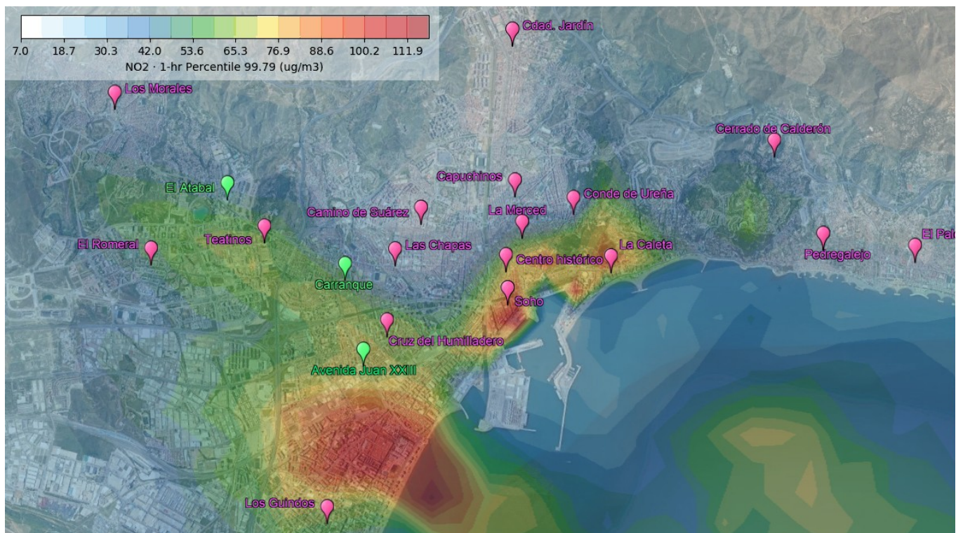
Figura All.8. Contribución del tráfico marítimo al percentil 99,79 de los valores medios horarios de NO 2 . Escenario 2 (2 cruceros + 1 ferry)
