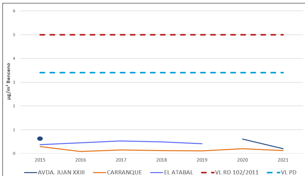
Figura 5.15. Valor límite anual de benceno ( \mu\text{g}/\text{m}^3 ) para la protección de la salud en Málaga y Costa del Sol
