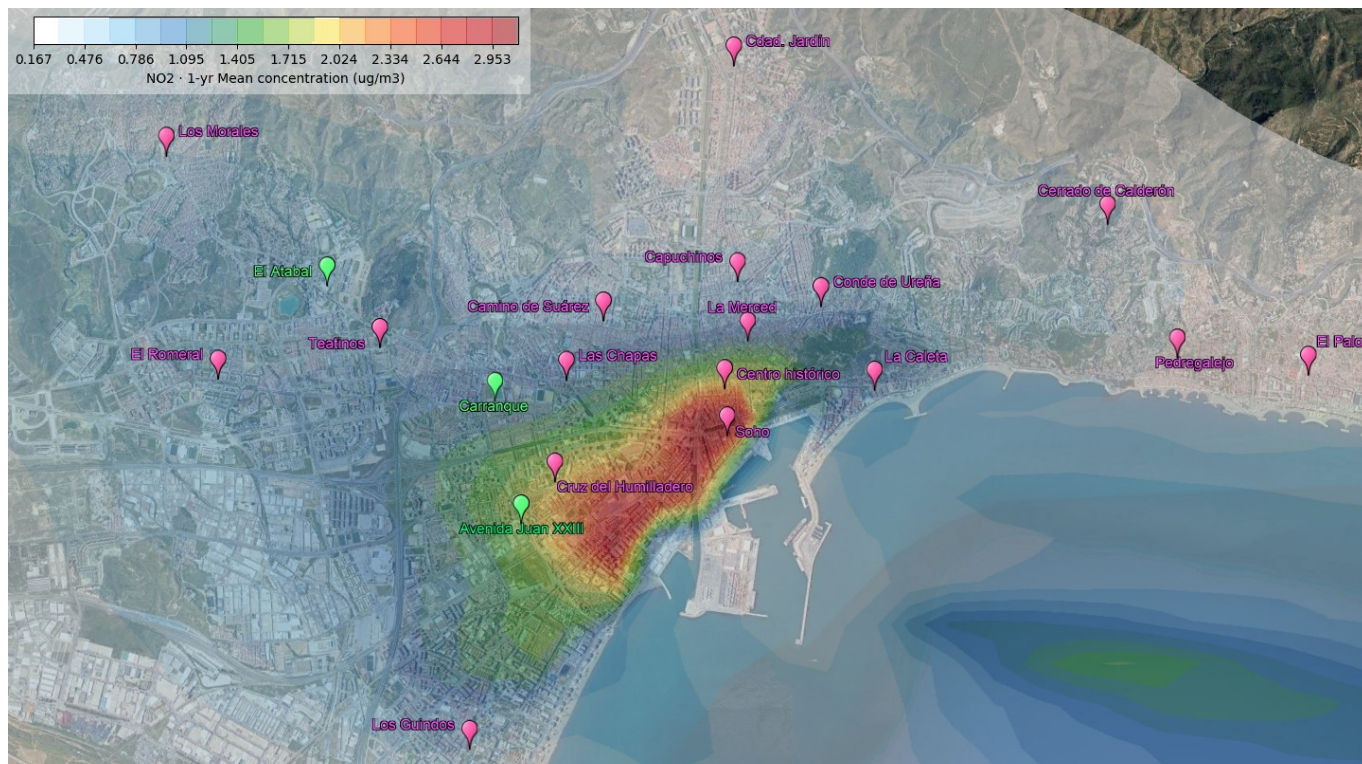
Figura All.3. Contribución del tráfico marítimo a la media anual de los valores de NO 2 . Escenario 1 (1 crucero + 1 ferry)
