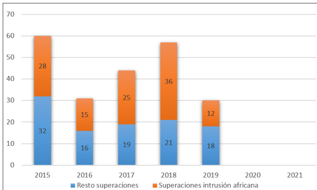
Figura 5.34. Origen y cuantificación del número de superaciones diarias de PM 10 (µg/m 3 ) en la estación Marbella Arco 6
