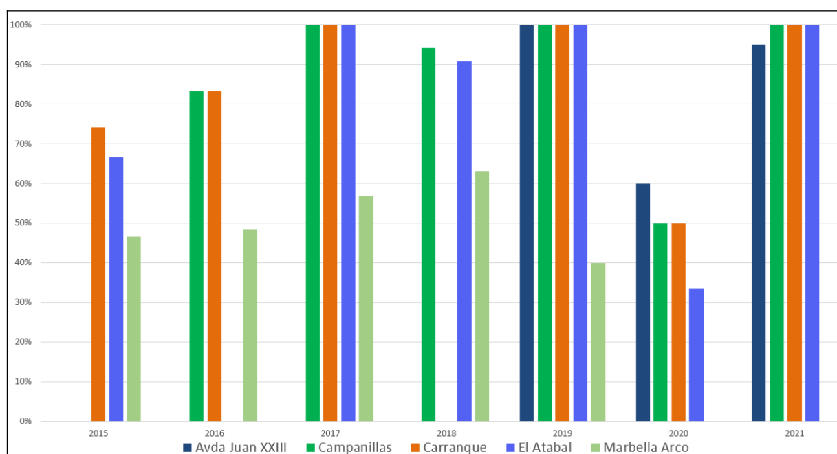
Figura 5.35. Porcentaje medio de la contribución de los eventos de intrusiones de masas de aire norteafricano al número de superaciones del valor límite diario en las 5 estaciones
