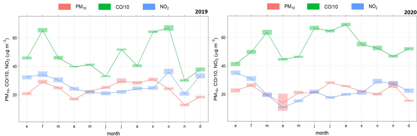
Figura 6.2. Medias mensuales de NO_2 , PM_{10} y CO en los años 2019 y 2020. Estación Carranque
