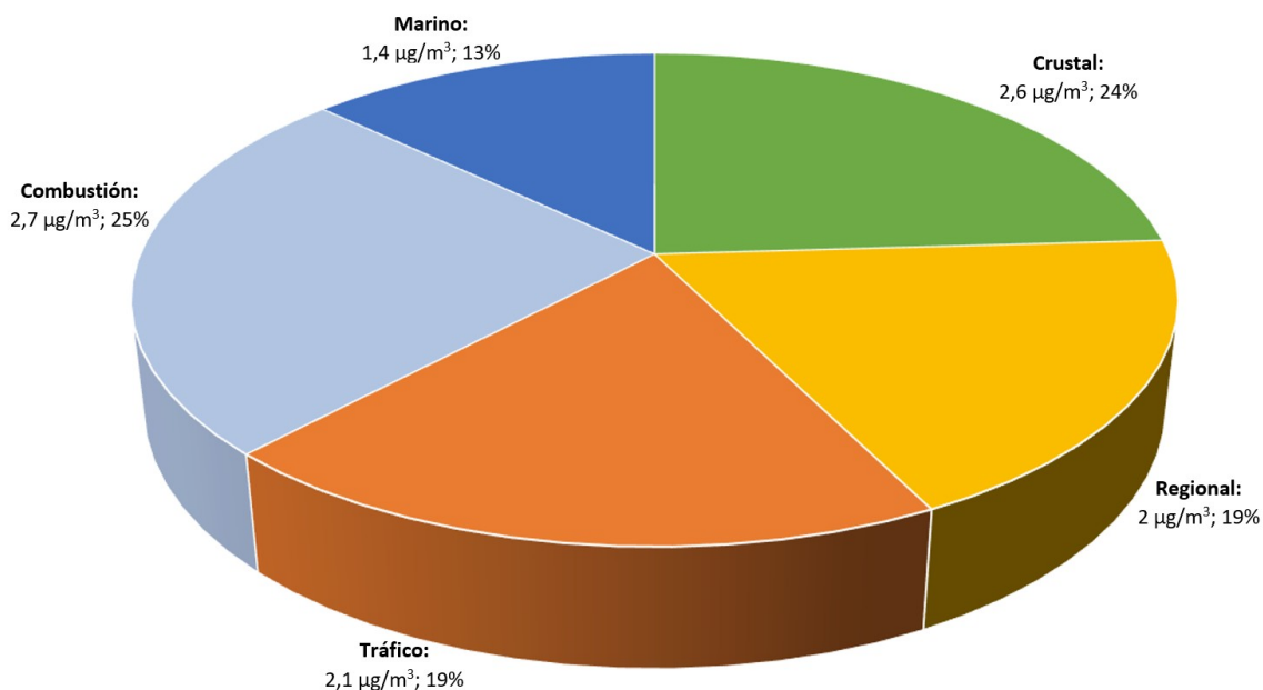
Figura 6.54. Contribución de fuentes en el periodo 2021 para PM_{2,5} en la estación de Marbella Arco
