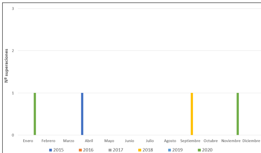
Figura 6.19. Número de superaciones por mes del valor límite diario de PM 10 en el periodo 2015-2020. Estación El Atabal
