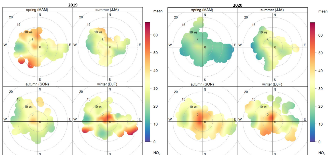
Figura 6.37. Relación entre los niveles horarios de \text{NO}_2 y la velocidad y dirección del viento en 2019 y 2020. Estación Avda. Juan XXIII
