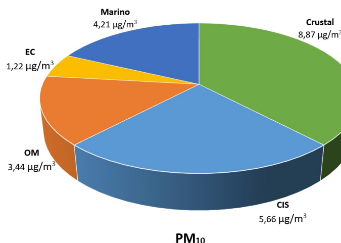
Figura 6.50. Diagrama de agrupación de compuestos y elementos principales en PM 10 en la estación de Carranque
