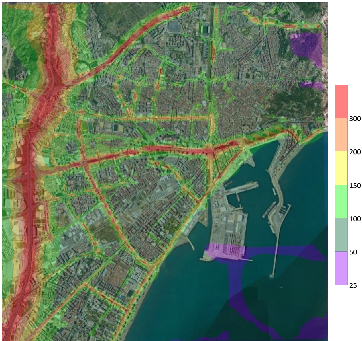
Figura AI.15. Contribución del tráfico al valor máximo horario de inmisión de NO 2 (µg/m 3 )
