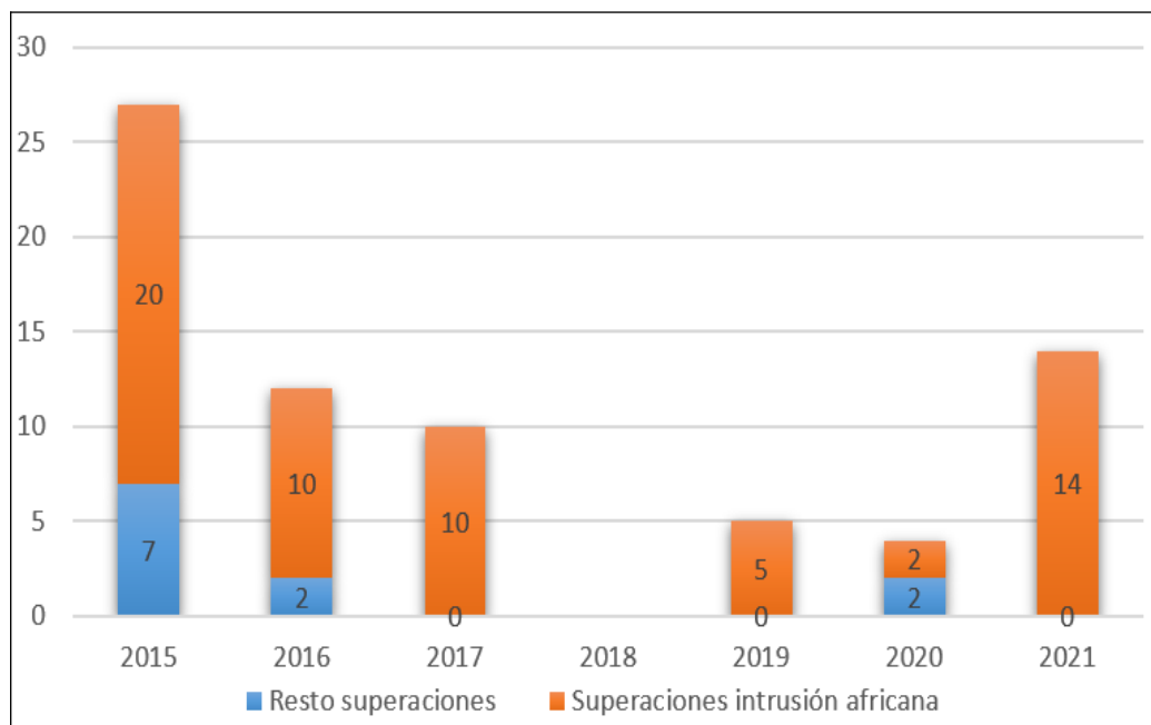
Figura 5.32. Origen y cuantificación del número de superaciones diarias de PM 10 (µg/m 3 ) en la estación Carranque 4
