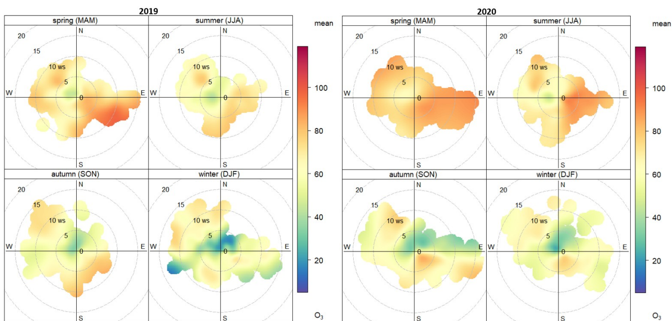
Figura 6.45. Relación entre los niveles horarios de O_3 y la velocidad y dirección del viento en 2019 y 2020. Estación Carranque
