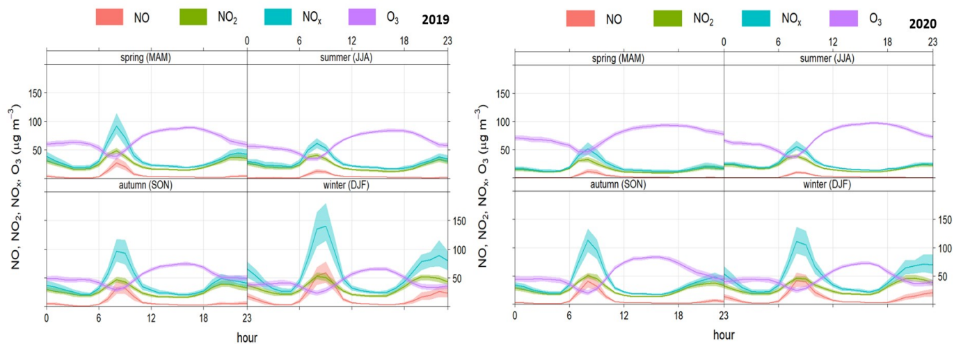
Figura 6.29. Patrón horario estacional para O 3 , NO x , NO 2 y NO en 2019 y 2020. Estación Carranque
