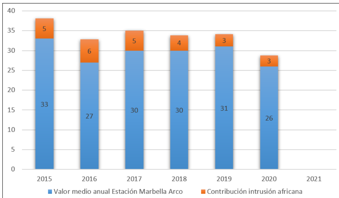
Figura 5.40. Contribución de la carga neta de polvo africano al valor medio anual. Estación Marbella Arco 11
