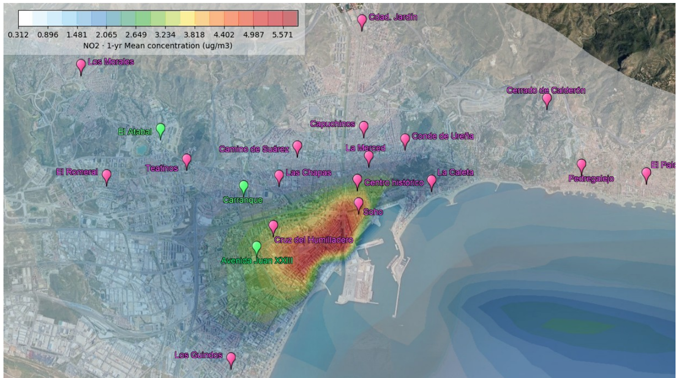
Figura All.7. Contribución del tráfico marítimo a la media anual de los valores de NO 2 . Escenario 2 (2 cruceros + 1 ferry)
