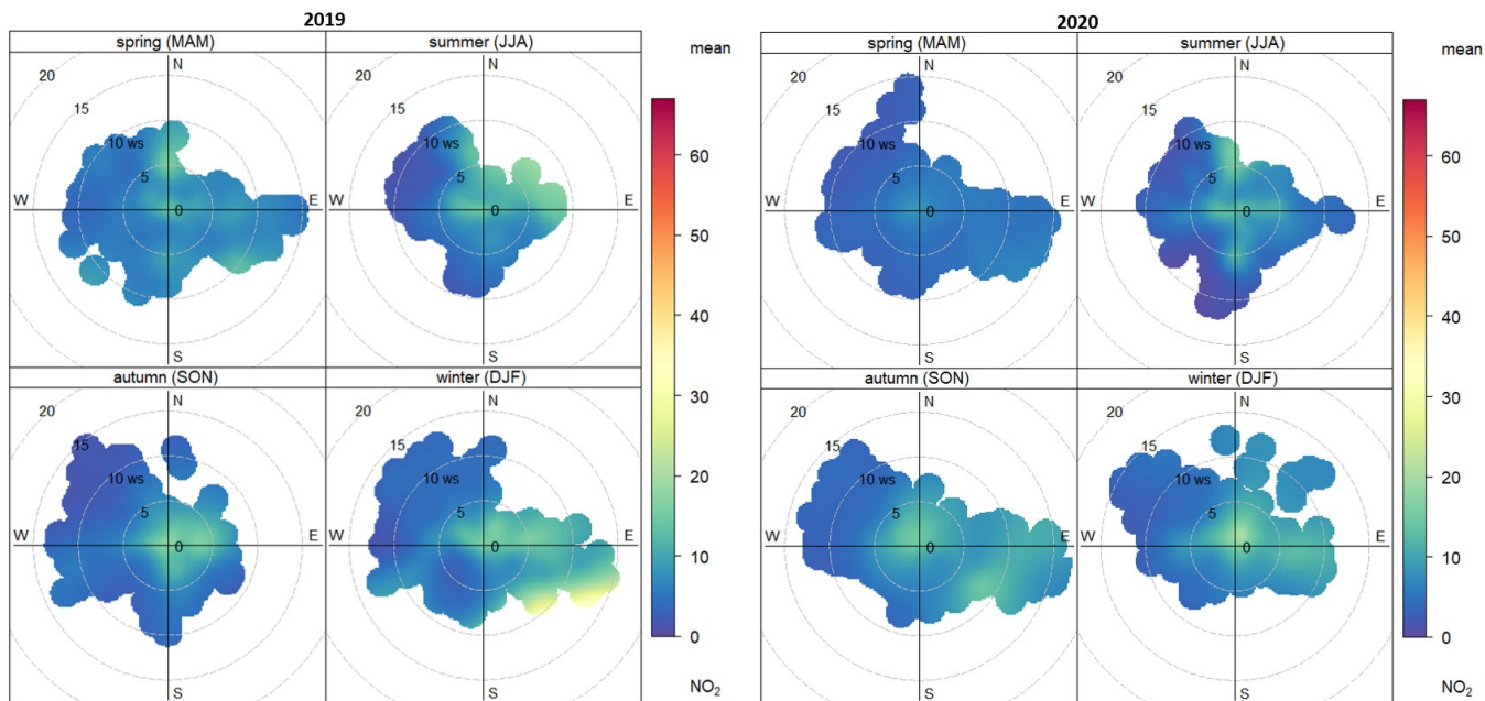
Figura 6.35. Relación entre los niveles horarios de \text{NO}_2 y la velocidad y dirección del viento en 2019 y 2020. Estación Campanillas
