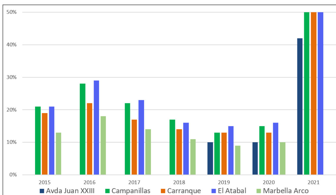
Figura 5.41. Porcentaje medio de la contribución de los eventos de intrusiones de masas de aire africano al valor medio anual en las 5 estaciones
