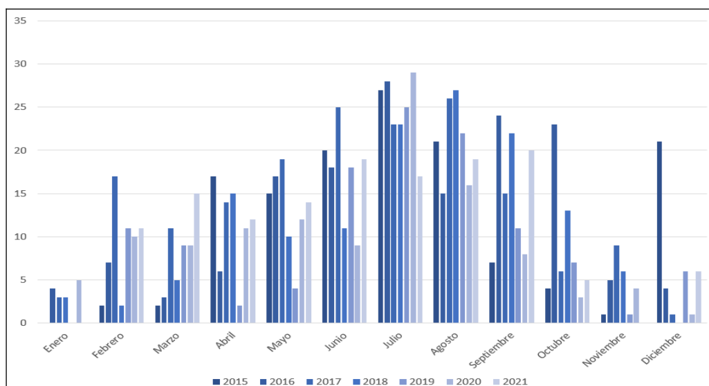
Figura 5.29. Días con intrusión de aire africano por mes. Periodo 2015-2021
