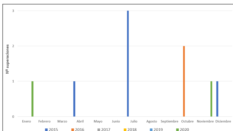
Figura 6.15. Número de superaciones por mes del valor límite diario de PM 10 en el periodo 2015-2020. Estación Carranque
