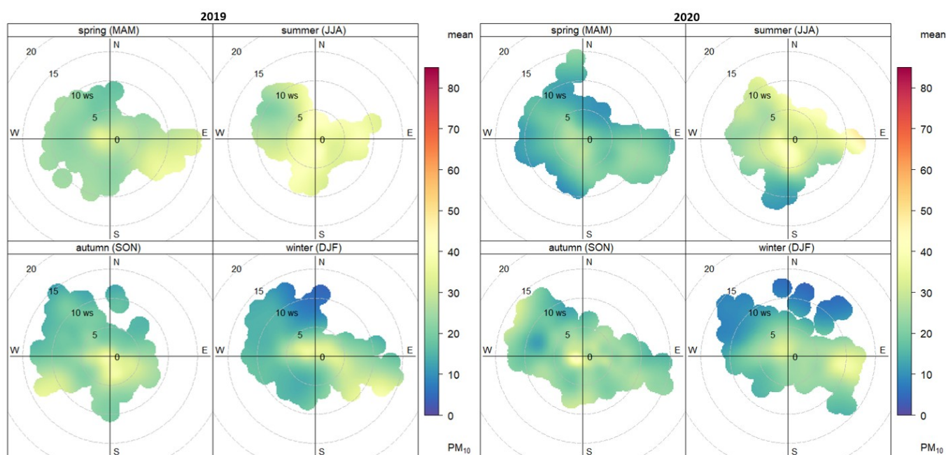
Figura 6.43. Relación entre los niveles horarios de PM_{10} y la velocidad y dirección del viento en 2019 y 2020. Estación Avda. Juan XXIII
