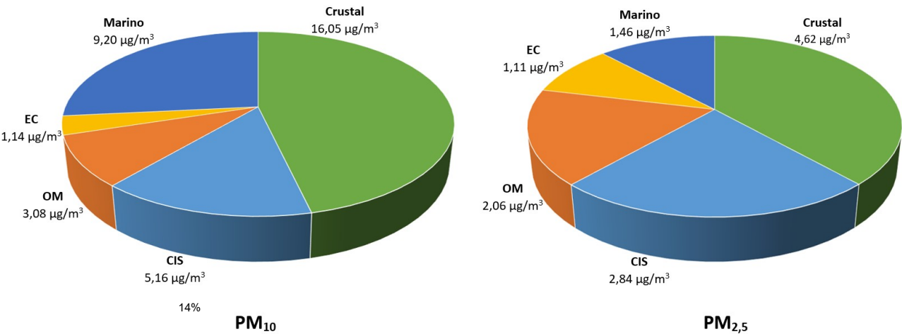
Figura 6.49. Diagrama de agrupación de compuestos principales en PM 10 y PM 2,5 en la estación de Marbella Arco
