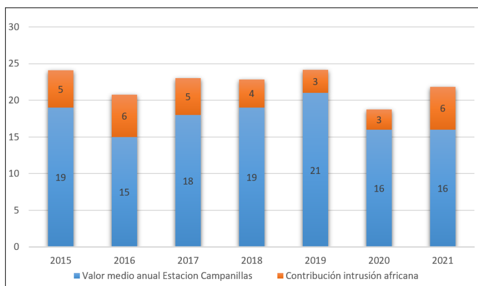
Figura 5.37. Contribución de la carga neta de polvo africano al valor medio anual. Estación Campanillas 8
