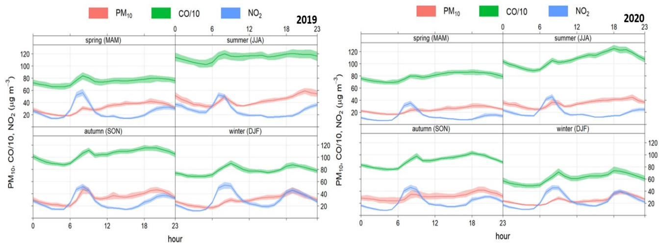
Figura 6.7. Patrón horario estacional para NO 2 , PM 10 y CO en 2019 y 2020. Estación Marbella Arco
