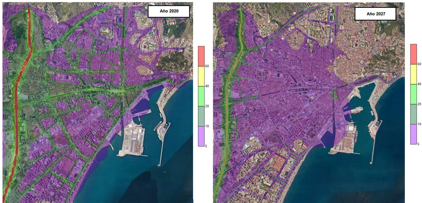
Figura AI.17. Contribución del tráfico a los niveles medios anuales de inmisión de \text{NO}_2 (Año 2020 vs. Año 2027) ( \mu\text{g}/\text{m}^3 )
