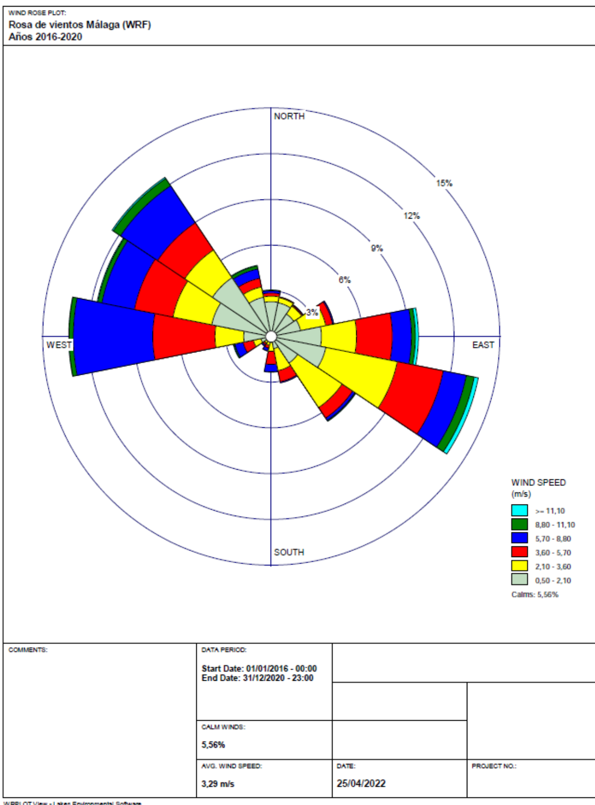
Figura AI.8. Rosa de vientos WRF periodo 2016-2020
