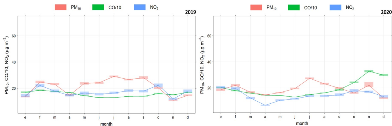
Figura 6.4. Medias mensuales de NO_2 , PM_{10} y CO en los años 2019 y 2020. Estación El Atabal
