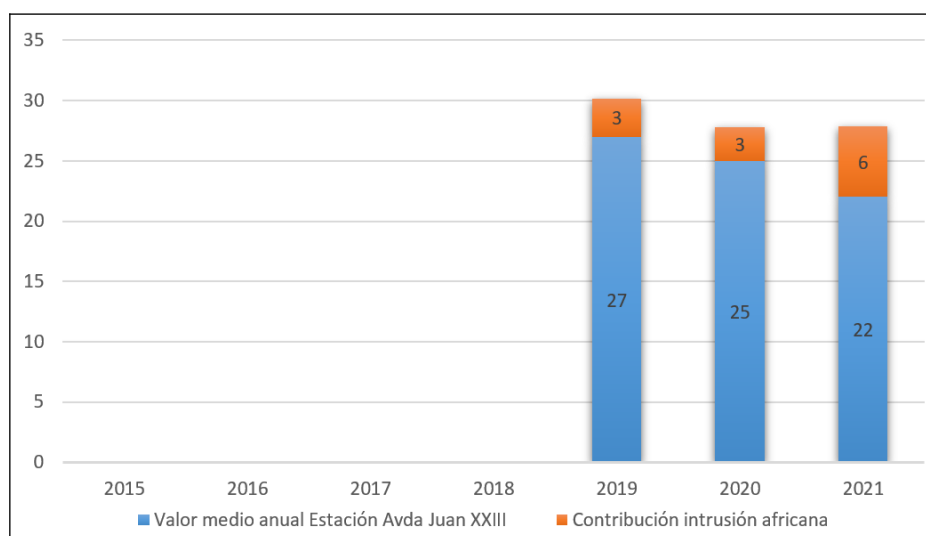
Figura 5.36. Contribución de la carga neta de polvo africano al valor medio anual. Estación Avda. Juan XXIII 7
