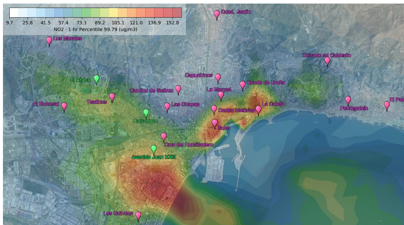
Figura AII.12. Contribución del tráfico marítimo al percentil 99,79 de los valores medios horarios de \text{NO}_2 . Escenario 3 (3 cruceros + 1 ferry)
