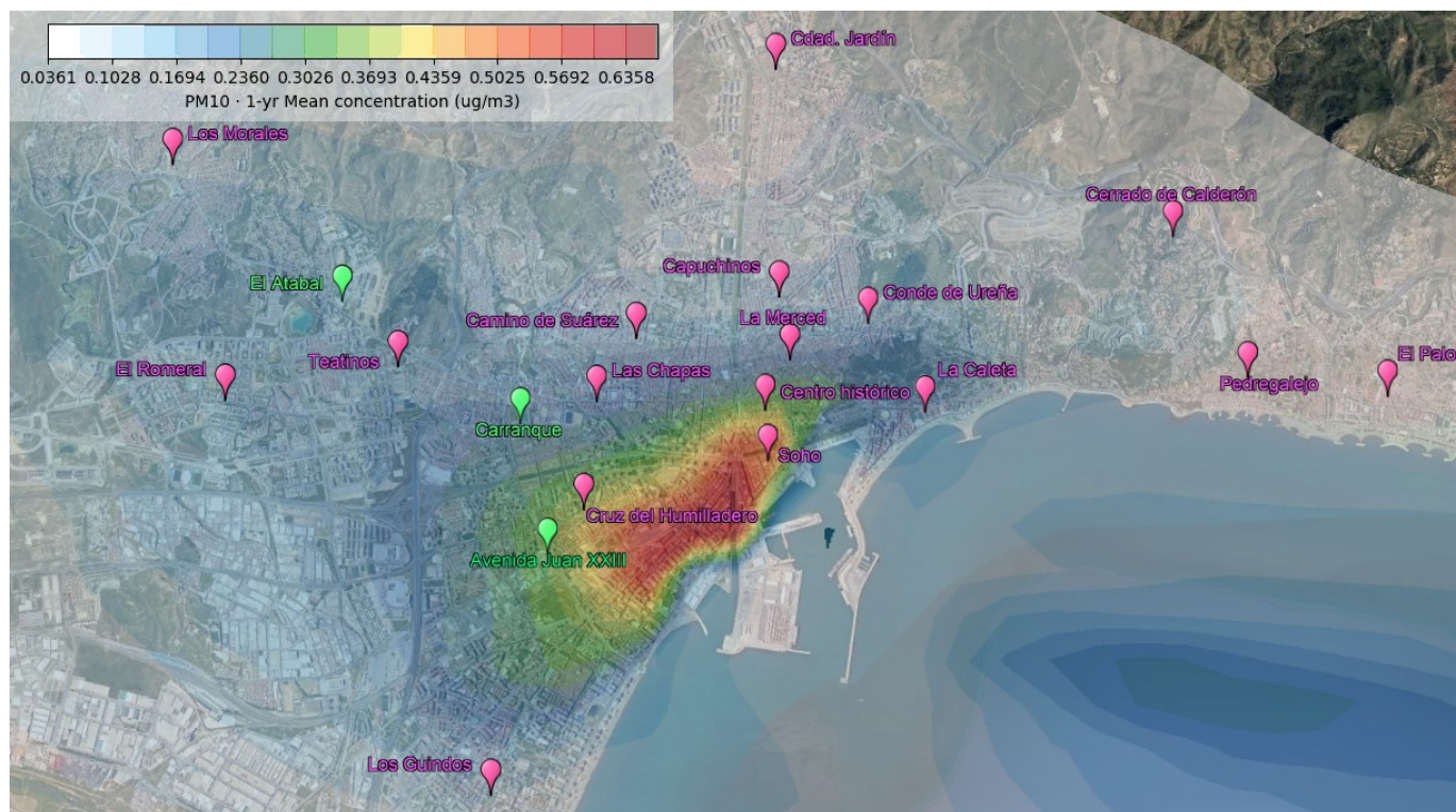
Figura AII.9. Contribución del tráfico marítimo a la media anual de los valores de PM 10 . Escenario 2 (2 cruceros + 1 ferry)
