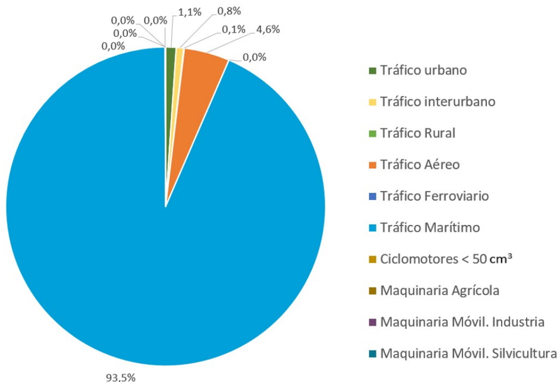
Figura 6.65. Contribución porcentual de distintas actividades a las emisiones de SO 2 en el sector tráfico en 2020
