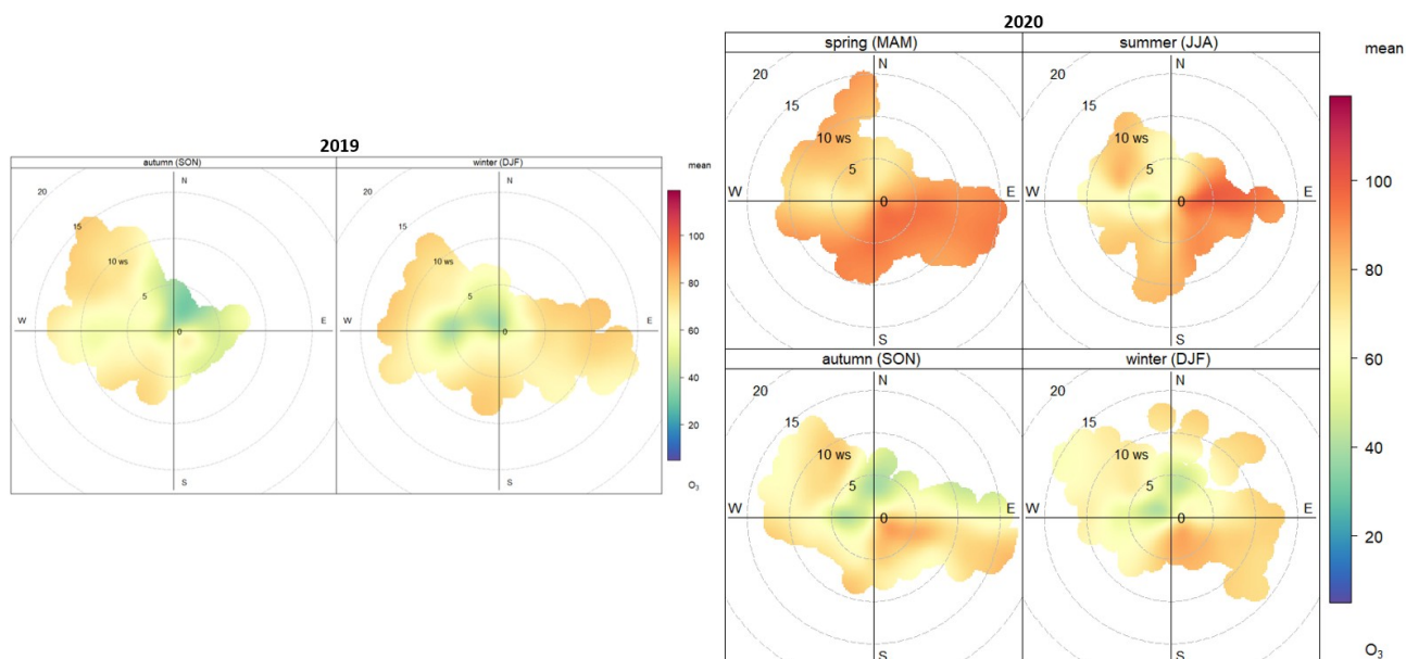
Figura 6.48. Relación entre los niveles horarios de O_3 y la velocidad y dirección del viento en 2019 y 2020. Estación Málaga Este
