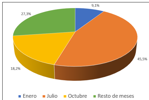
Figura 6.16. Distribución mensual de las superaciones del valor límite diario de PM 10 en el periodo 2015-2020. Estación Carranque
