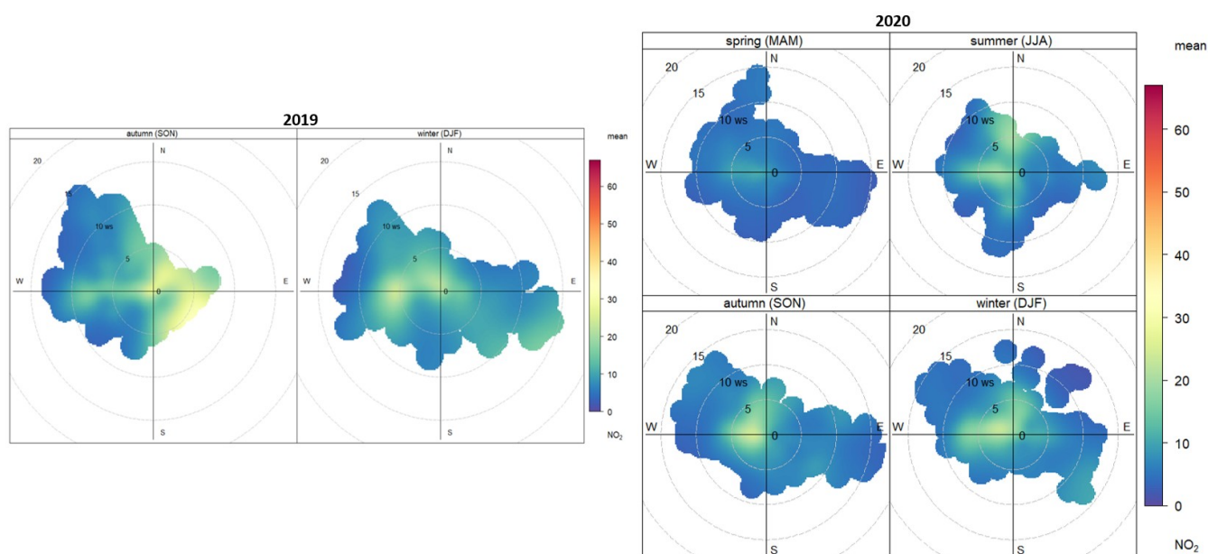
Figura 6.38. Relación entre los niveles horarios de \text{NO}_2 y la velocidad y dirección del viento en 2019 y 2020. Estación Málaga-Este
