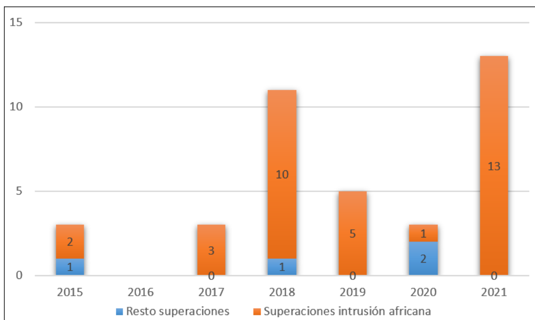
Figura 5.33. Origen y cuantificación del número de superaciones diarias de PM 10 (µg/m 3 ) en la estación El Atabal 5
