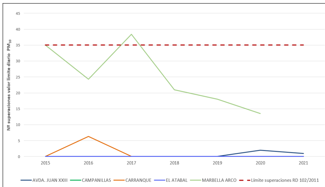
Figura 5.4. Número de superaciones del valor límite diario de PM_{10} en Málaga y Costa del Sol
