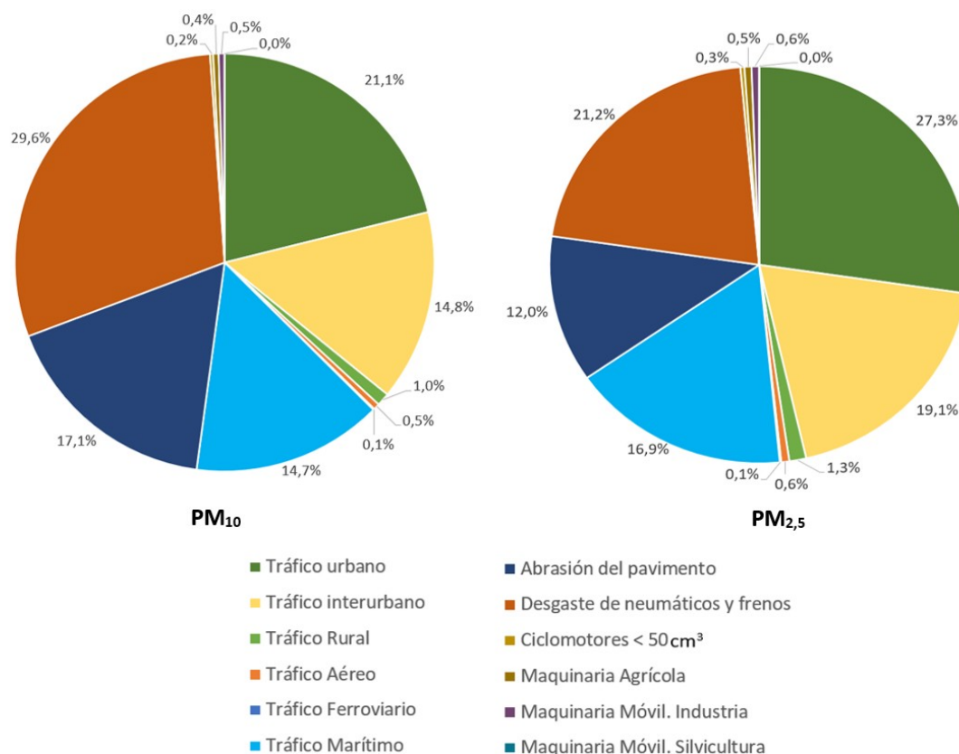
Figura 6.63. Contribución porcentual de distintas actividades a las emisiones de PM_{10} y PM_{2,5} en el sector tráfico en 2020
