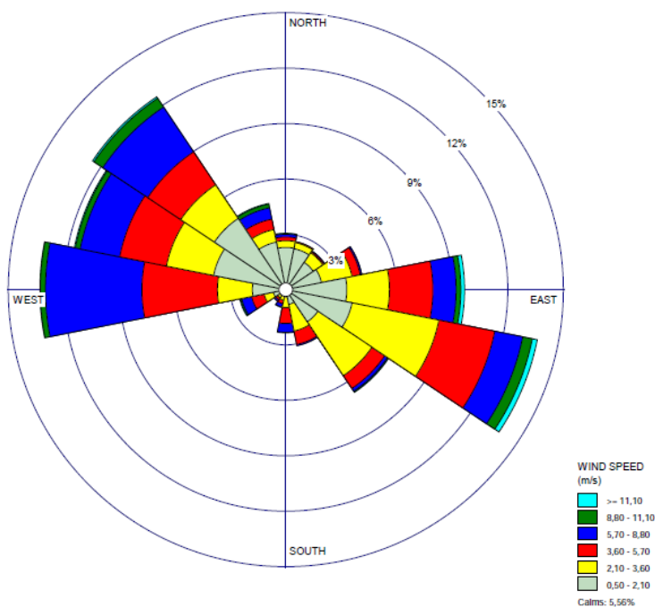
Figura 4.7. Rosa de los vientos (modelo WRF)
