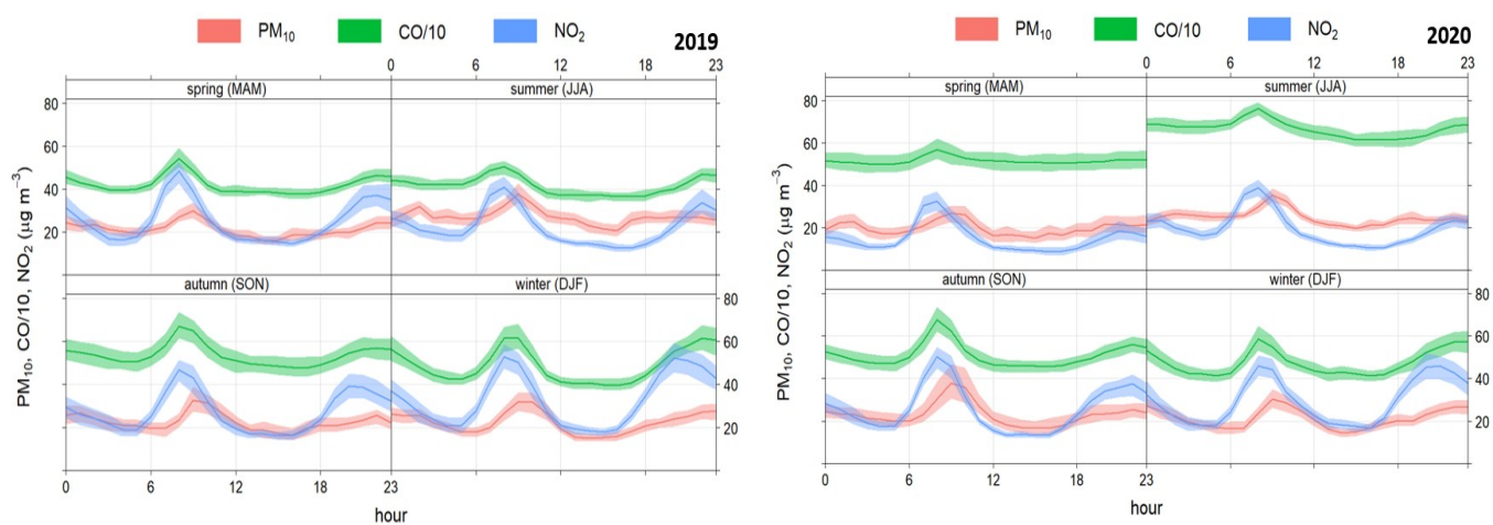
Figura 6.8. Patrón horario estacional para NO 2 , PM 10 y CO en 2019 y 2020. Estación Carranque
