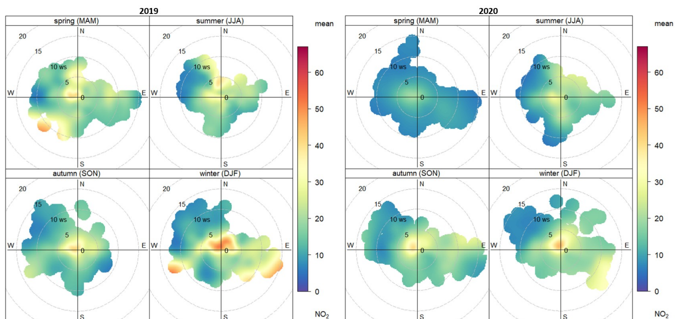
Figura 6.34. Relación entre los niveles horarios de \text{NO}_2 y la velocidad y dirección del viento en 2019 y 2020. Estación Carranque
