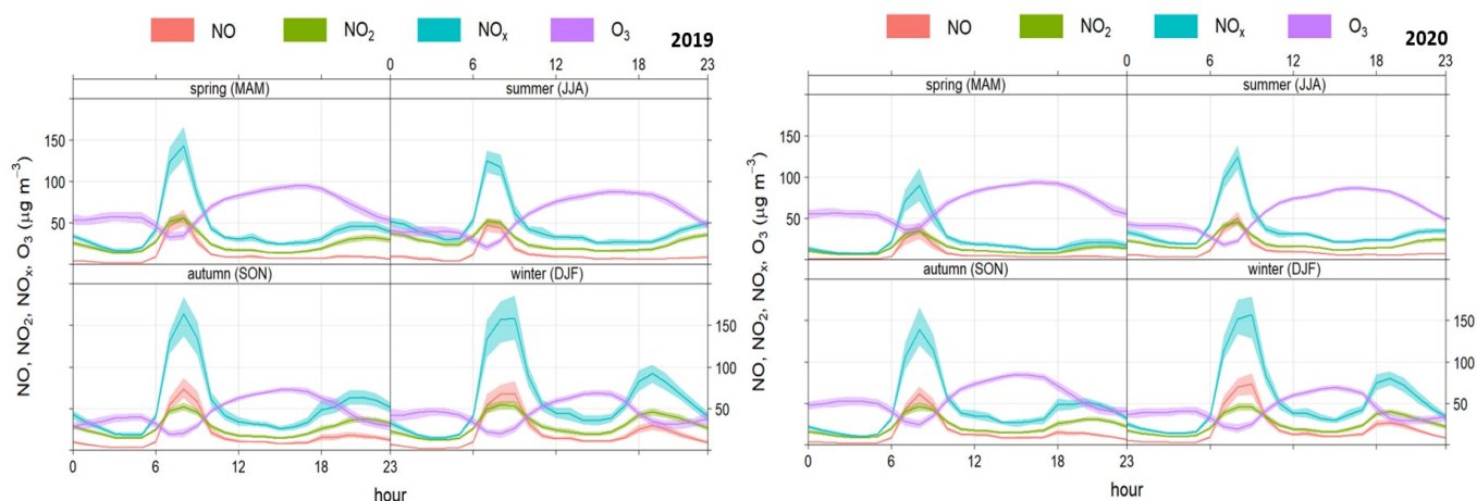
Figura 6.28. Patrón horario estacional para O 3 , NO x , NO 2 y NO en 2019 y 2020. Estación Marbella Arco
