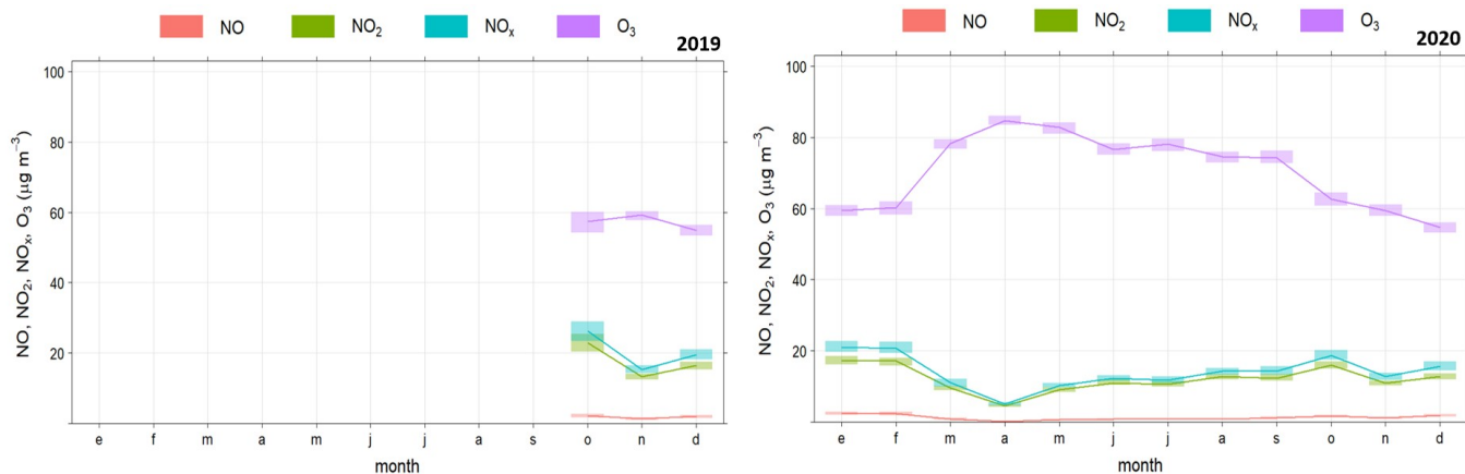
Figura 6.27. Medias mensuales de O 3 , NO x , NO 2 y NO en los años 2019 y 2020. Estación Málaga Este
