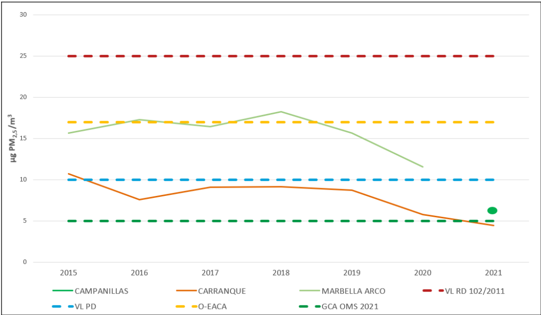
Figura 5.6. Promedio anual de PM 2,5 (µg/m³) en las estaciones de Málaga y Costa del Sol
