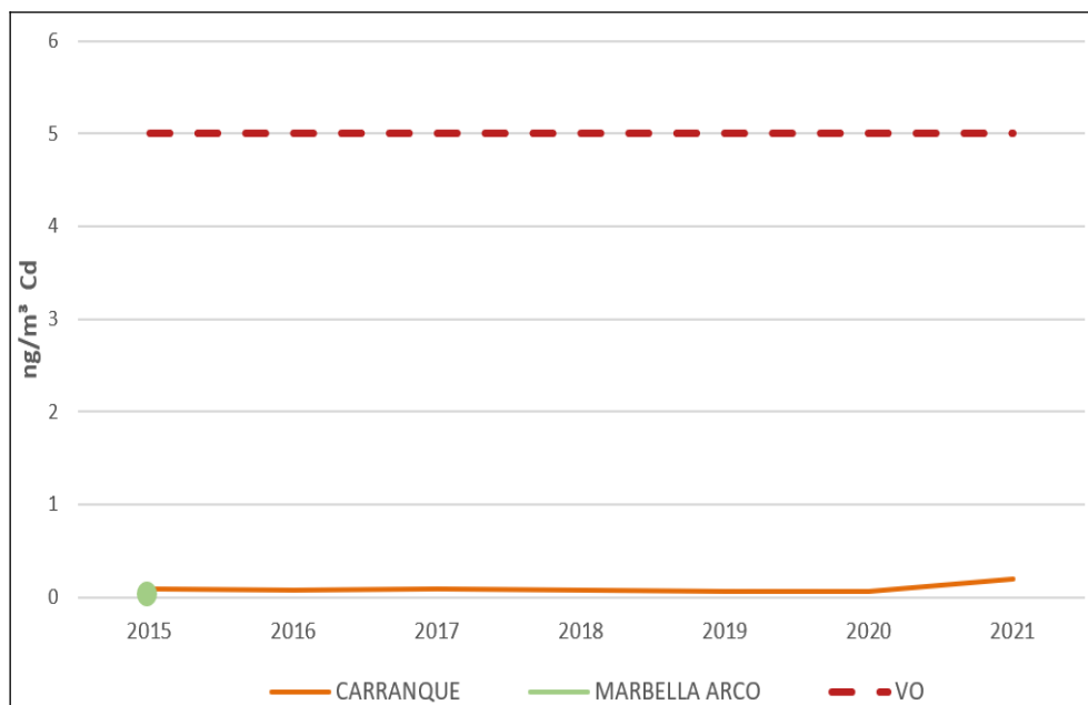
Figura 5.18. Medias anuales de Cd (ng/m³) en Málaga y Costa del Sol
