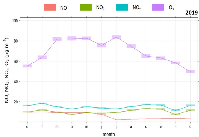
Figura 6.25. Medias mensuales de O 3 , NO x , NO 2 y NO en los años 2019 y 2020. Estación Campanillas
