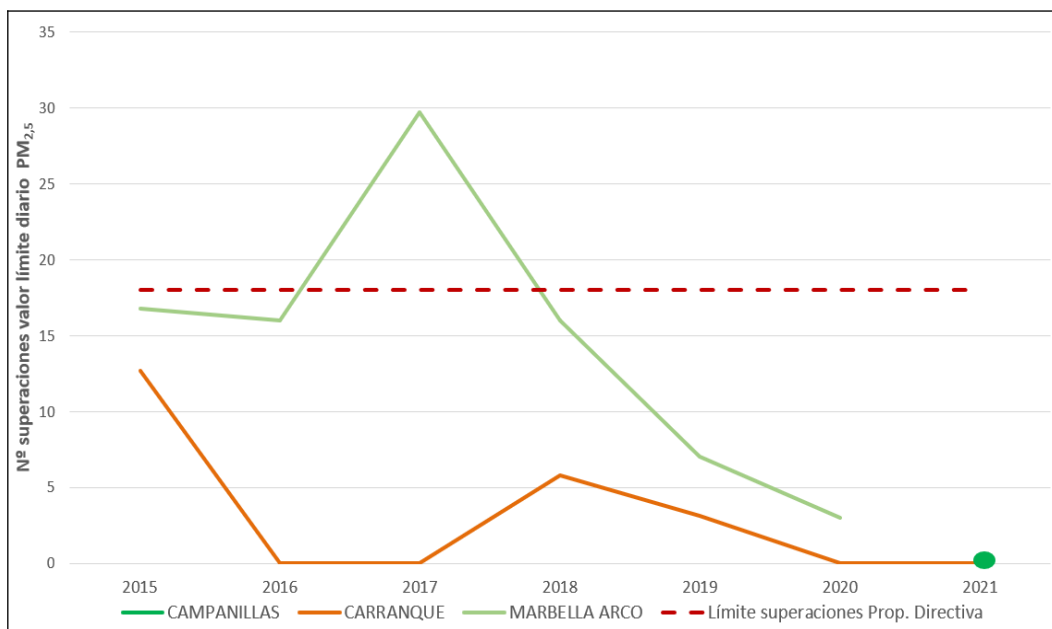
Figura 5.7. Número de superaciones del futuro valor límite diario de PM 2,5 (propuesta de directiva de calidad del aire) en Málaga y Costa del Sol
