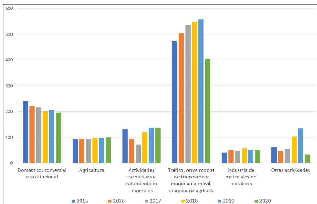
Figura 6.61. Evolución de las emisiones inventariadas de PM 10 (t/año)
