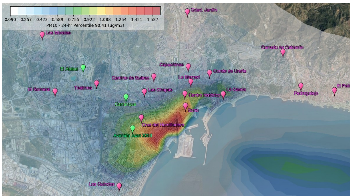
Figura AII.10. Contribución del tráfico marítimo al percentil 90,41 de los valores medios diarios de PM 10 . Escenario 2 (2 cruceros + 1 ferry)
