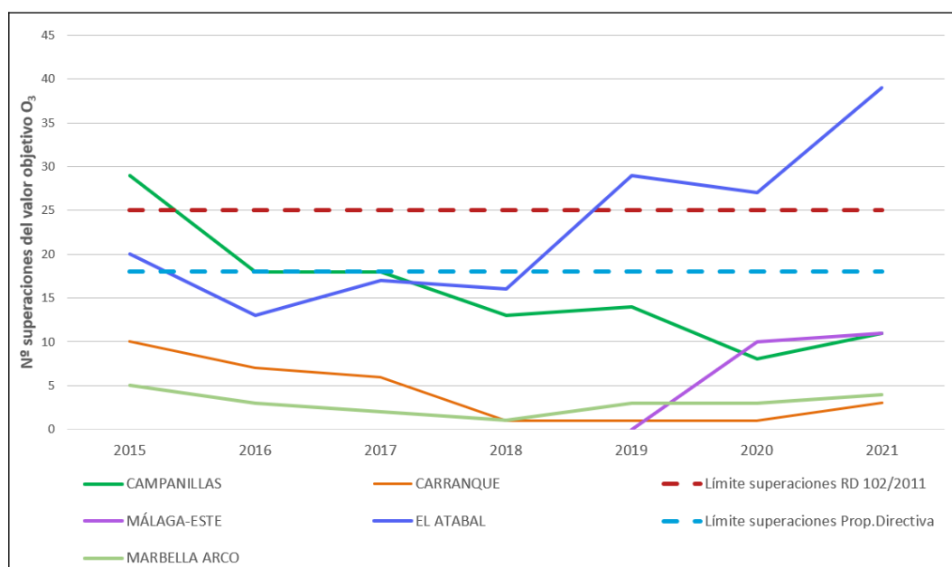
Figura 5.11. Número de superaciones del valor objetivo de ozono para la protección de la salud humana en Málaga y Costa del Sol
