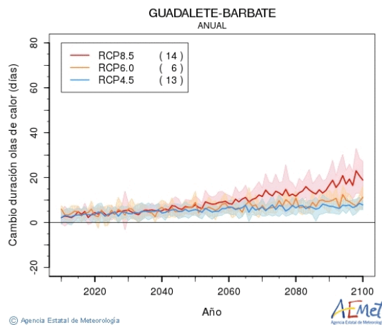
Figura nº 2. Gráficos de evolución anual de temperatura máxima (a), cambio en el número de días cálidos (b) y olas de calor (c) en la DHGB a lo largo del siglo XXI (Fuente: AEMET, 2021)
