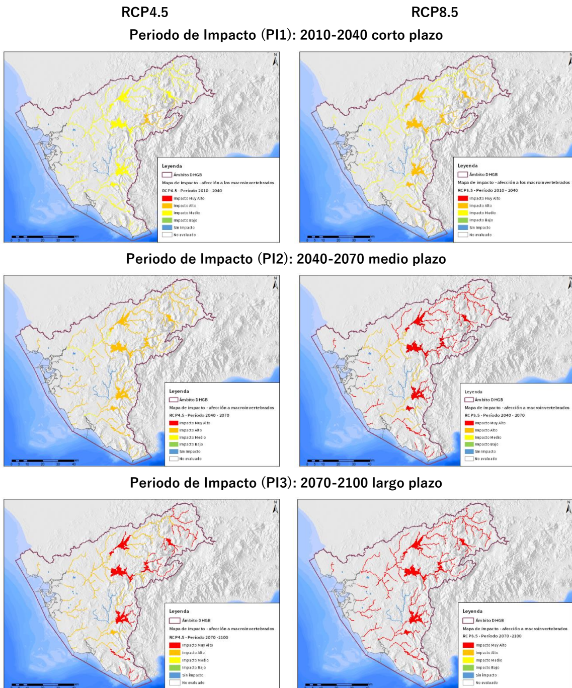
Figura nº 4. Mapas de impacto potencial en los macroinvertebrados para los dos escenarios de emisiones RCP4.5 (izquierda) y RCP8.5 (derecha), y los tres PI (2010-2040 arriba, 2040-2070 medio y 2070-2100 abajo)
