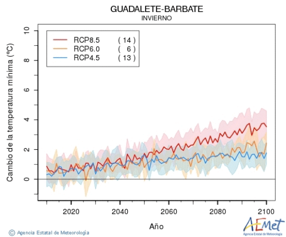
Figura nº 5. Gráficos de evolución temperatura mínima estacional en la DHGB a lo largo del siglo XXI: primavera (a), verano (b), otoño (c) e invierno (d) (Fuente: AEMET, 2021)
