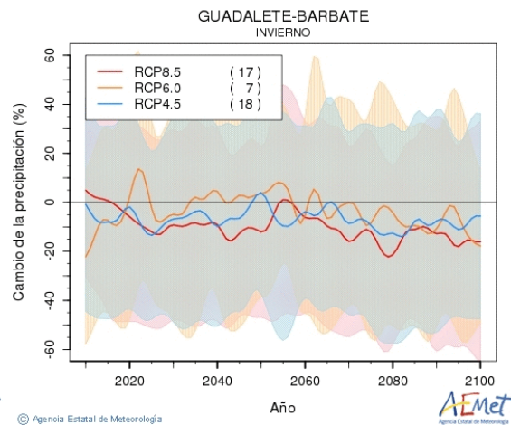
Figura nº 7. Gráficos de evolución precipitación estacional en la DHGB a lo largo del siglo XXI: primavera (a), verano (b), otoño (c) e invierno (d) (Fuente: AEMET, 2021)
