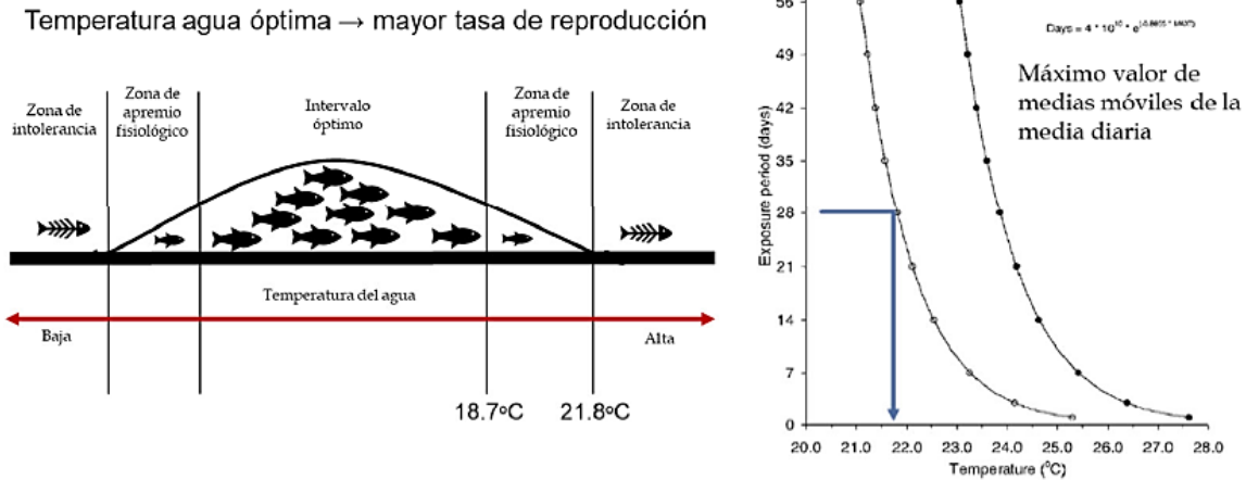
Figura nº 16. Definición de la zona de apremio y de la barrera termal de la trucha común y límites máximos de exposición en días en función de la temperatura media diaria del agua (Wehrly y Wang, 2007).
