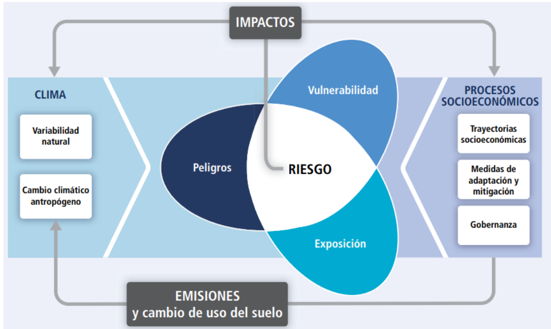
Figura nº 30. Marco conceptual para la evaluación de riesgos asociados al cambio climático. IPCC, 2014
