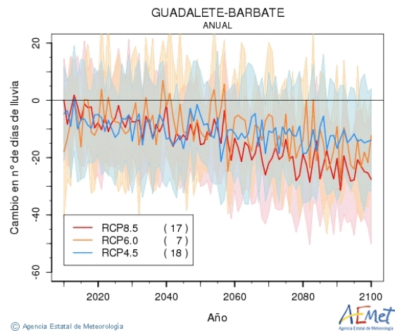
Figura nº 6. Gráficos de evolución anual de precipitación (a), cambio en precipitaciones intensas (b), cambio en periodos secos (c) y cambio en el número de días de lluvia (d) en la DHGB a lo largo del siglo XXI (Fuente: AEMET, 2021)
