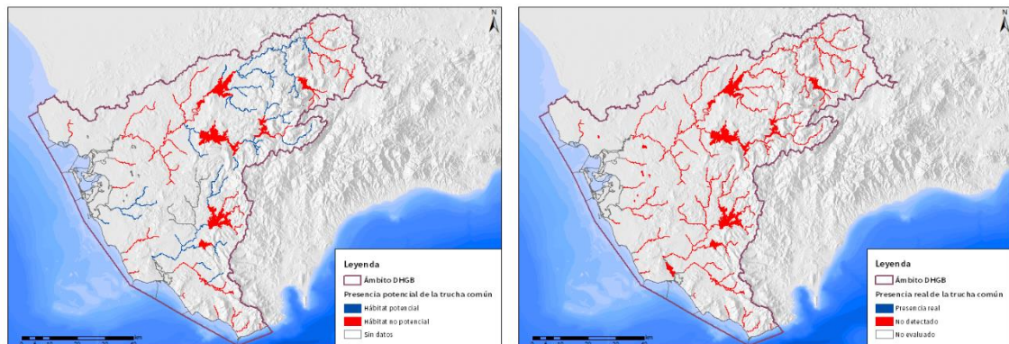
Figura nº 17. Mapa de Exposición. Hábitat potencial calculado con el límite termal de 21,8°C (izquierda) y adaptación de la presencia de la trucha común a las masas de agua superficiales (MMA, 2001) (derecha)
