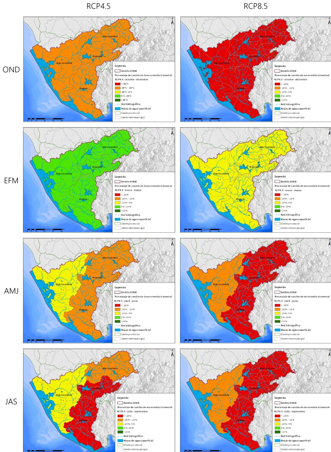
Figura nº 11. Porcentaje de cambio de la escorrentía trimestral (OND, EFM, AMJ, JAS) por sistema en la DHGB para el horizonte 2039. Escenario RCP4.5 (izquierda) y RCP8.5 (derecha). Los colores reflejan la gradación del cambio
