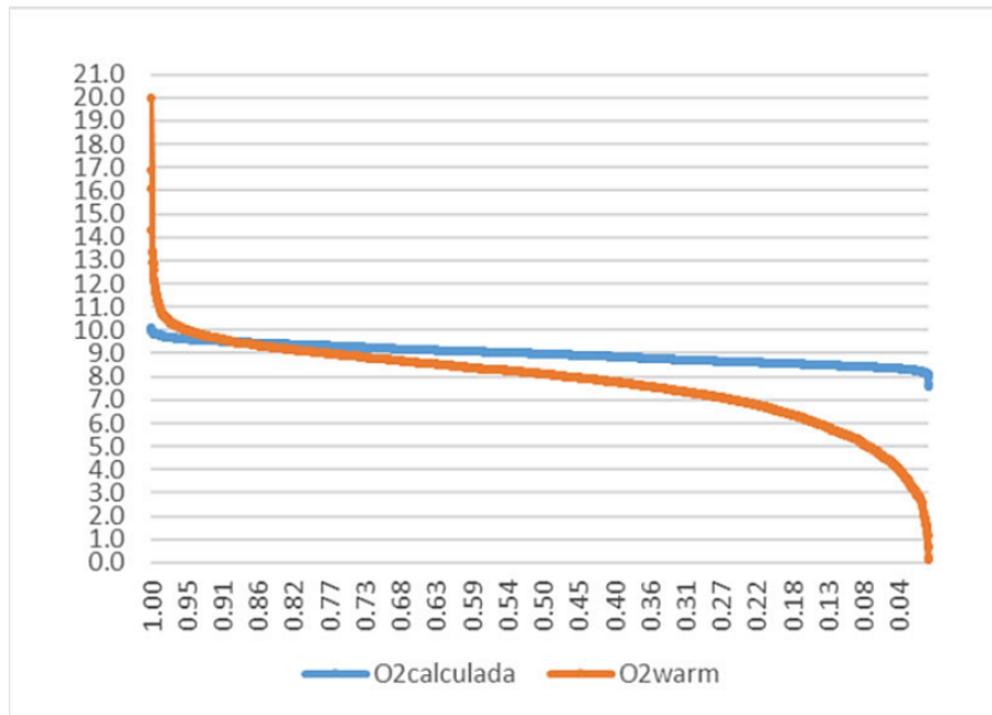
Figura nº 21. Distribución de la concentración de oxígeno disuelto en agua calculada, en función de la temperatura y la altitud, y observada (mg/l)
