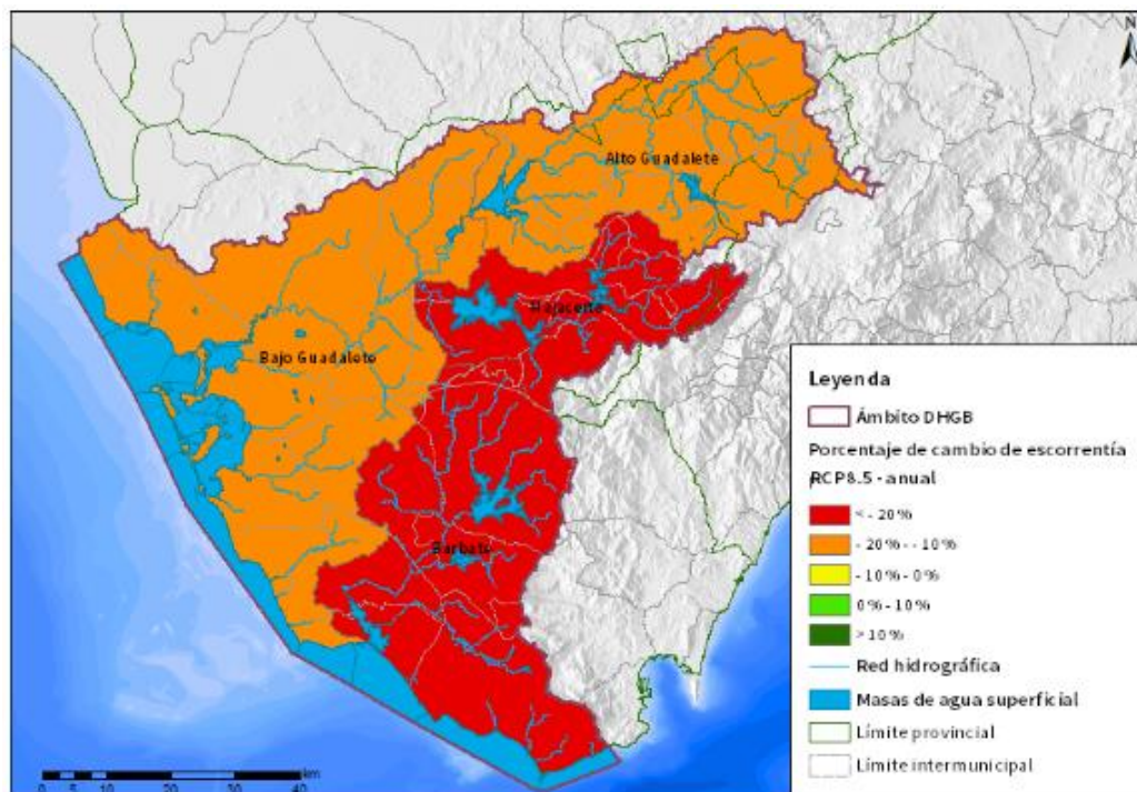
Figura nº 10. Porcentaje de cambio de la escorrentía medio anual por sistema en la DHGB para el horizonte 2039. Escenario RCP4.5 (izquierda) y RCP8.5 (derecha). Los colores reflejan la gradación del cambio.
