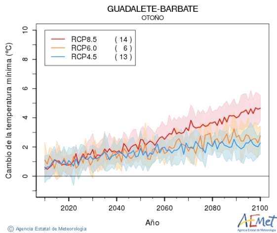
Figura nº 5. Gráficos de evolución temperatura mínima estacional en la DHGB a lo largo del siglo XXI: primavera (a), verano (b), otoño (c) e invierno (d) (Fuente: AEMET, 2021)
