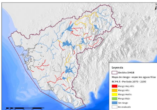
Figura nº 5. Mapas de riesgo sobre la pérdida de hábitat para especies de aguas frías para los dos escenarios de emisiones RCP4.5 (izquierda) y RCP8.5 (derecha), y los tres PI (2010-2040 arriba, 2040-2070 medio y 2070-2100 abajo)
