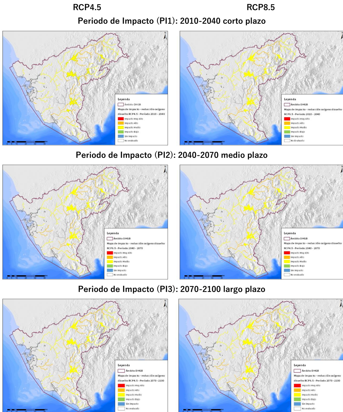
Figura nº 3. Mapas de impacto potencial en el oxígeno disuelto para los dos escenarios de emisiones RCP4.5 (izquierda) y RCP8.5 (derecha), y los tres PI (2010-2040 arriba, 2040-2070 medio y 2070-2100 abajo)
