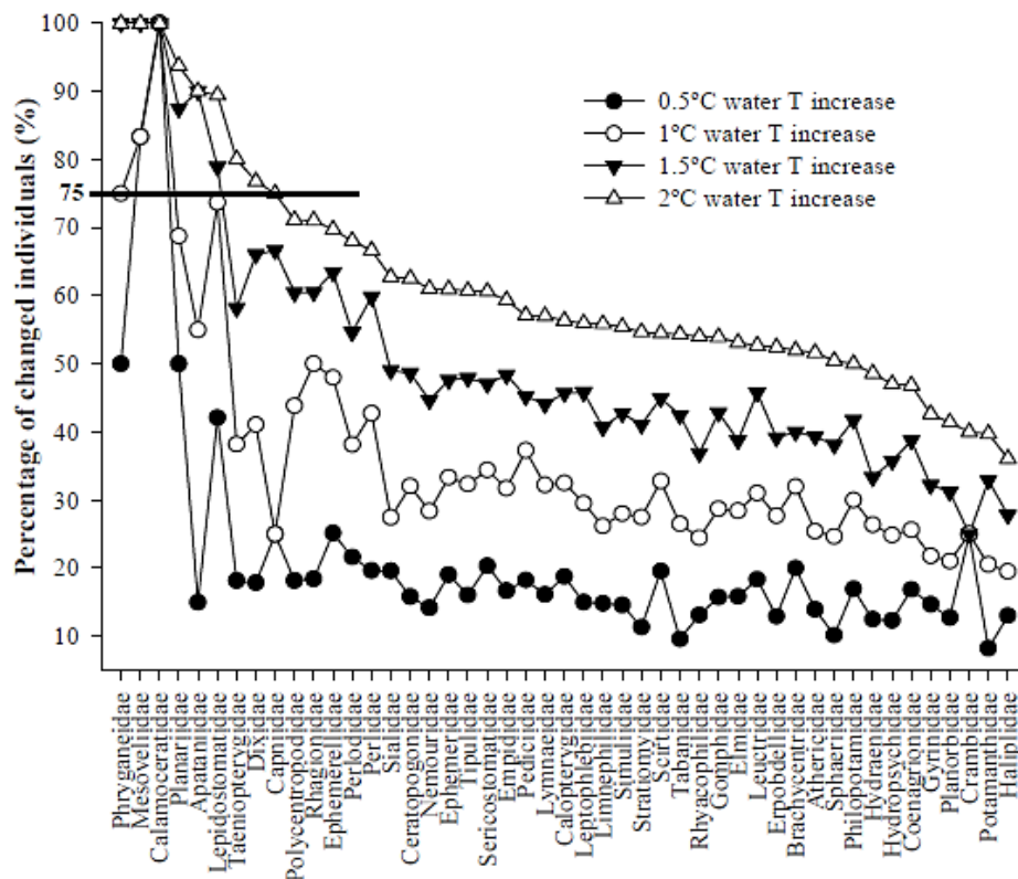
Figura nº 26. Porcentaje de individuos por familia que experimentan un cambio como resultado de incrementos en la temperatura del agua (Método del Óptimo Robusto)
