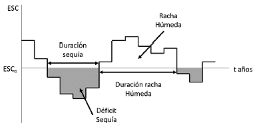
Figura nº 12. Concepto y definición de sequía (CEDEX, 2017)
