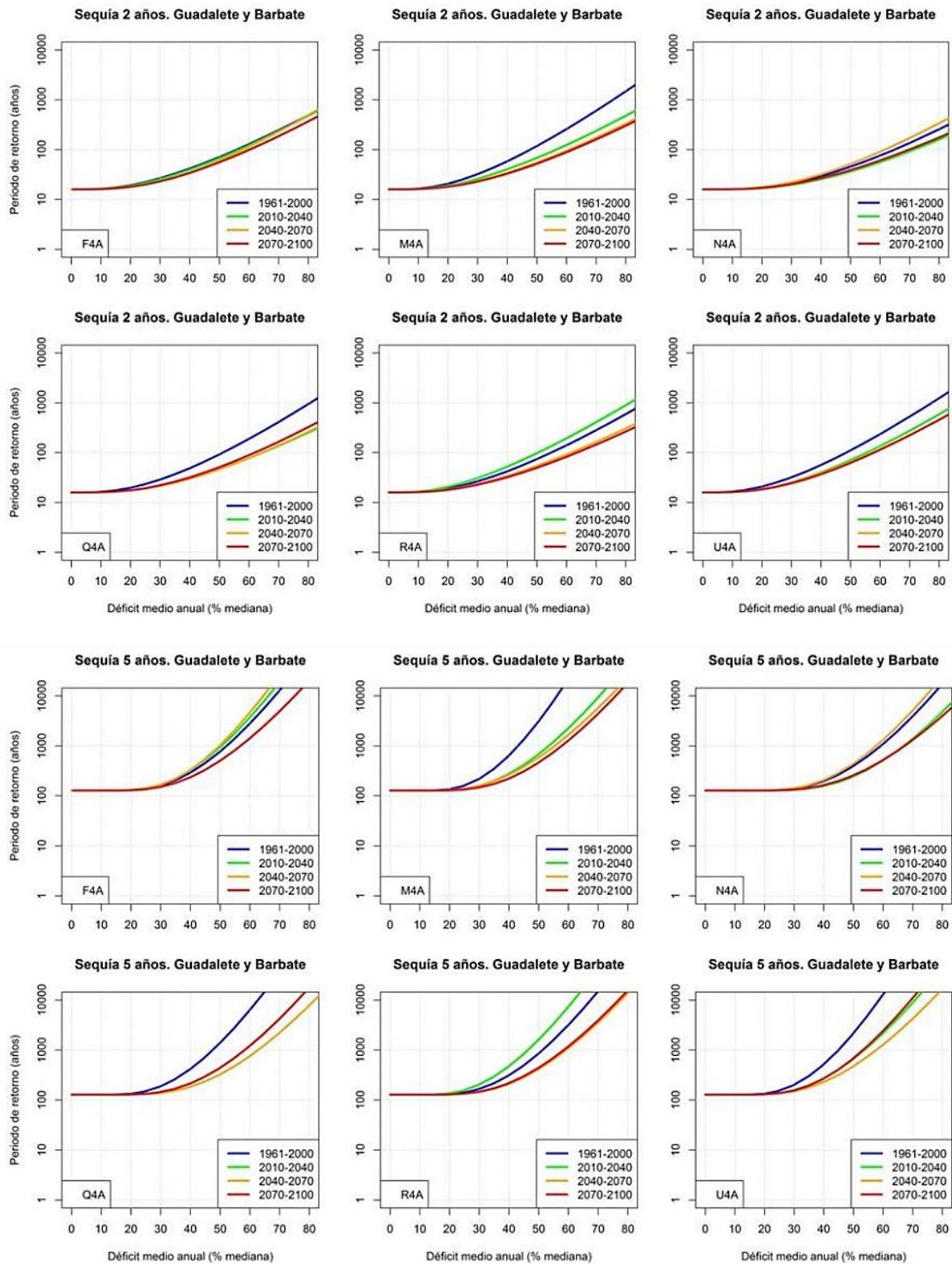
Figura nº 13. Periodo de retorno de sequías en la DHGB para diferentes déficits medios anuales y duración 2 años (arriba) y 5 años (debajo) para el PC y los tres PI según cada una de las proyecciones. Escenario RCP4.5.
