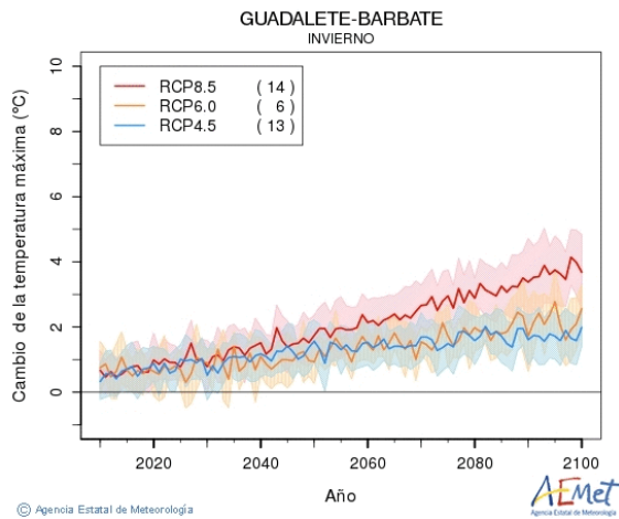
Figura nº 3. Gráficos de evolución temperatura máxima estacional en la DHGB a lo largo del siglo XXI: primavera (a), verano (b), otoño (c) e invierno (d) (Fuente: AEMET, 2021)
