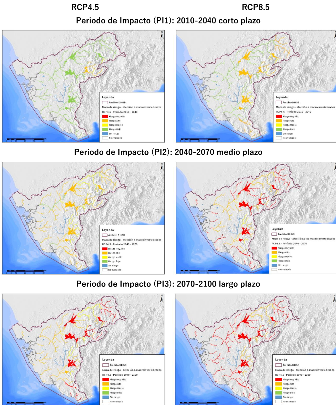
Figura nº 7. Mapas de riesgo en los macroinvertebrados para los dos escenarios de emisiones RCP4.5 (izquierda) y RCP8.5 (derecha), y los tres PI (2010-2040 arriba, 2040-2070 medio y 2070-2100 abajo)
