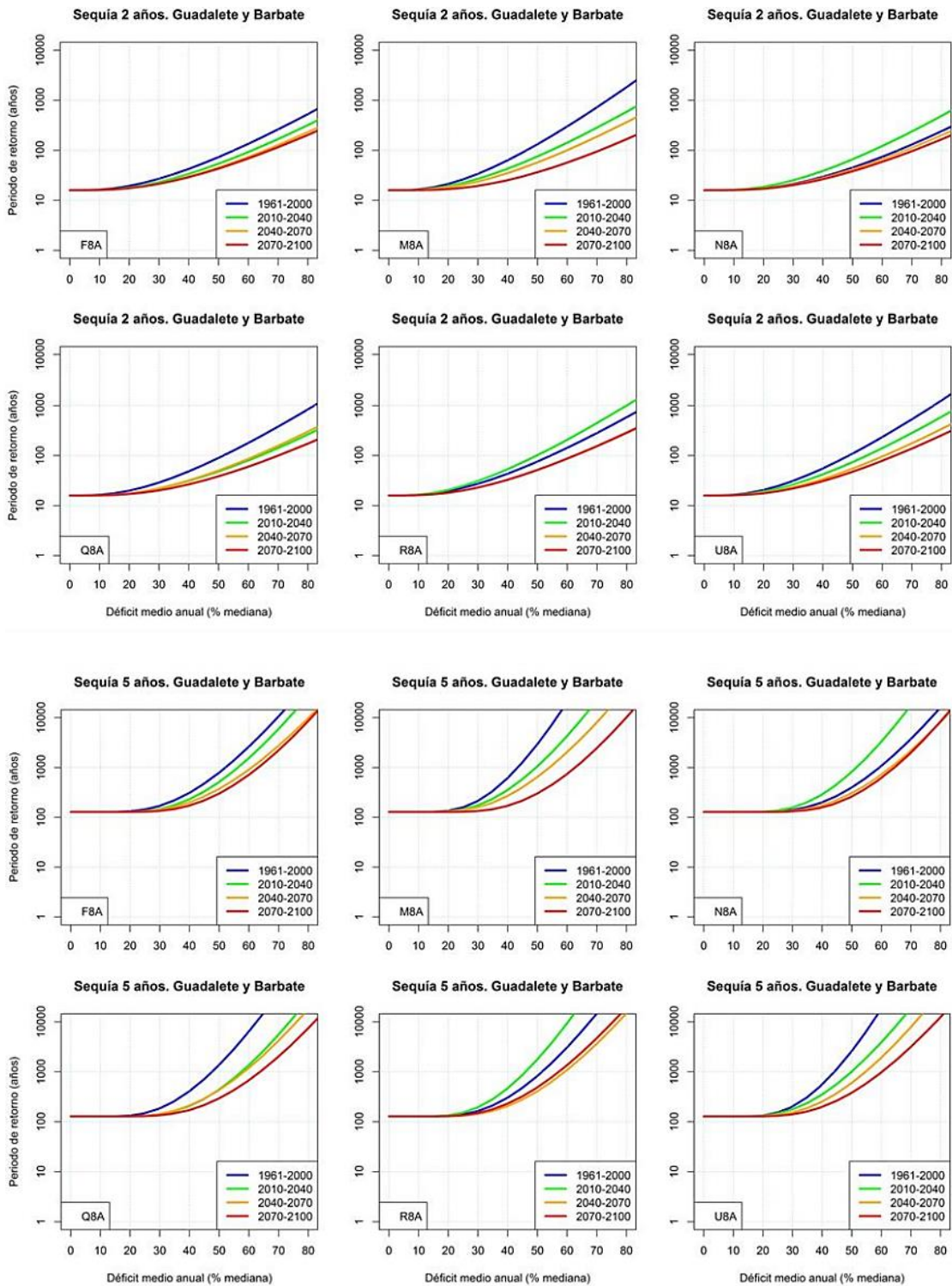
Figura nº 14. Periodo de retorno de sequías en la DHGB para diferentes déficits medios anuales y duración 2 años (arriba) y 5 años (debajo) para el PC y los tres PI según cada una de las proyecciones. Escenario RCP 8.5.
