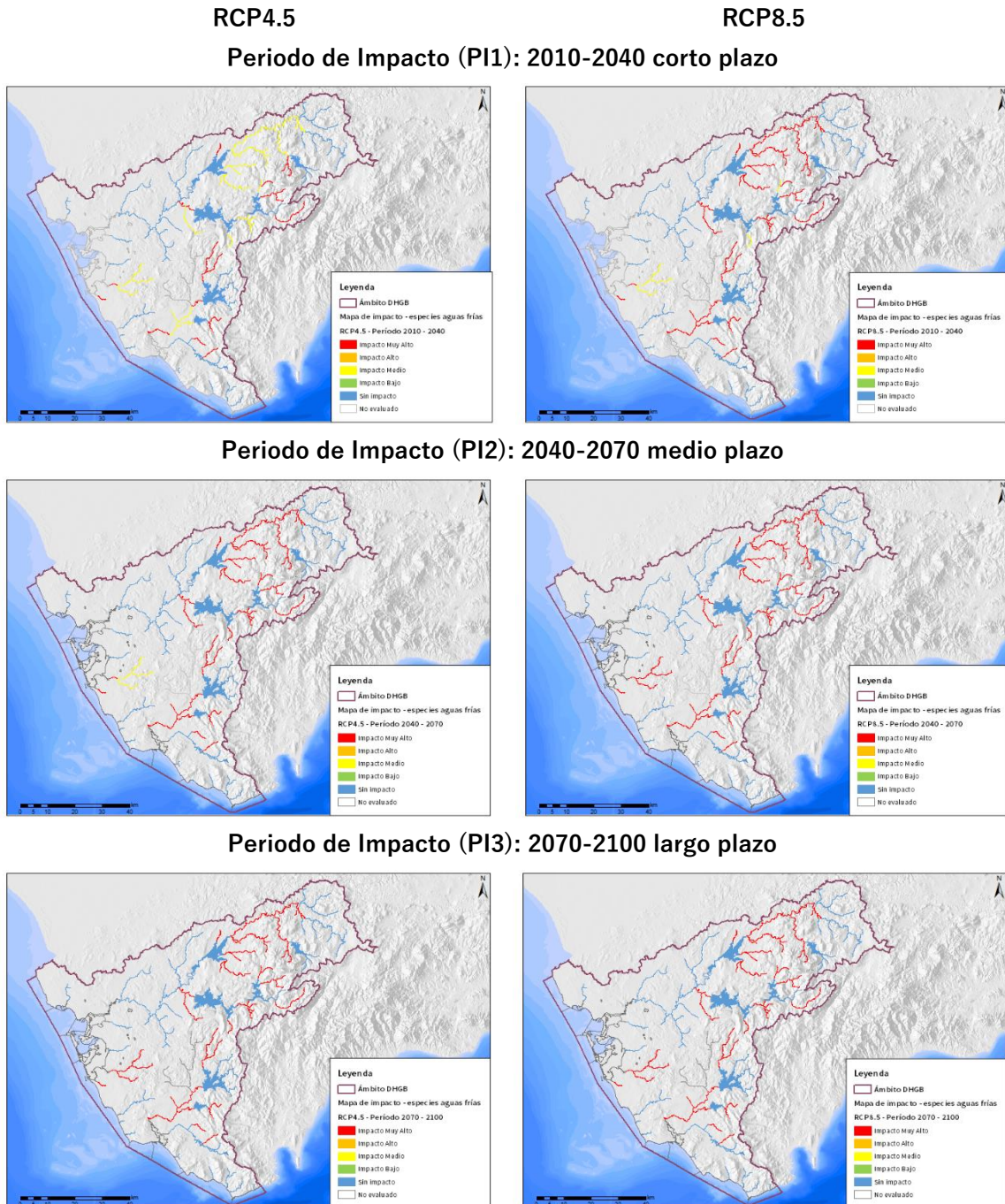
Figura nº 2. Mapas de impacto potencial sobre la pérdida de hábitat para especies de aguas frías para los dos escenarios de emisiones RCP4.5 (izquierda) y RCP8.5 (derecha), y los tres PI (2010-2040 arriba, 2040-2070 medio y 2070-2100 abajo)
