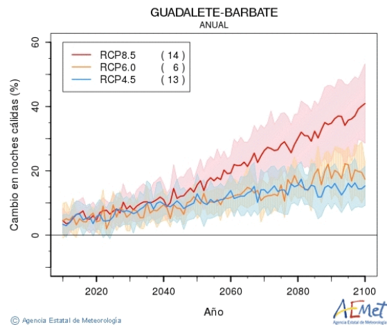
Figura nº 4. Gráficos de evolución anual de temperatura mínima (a), número de días de heladas (b) y noches cálidas (c) en la DHGB a lo largo del siglo XXI (Fuente: AEMET, 2021)
