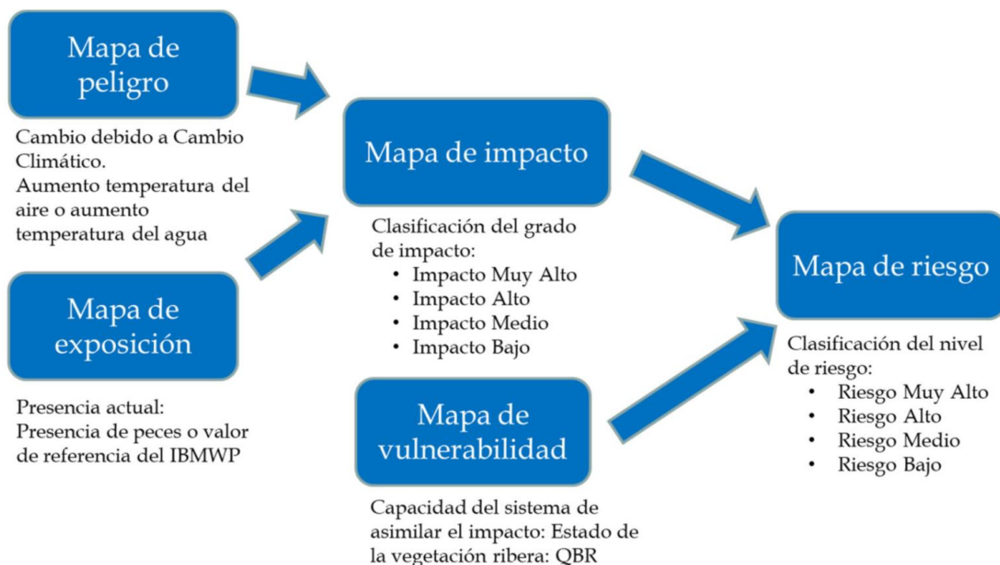
Figura nº 15. Metodología propuesta para la definición del riesgo asociado al cambio climático (Pérez Martín, 2020)
