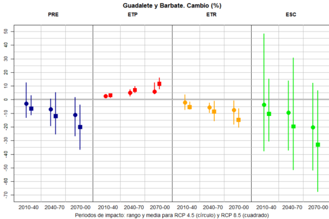
Figura nº 8. Cambio (%) en las principales variables hidrológicas en los tres PI respecto al PC para la DHGB. Rango y media de resultados para RCP 4.5 (círculos) y RCP 8.5 (cuadrados).
