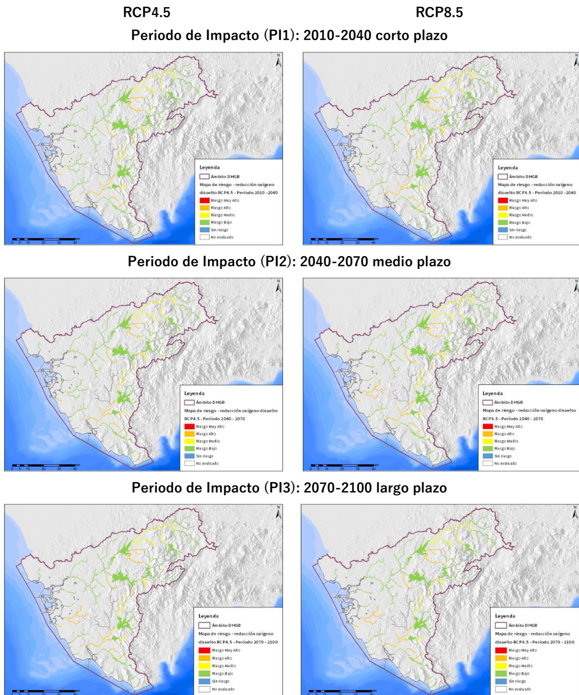
Figura nº 6. Mapas de riesgo en el oxígeno disuelto para los dos escenarios de emisiones RCP4.5 (izquierda) y RCP8.5 (derecha), y los tres PI (2010-2040 arriba, 2040-2070 medio y 2070-2100 abajo)
