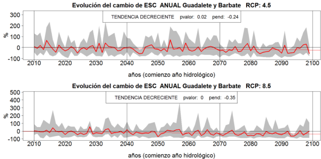
Figura nº 9. Tendencia del \Delta (%) escorrentía del año 2010 al 2099 para los RCP4.5 (arriba) y RCP8.5 (abajo) en la DHGB (CEH, 2017).
