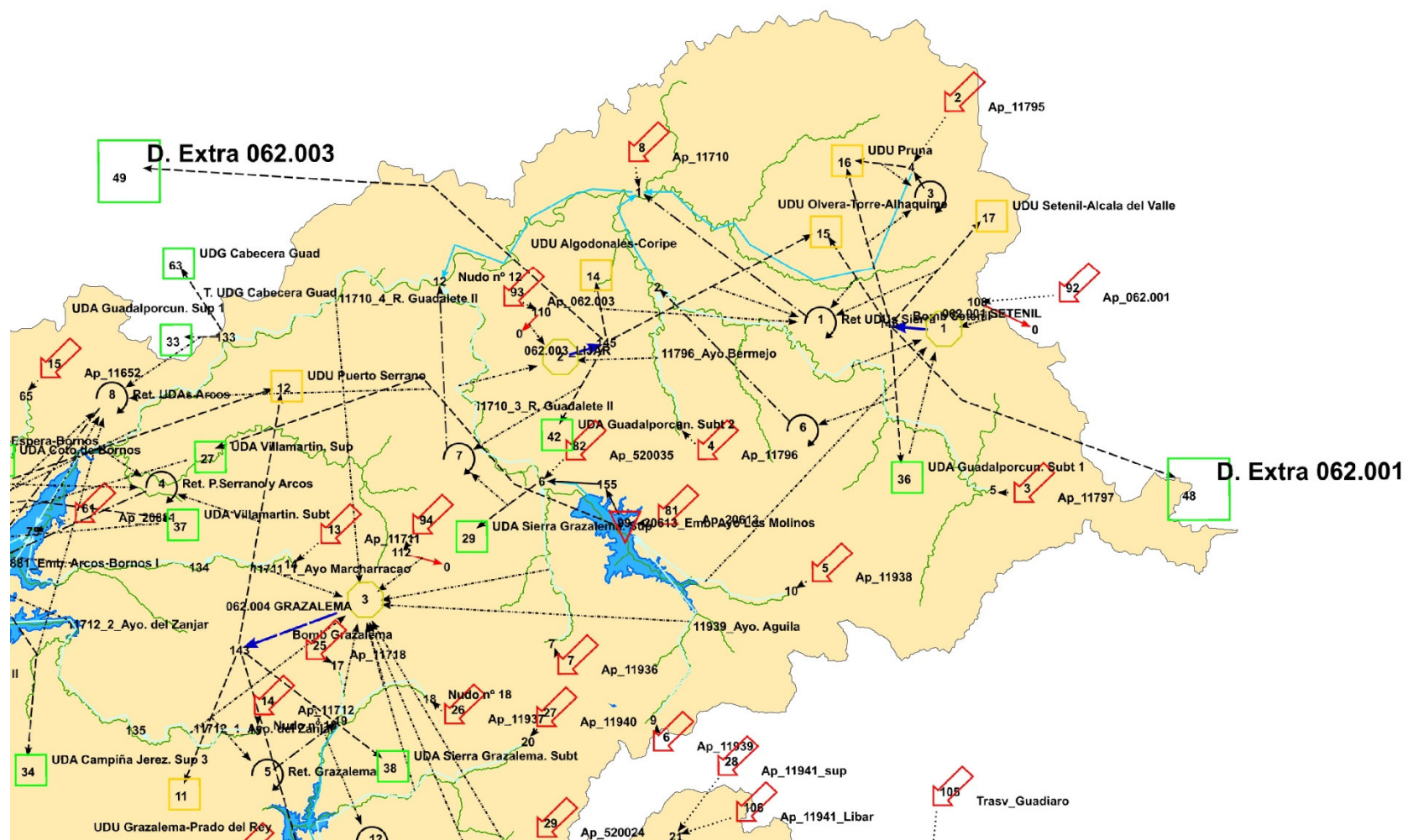
Figura nº 12. Detalle del esquema del modelo de simulación en la cabecera del río Guadalete
