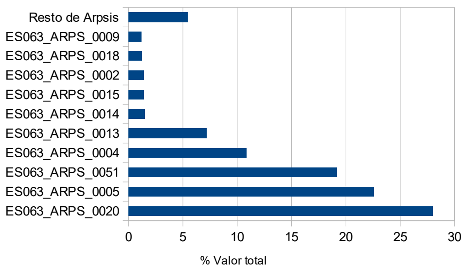
Figura 19. Usos del suelo con mayor valor económico en riesgo en las Arpsis de la demarcación T-500
