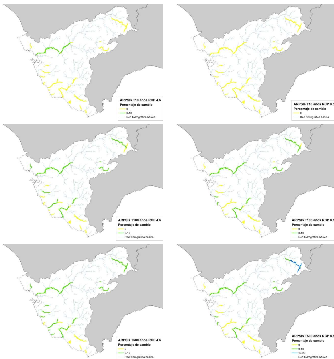
Figura 28. Tasas de cambio en cuantil de precipitación diaria máxima anual acumulada para las ARPSIs fluviales de la DH del Guadalete y Barbate para el periodo de impacto 2041-2070 en relación al modelo SQRT-R para los periodos de retorno de 10 (arriba), 100 (medio) y 500 años (abajo) y RCP 4.5 (izquierda) y 8.5 (derecha)
