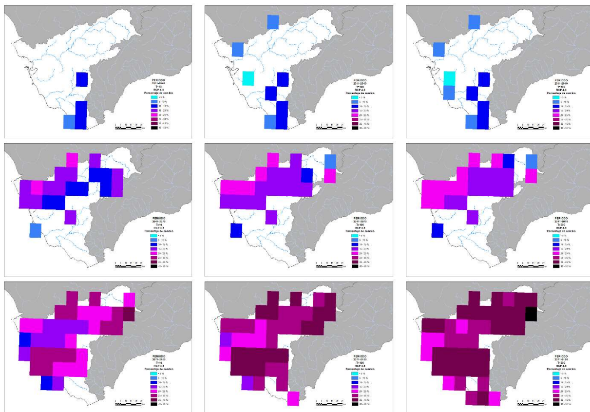
Figura 20. Tasas de cambio en cuantil medias significativas para precipitación horaria máxima anual en base a modelos climáticos comunes para el modelo SQRT-R en RCP 4.5 en la DH del Guadalete y Barbate
