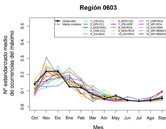
Figura 12. Contraste de la estacionalidad de la precipitación diaria máxima anual obtenida mediante observaciones y simulaciones en la región “0603” de la DH del Guadalete y Barbate
