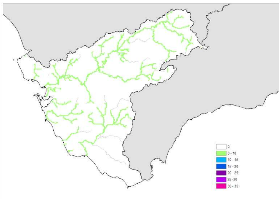
Figura 24. Tasas de cambio en cuantil de precipitación diaria máxima anual acumulada para el periodo de impacto 2041-2070 en relación al modelo SQRT-R para RCP 4.5 y T= 500 años
