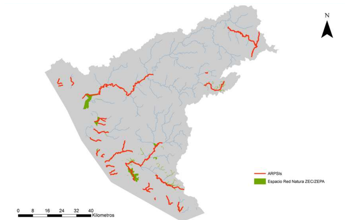
Figura 27. Espacios de la Red Natura afectados por inundabilidad para el escenario T-500
