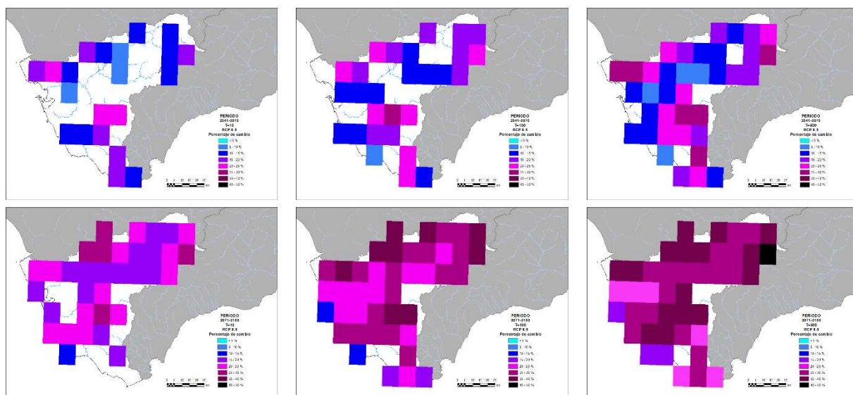
Figura 21. Tasas de cambio en cuantil medias significativas para precipitación horaria máxima anual en base a modelos climáticos comunes para el modelo SQRT-R en RCP 8.5 en la DH del Guadalete y Barbate
