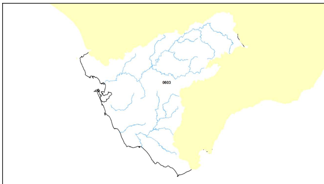
Figura 10. Región climática situada parcialmente en la DH del Guadalete y Barbate
