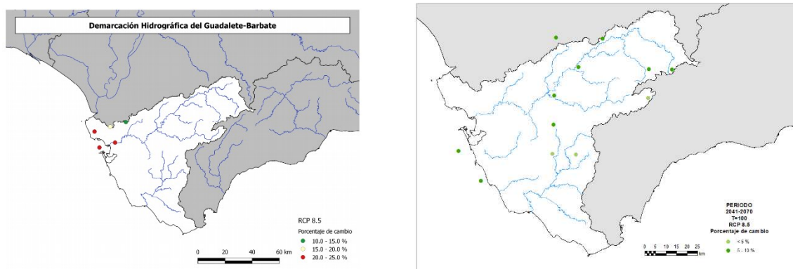
Figura 19. Celdas con tasas de cambio significativas para el periodo de impacto “2041-2070” y RCP 4.5 (arriba) y 8.5 (abajo), asociadas al periodo de retorno de 100 años, obtenidas en MITECO (2018) (izquierda) y, para el modelo SQRT-R, en CEDEX (2021) (derecha)
