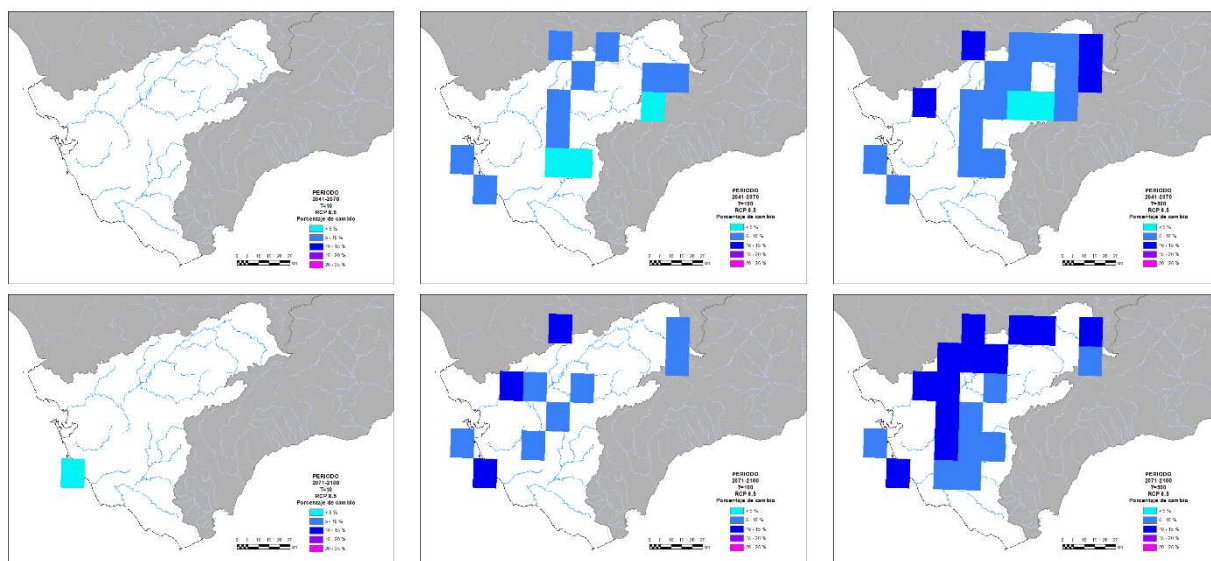
Figura 16. Tasas de cambio en cuantil medias significativas para precipitación diaria máxima anual en base a modelos climáticos comunes para el modelo SQRT-R en RCP 8.5
