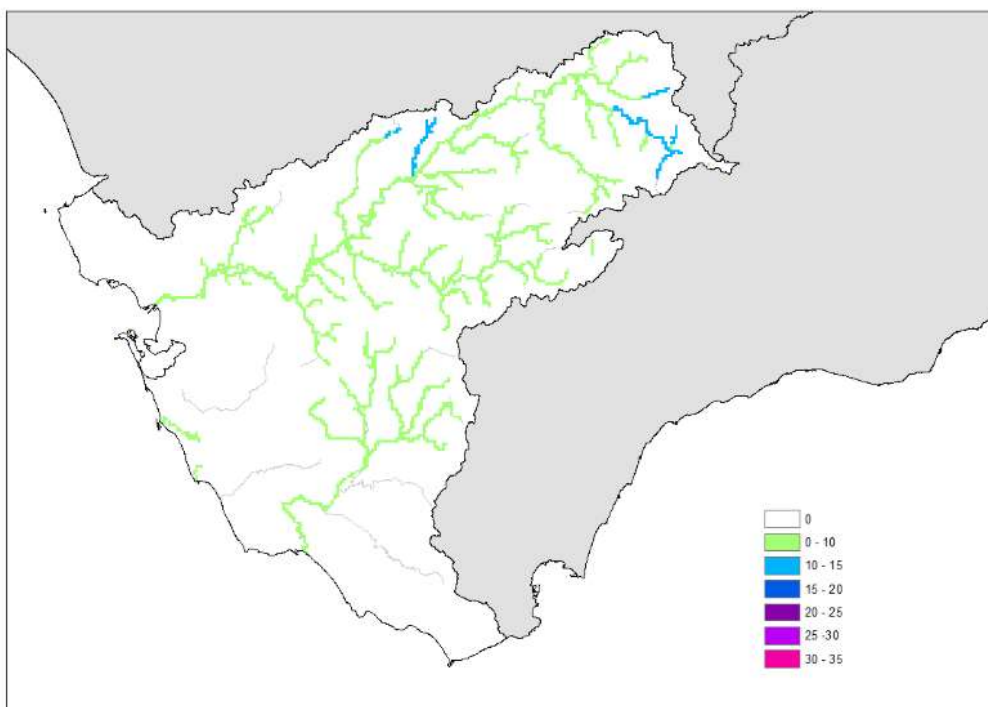
Figura 27. Tasas de cambio en cuantil de precipitación diaria máxima anual acumulada en la DH del Guadalete y Barbate para el periodo de impacto 2041-2070 en relación al modelo SQRT-R para RCP 8.5 y T = 500 años
