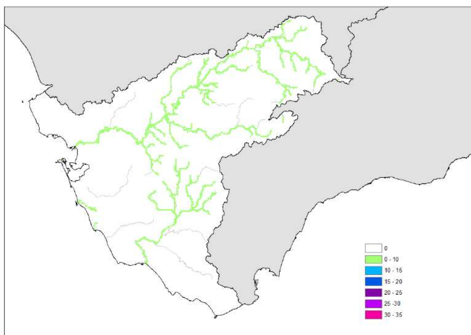
Figura 26. Tasas de cambio en cuantil de precipitación diaria máxima anual acumulada para el periodo de impacto 2041-2070 en relación al modelo SQRT-R para RCP 8.5 y T = 100 años
