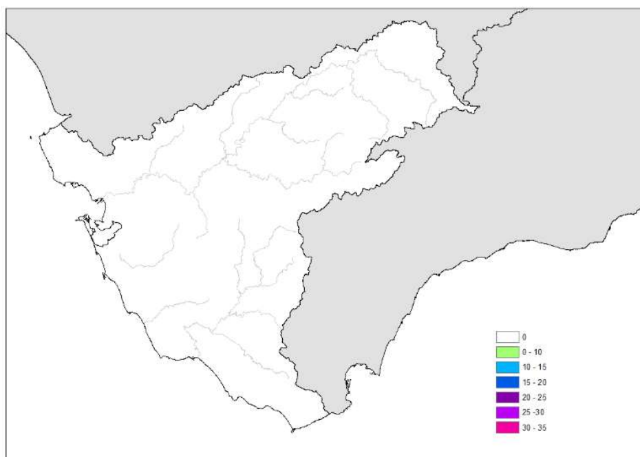
Figura 25. Tasas de cambio en cuantil de precipitación diaria máxima anual acumulada para el periodo de impacto 2041-2070 en relación al modelo SQRT-R para RCP 8.5 y T = 10 años
