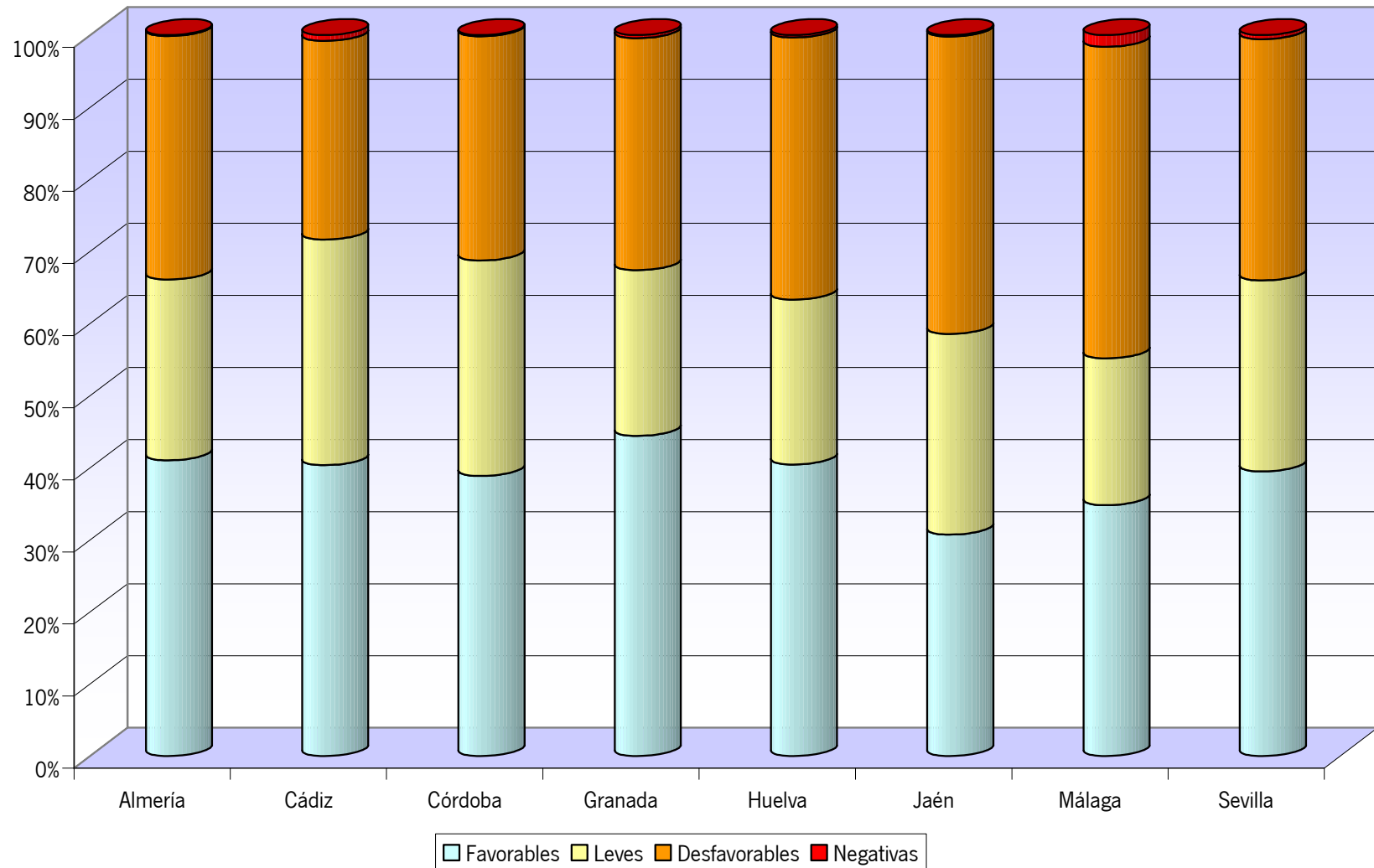
5.1.12. Gráfico. Mercancías P.M.A. > 3500 Kg. según el resultado de la inspección
