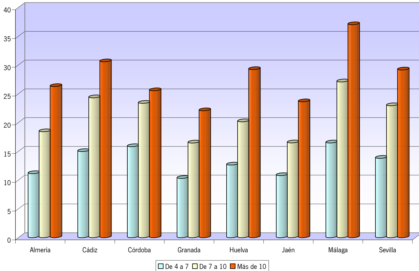
5.1.6. Gráfico. Turismos particulares. Porcentaje de rechazo según antigüedad del vehículo
