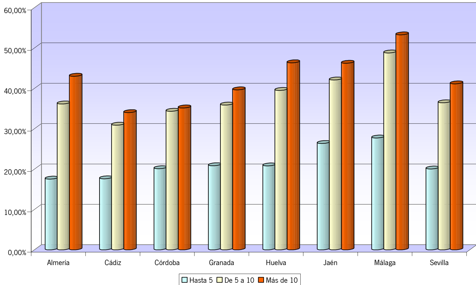
5.1.8. Gráfico. Mercancías P.M.A. > 3500 Kg. Porcentaje de rechazo según antigüedad del vehículo
