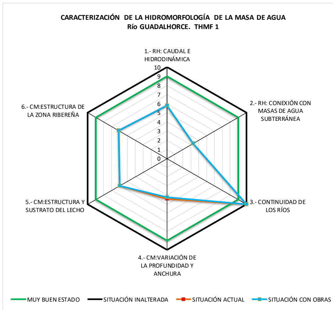
Figura 16: Esquema de valoración ponderada en el río Guadalhorce, Málaga.
