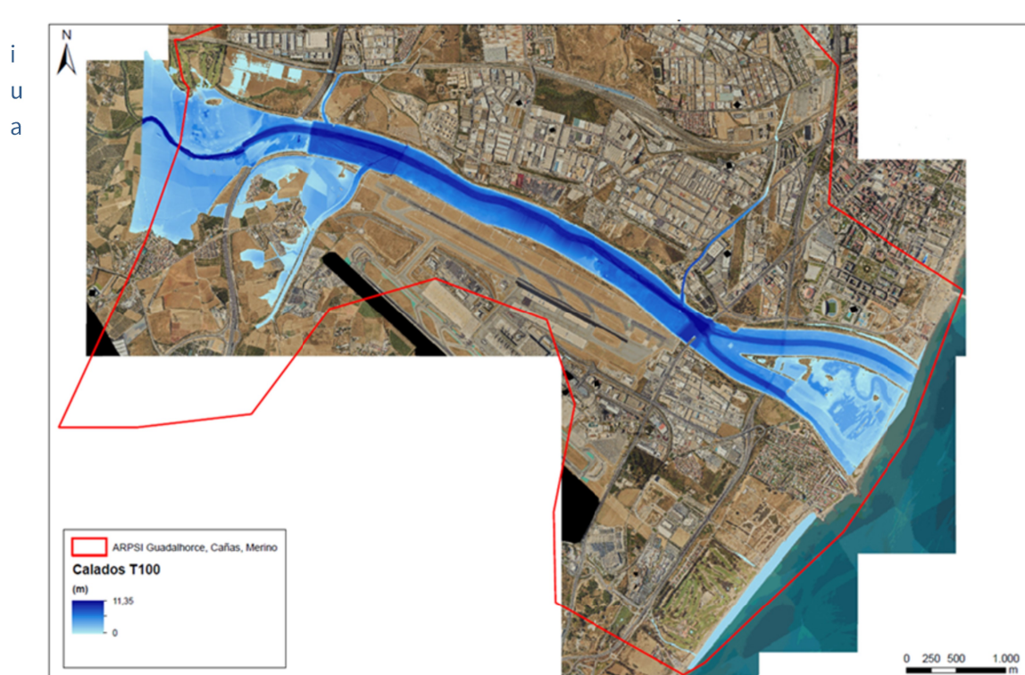
5. Situación prevista con la ejecución de las 3 Fases con la sustitución del puente de la MA-21
