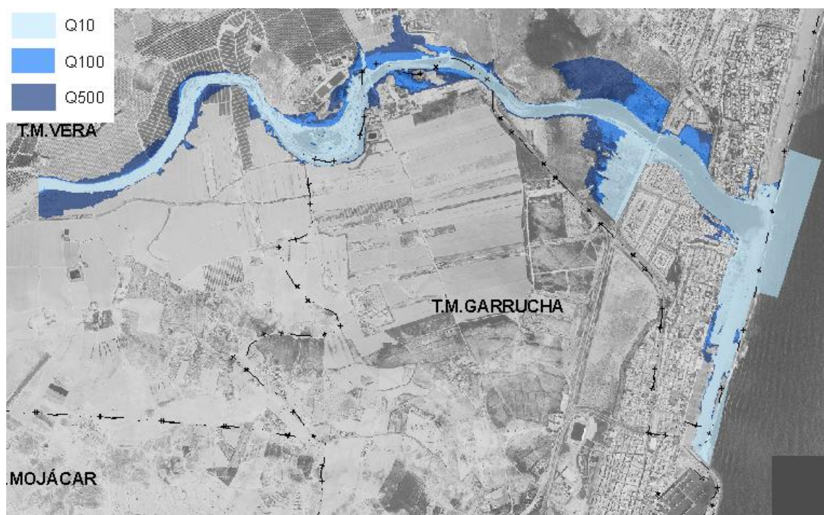
Figura 22: Detalle de la zona inundable de la alternativa 4.
