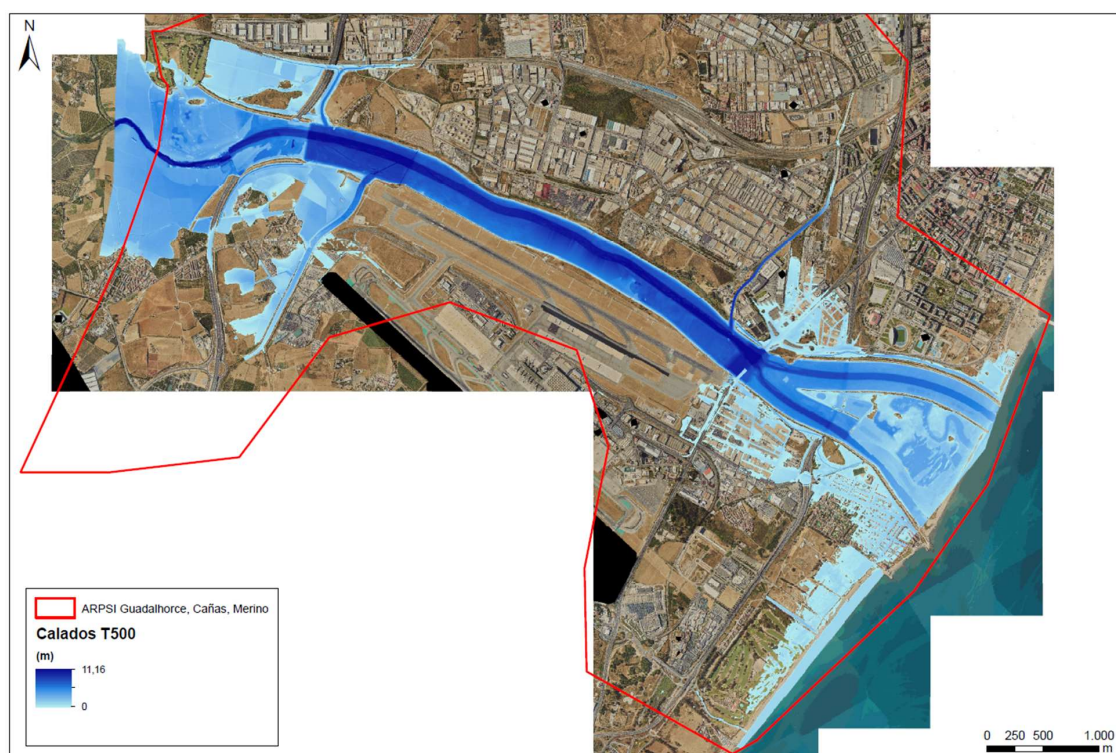
Figura 4. Situación prevista con la ejecución de las 3 Fases aumentando la sección del puente de la MA-21
