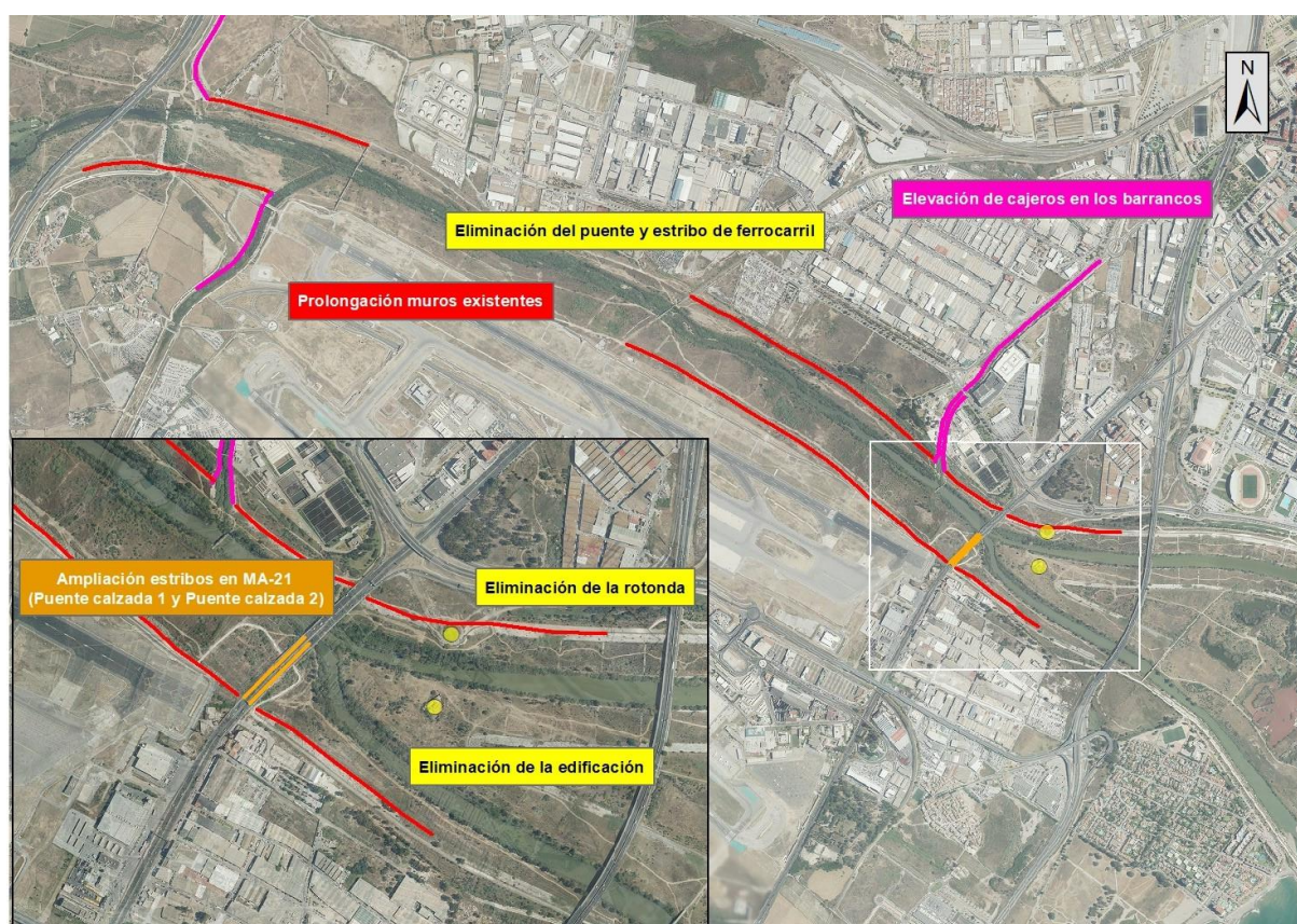
Figura 5: Croquis de la Alternativa 2
