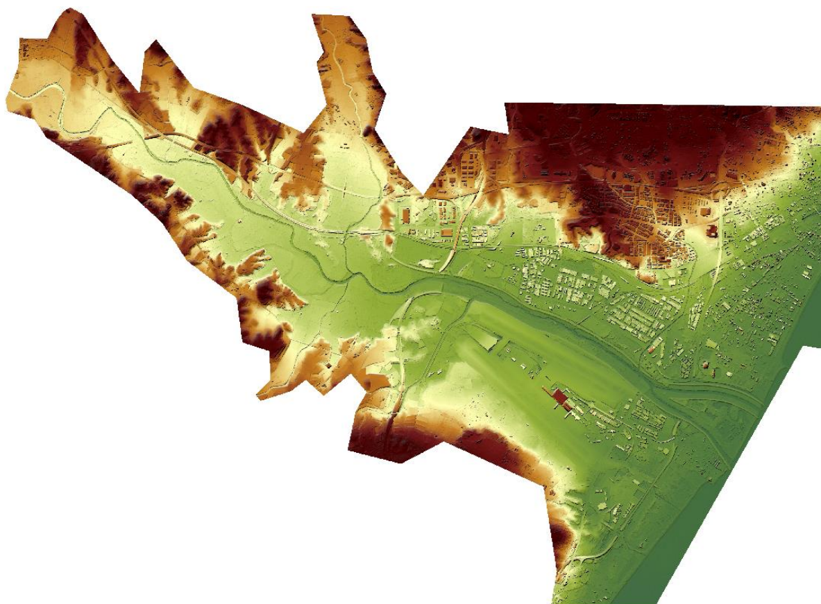
Figura 6: MDT generado para la alternativa 0.
