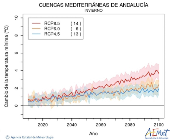
Figura nº 5. Gráficos de cambio de temperatura mínima estacional: (a) primavera, (b) verano, (c) otoño y (d) invierno en la DHCMa a lo largo del siglo XXI (Fuente: AEMET, 2021).
