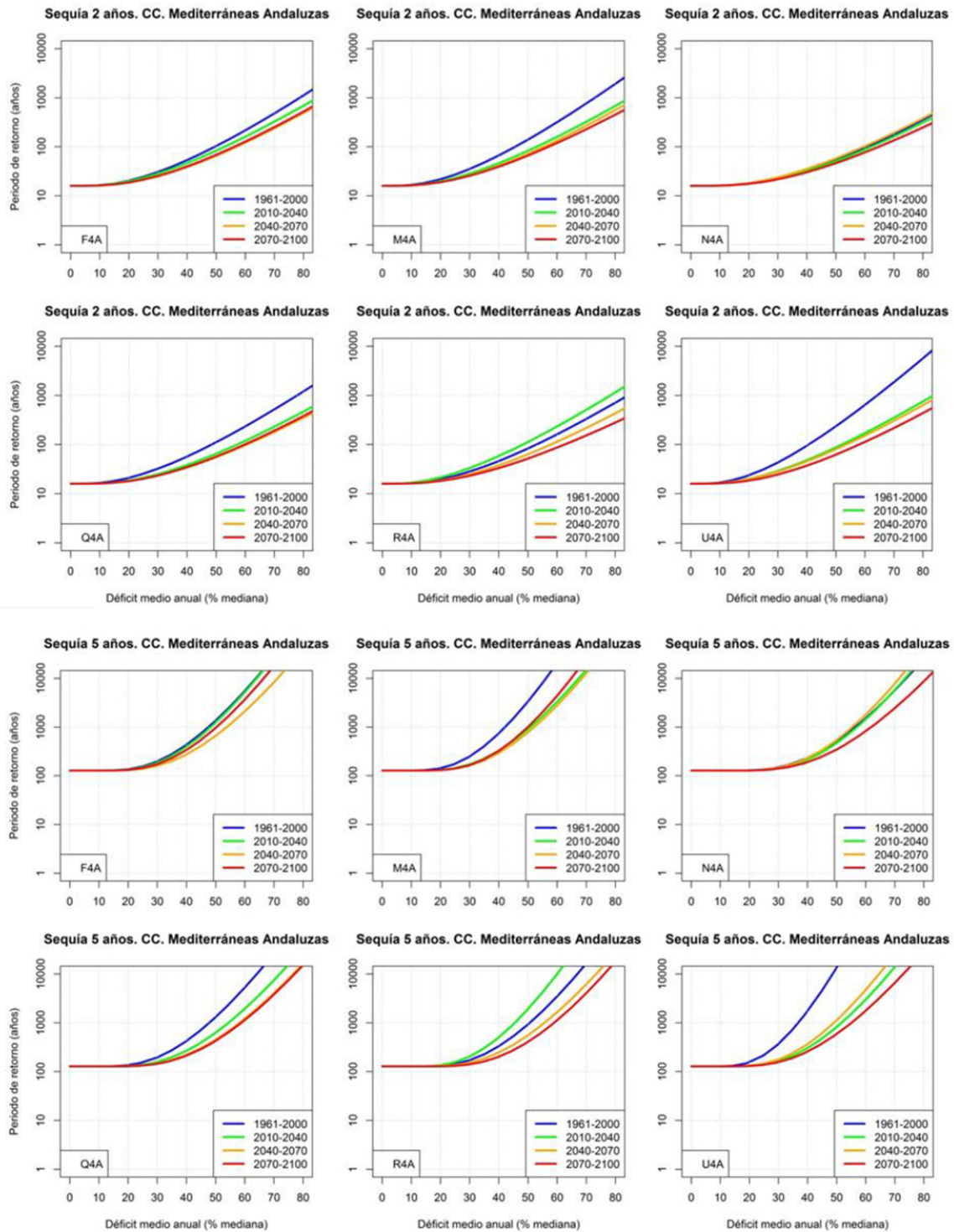
Figura nº 13. Período de retorno de sequías en la DHMA para diferentes déficits medios anuales y duración 2 años (arriba) y 5 años (debajo) para el PC y los tres PI según cada una de las proyecciones. Escenario RCP 4.5
