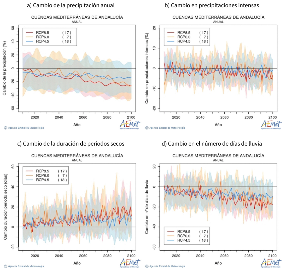
Figura nº 6. Gráficos de cambio en: (a) precipitación anual, (b) precipitaciones intensas, (c) duración de periodos secos y (d) número de días de lluvia en la DHCMA a lo largo del siglo XXI (Fuente: AEMET, 2021)
