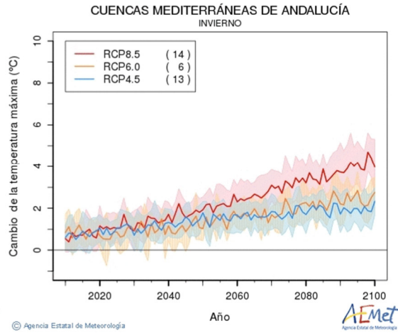
Figura nº 3. Gráficos de cambio de temperatura máxima estacional: (a) primavera, (b) verano, (c) otoño y (d) invierno en la DHCMa a lo largo del siglo XXI (Fuente: AEMET, 2021).
