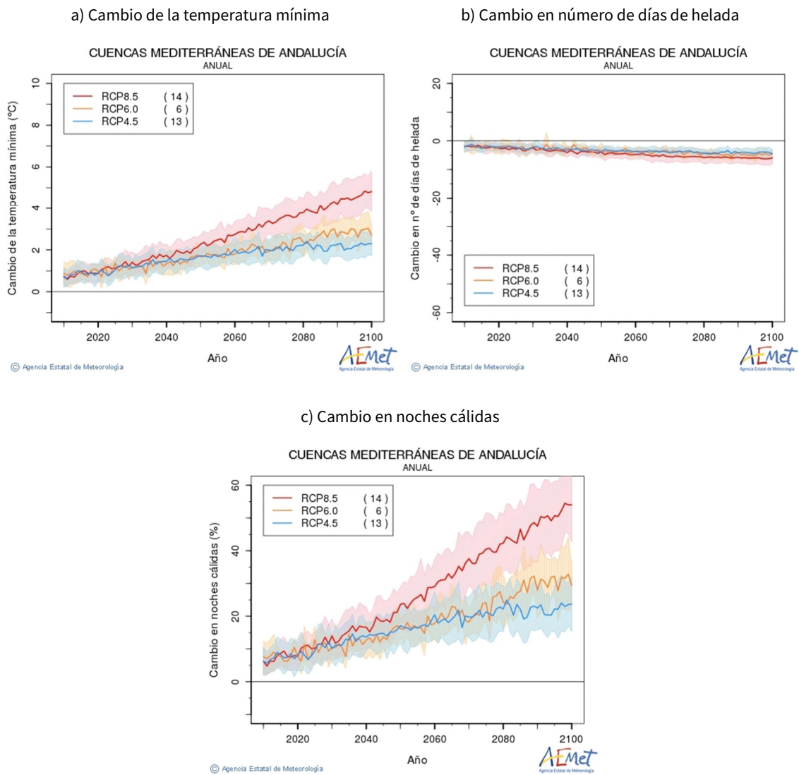
Figura nº 4. Gráficos de cambio en: (a) temperatura mínima, (b) número de días de heladas y (c) noches cálidas en la DHCMA a lo largo del siglo XXI (Fuente: AEMET, 2021).
