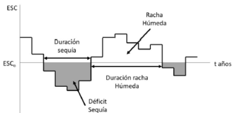
Figura nº 12. Concepto y definición de sequía (CEDEX, 2017)
