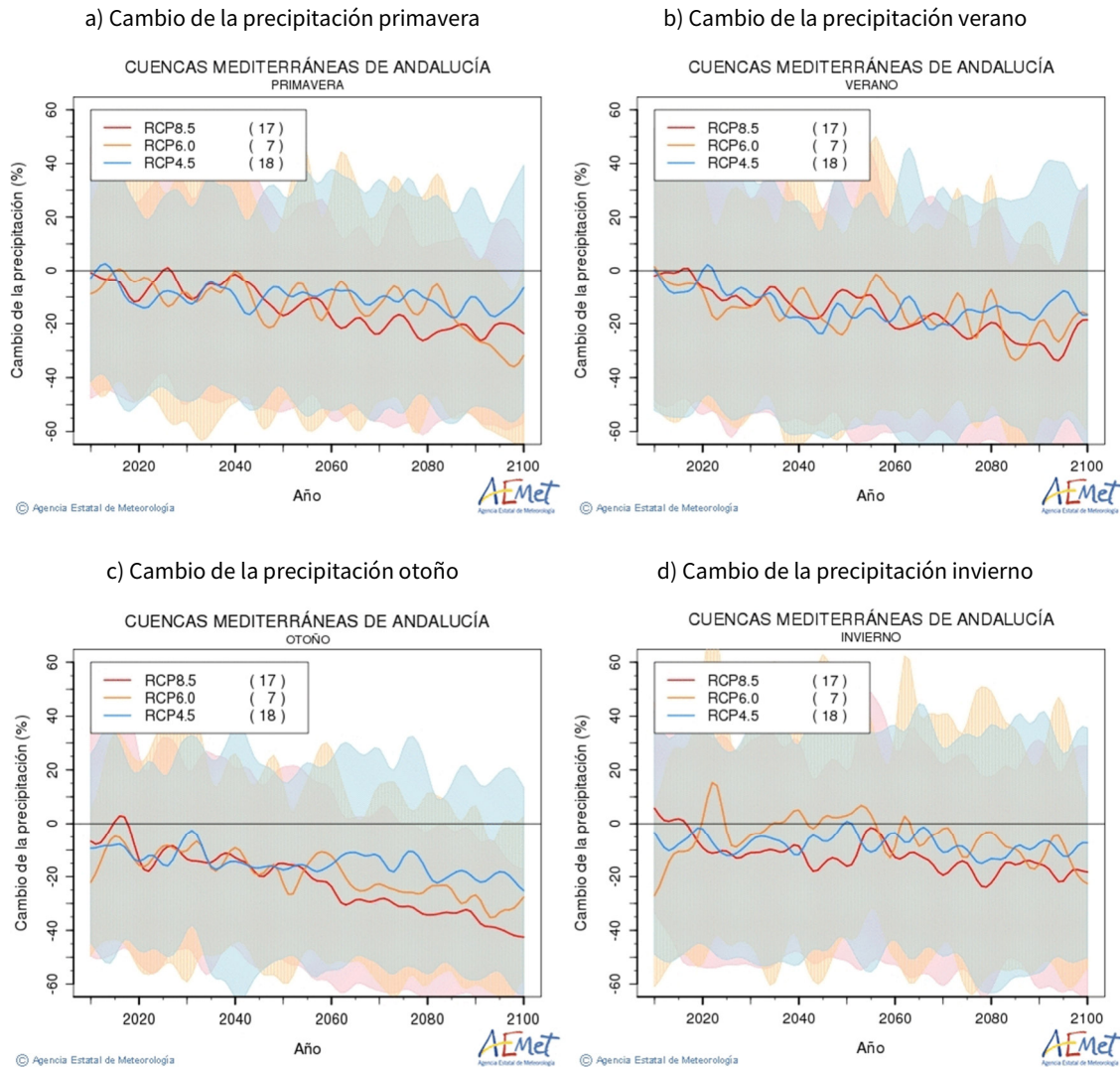
Figura nº 7. Gráficos de cambio de la precipitación estacional: (a) primavera, (b) verano, (c) otoño y (d) invierno en la DHCMA a lo largo del siglo XXI (Fuente: AEMET, 2021).
