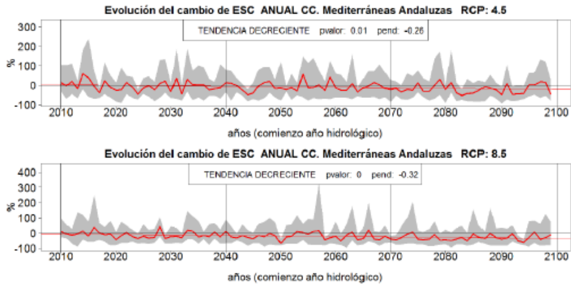
Figura nº 9. Tendencia del \Delta (%) escorrentía del año 2010 al 2099 para los RCP 4.5 (arriba) y 8.5 (abajo) en la DHCMA
