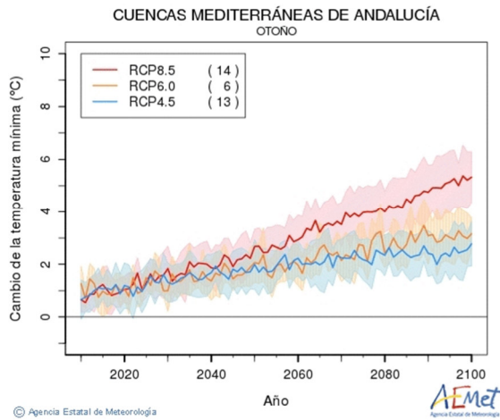
Figura nº 5. Gráficos de cambio de temperatura mínima estacional: (a) primavera, (b) verano, (c) otoño y (d) invierno en la DHCMa a lo largo del siglo XXI (Fuente: AEMET, 2021).
