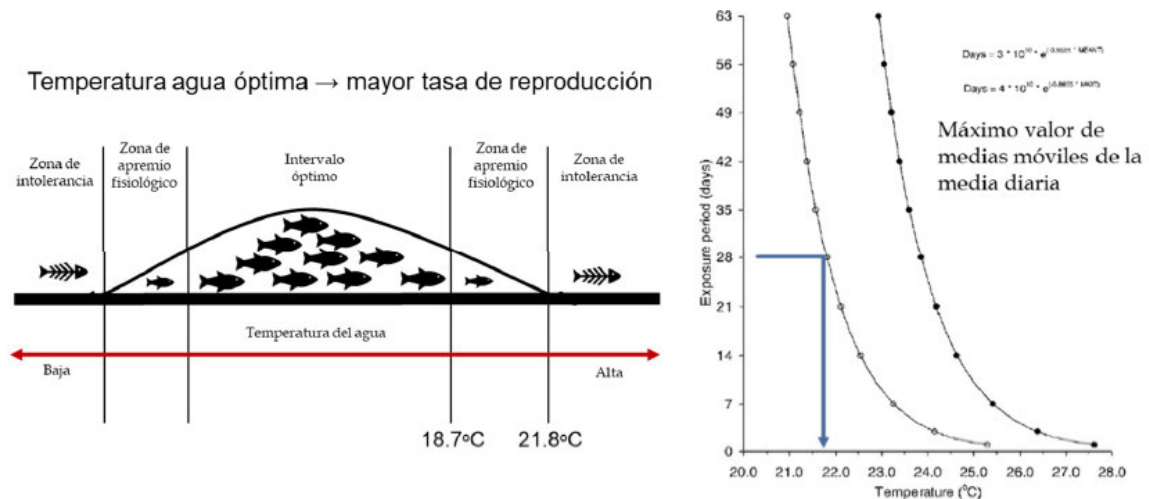
Figura nº 16. Definición de la zona de apremio y de la barrera termal de la trucha común y límites máximos de exposición en días en función de la temperatura media diaria del agua (Wehrly & Wang, 2007).
