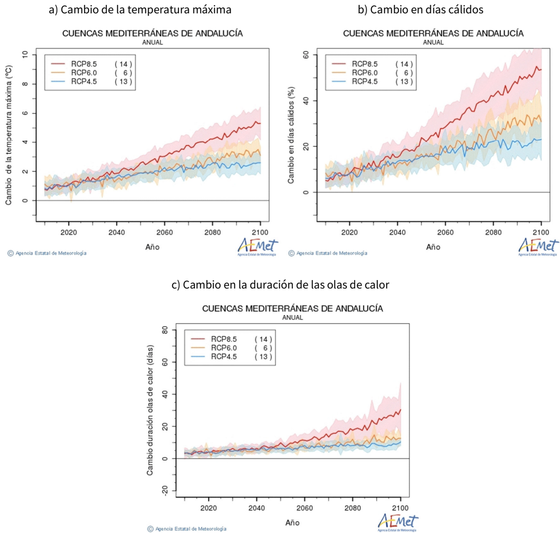
Figura nº 2. Gráficos de cambio de: (a) temperatura máxima, (b) días cálidos y (c) duración de las olas de calor en la DHCMA a lo largo del siglo XXI (Fuente: AEMET, 2021).
