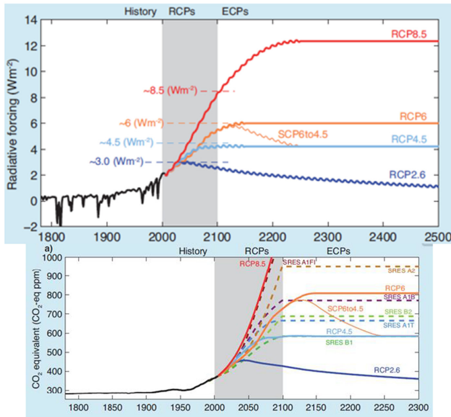
Figura nº 1. Escenarios de emisiones, con indicación del forzamiento radiativo (arriba) y la concentración de CO 2 equivalente en la atmósfera (abajo). (Fuente: IPCC, 2013).
