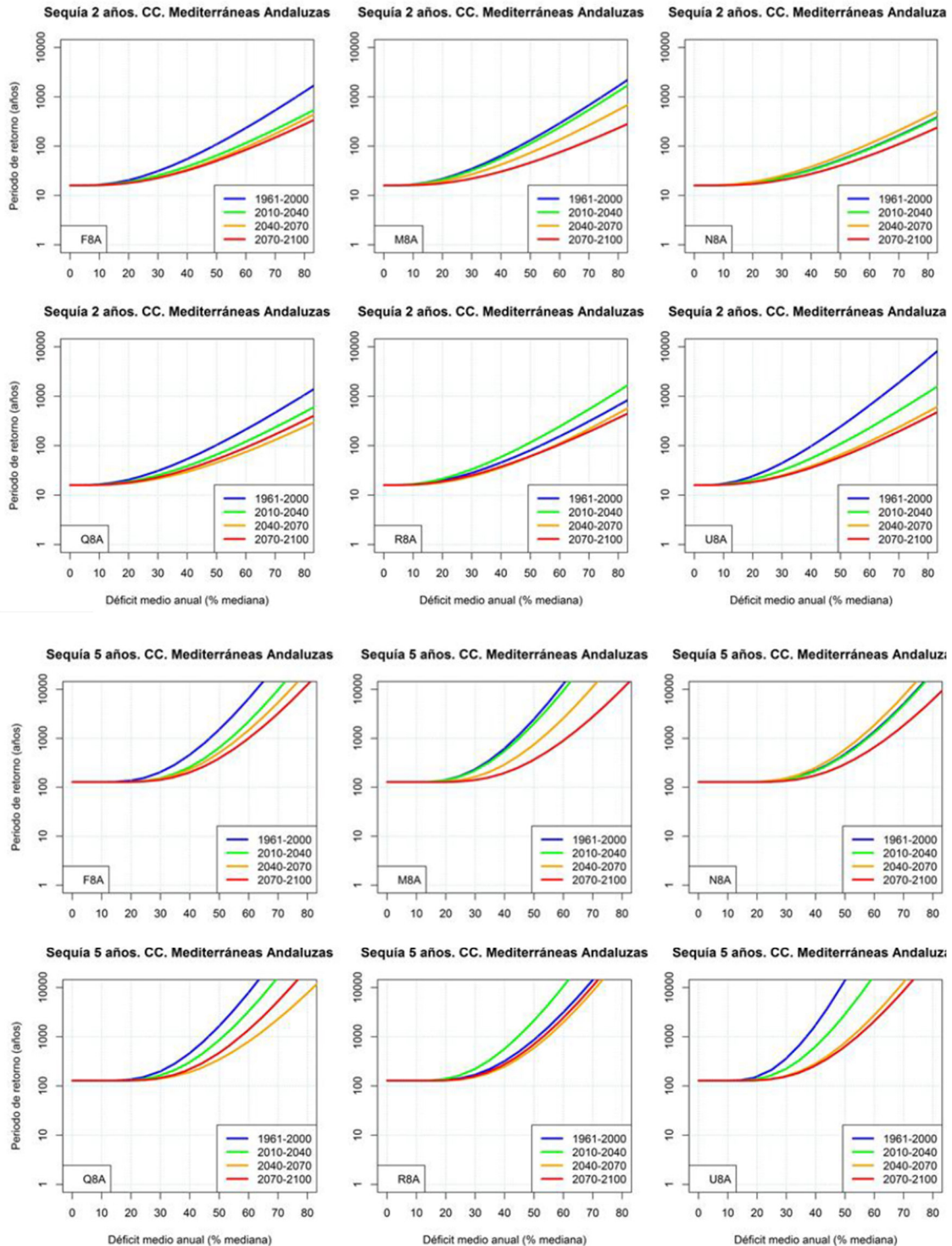
Figura nº 14. Período de retorno de sequías en la DHCMA para diferentes déficits medios anuales y duración 2 años (arriba) y 5 años (debajo) para el PC y los tres PI según cada una de las proyecciones. Escenario RCP 8.5
