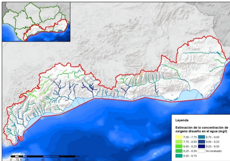
Figura nº 22. Estimación de la concentración de oxígeno disuelto en el agua ( \text{mgO}_2/\text{l} ) calculada en función de la temperatura y la altitud en el mes de agosto
