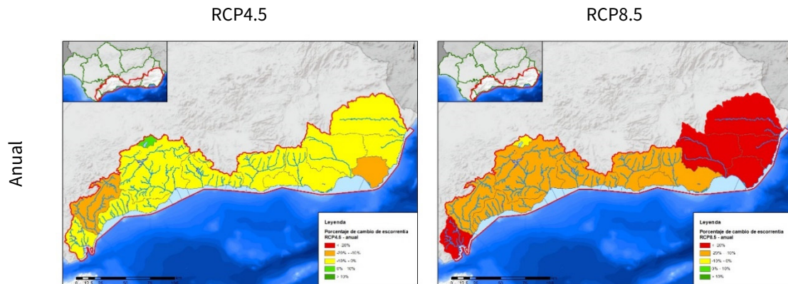
Figura nº 11. Porcentaje de cambio de la escorrentía medio anual por subsistema de explotación en la DHCMA para el horizonte 2039. Escenario RCP4.5(izquierda) y RCP8.5 (derecha). Los colores reflejan la gradación del cambio.
