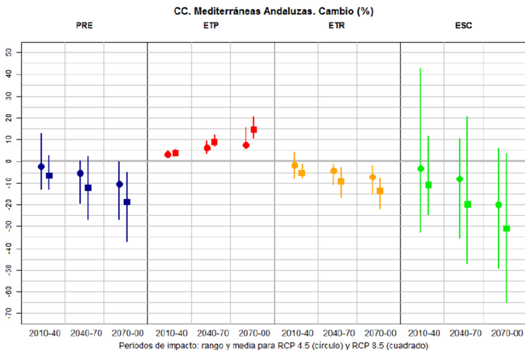
Figura nº 8. Cambio (%) en las principales variables hidrológicas en los tres PI respecto al PC para la DHCMA. Rango y media de resultados para RCP 4.5 (círculos) y RCP 8.5 (cuadrados). Fuente: CEDEX, 2017
