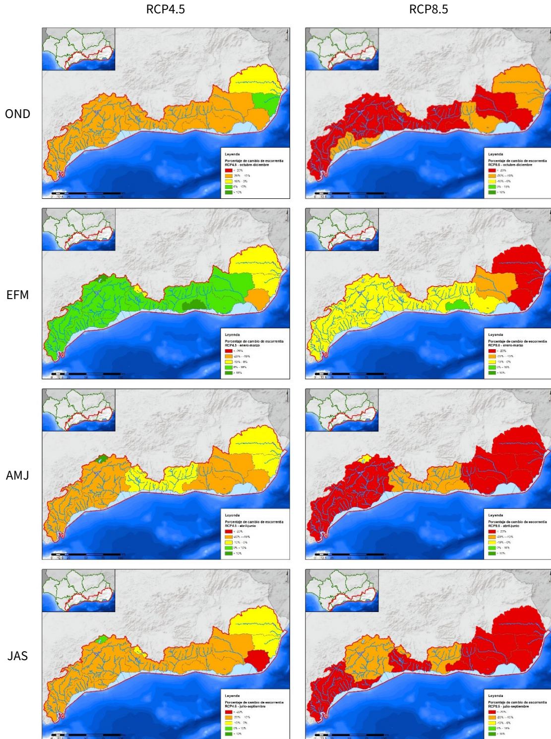
Figura nº 10. Porcentaje de cambio de la escorrentía trimestral (OND, EFM, AMJ, JAS) por subsistema de explotación en la DHCMA para el horizonte 2039. Escenario RCP4.5(izquierda) y RCP8.5 (derecha). Los colores reflejan la gradación del cambio.
