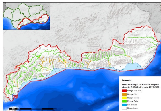
Figura nº 6. Mapas de riesgo en el oxígeno disuelto para los dos escenarios de emisiones RCP4.5 (izquierda) y RCP8.5 (derecha), y los tres PI (2010-2040 arriba, 20140-2070 medio y 2017-2100 abajo)
