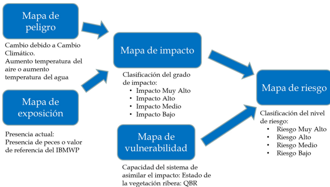
Figura nº 15. Metodología propuesta para la definición del riesgo asociado al cambio climático
