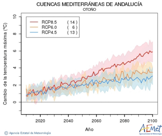
Figura nº 3. Gráficos de cambio de temperatura máxima estacional: (a) primavera, (b) verano, (c) otoño y (d) invierno en la DHCMa a lo largo del siglo XXI (Fuente: AEMET, 2021).
