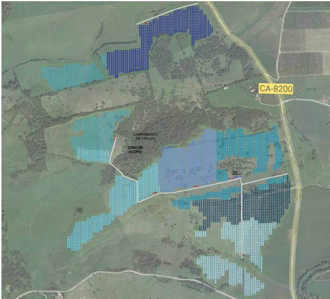
Ilustración 1. Layout general de la planta fotovoltaica
