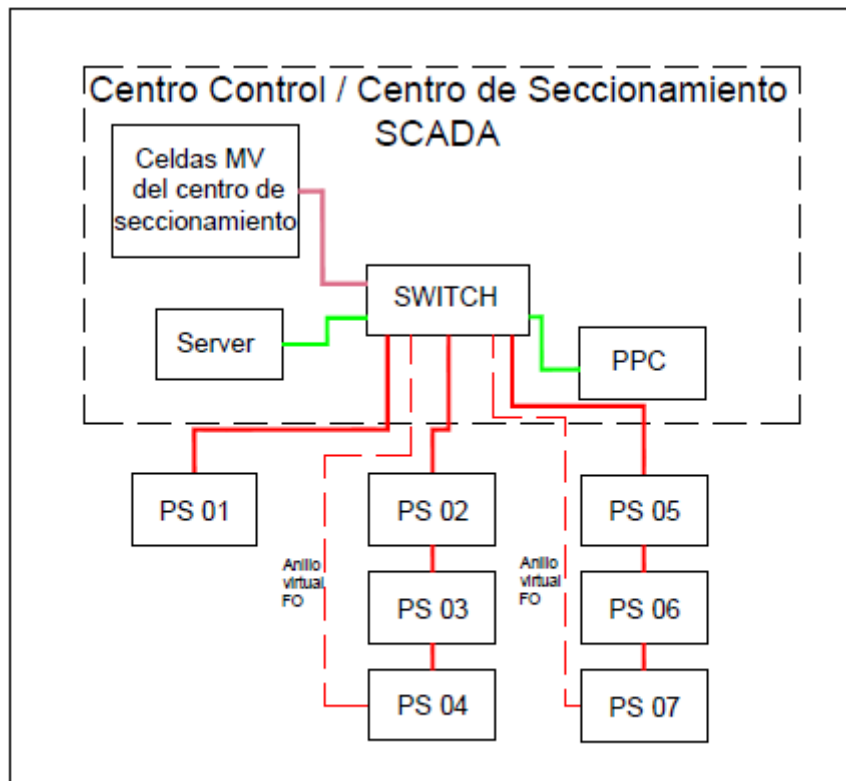
Ilustración 3. Equipos y arquitectura SCADA
