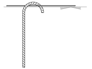
PERFIL DEL ANCLAJE DE LA MALLA AL SUELO POR MEDIO DE GANCHOS Ø12 y 30 cm
