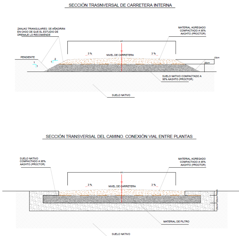
Fig. 4. Sección tipo de viales.
