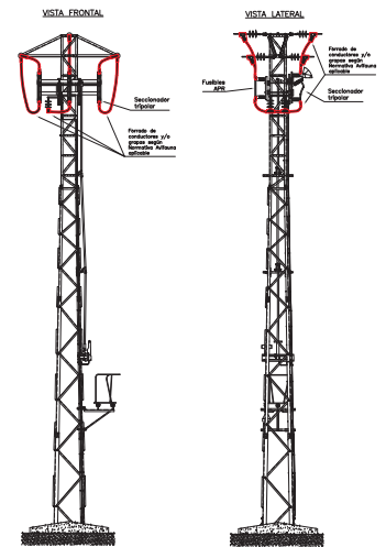
Apoyo privado nº 1: Apoyo con interruptor-seccionador tripolar y fusibles APR
