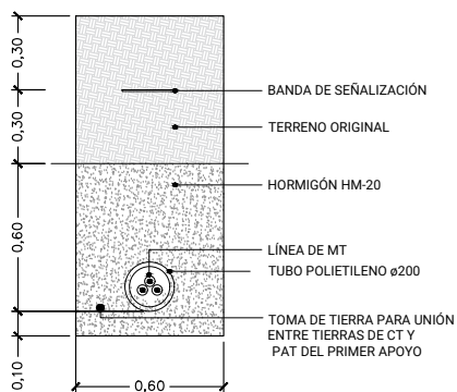
SECCIÓN (1 TERNA)
