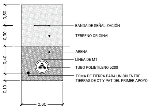
SECCIÓN (1 TERNA)
