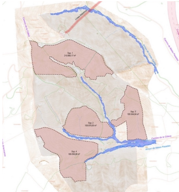
Ilustración 7-Retranqueo de los recintos seleccionados respecto a las zonas inundables
