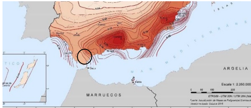
Ilustración 11-Riesgo sísmico
