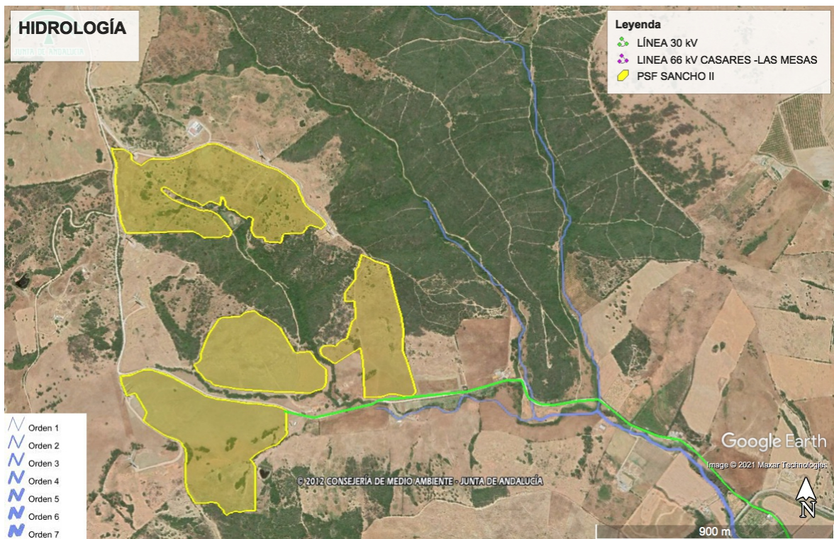
Ilustración 6-Sistema hidrológico
