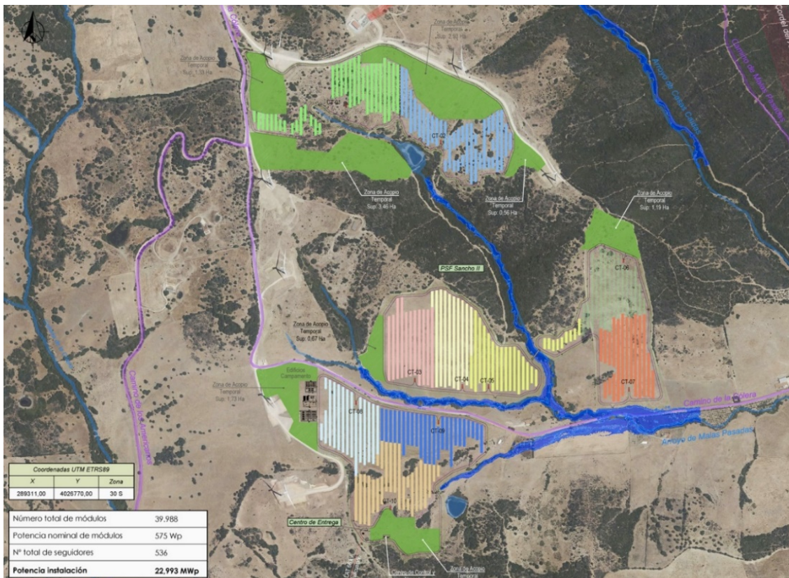
Ilustración 8- Diseño de la planta respecto a las zonas inundables
