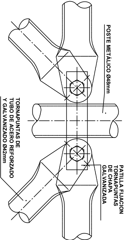
DETALLE A ESCALA 1:3
