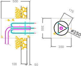
DETALLE - J
