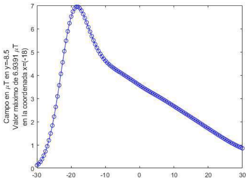
Figura 6: Representación del campo a 1 metro vallado en sentido SUR.
