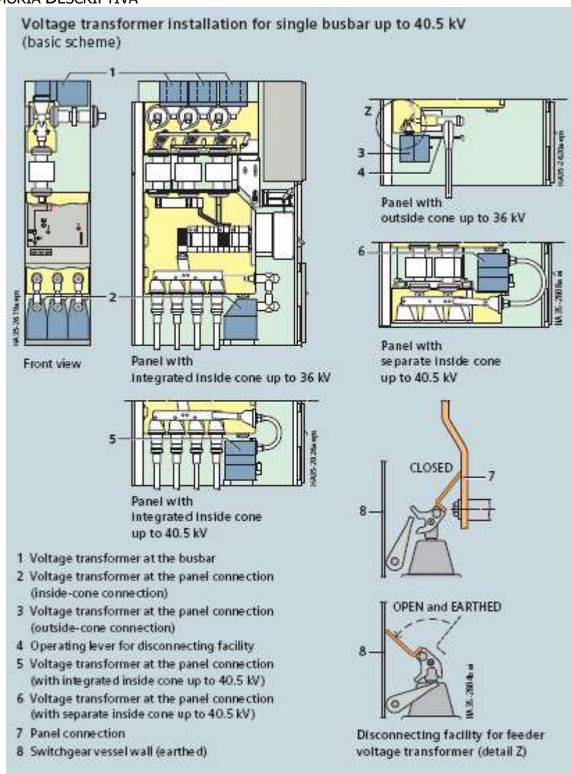
Imagen 3: Instalación del transformador de tensión y del seccionamiento a tierra de la celda.
