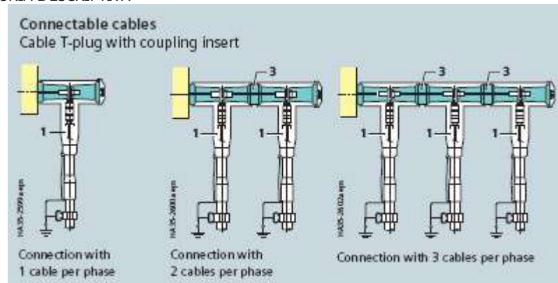
Imagen 5: conexión de hasta 3 cables / botellas por fase en el embarrado de la propia celda.
