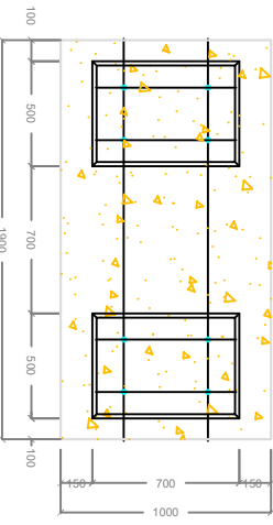
BANCADA EQUIPOS 20 kV
