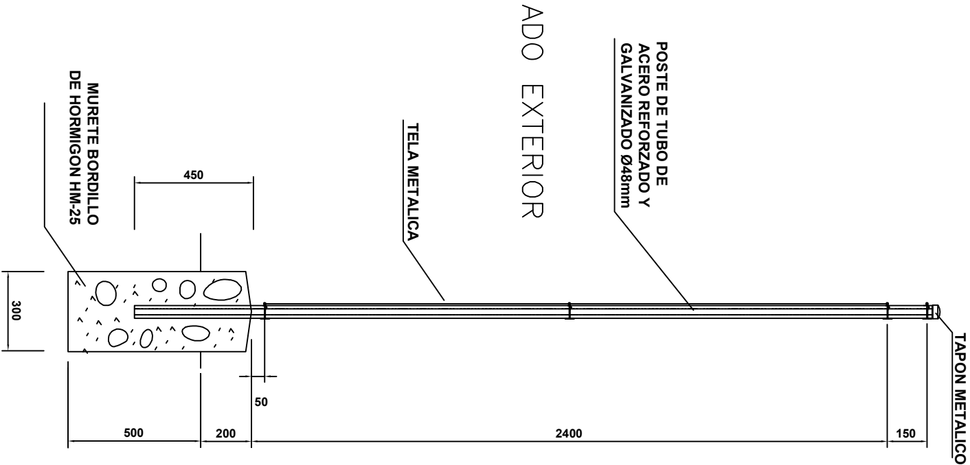
PERFIL
