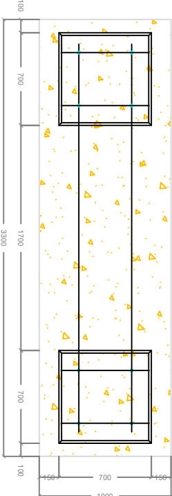
DETALLE - C
