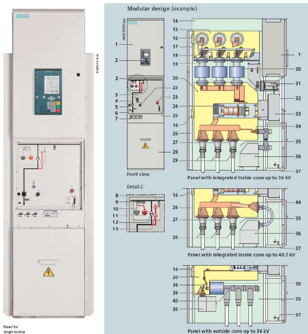
Imagen 1: Frontal e interior de celda. Permite hasta 3 botellas por fase en su conexión.
