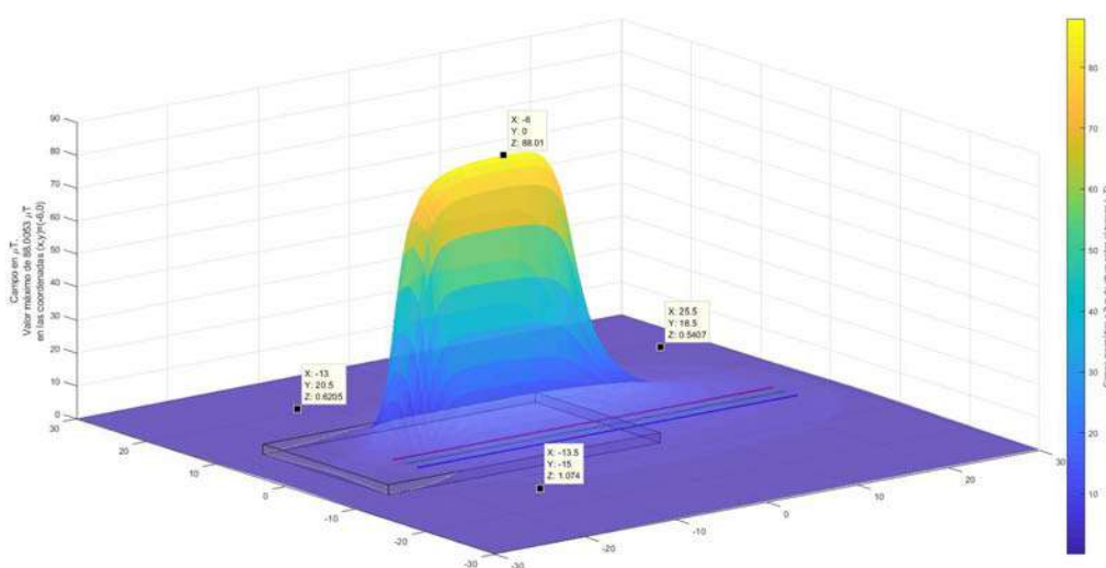
Figura 9: Representación en 3D del campo magnético a 3 metros de altura sobre el terreno.
