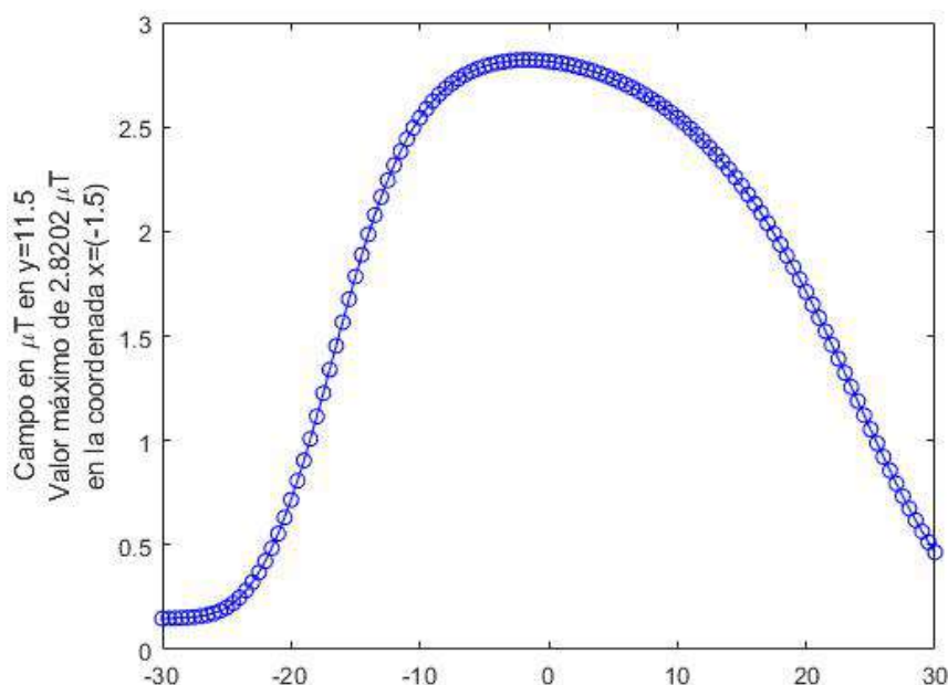
Figura 12: Representación del campo a 1 metro vallado en sentido NORTE.
