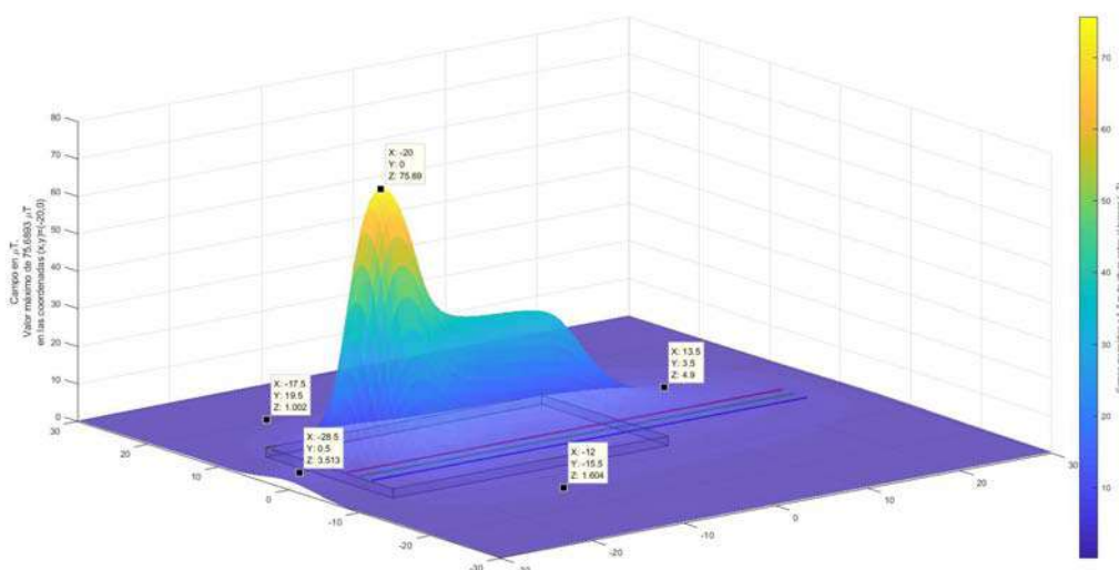
Figura 2: Representación en 3D del campo magnético a 1,7 metros de altura sobre el terreno.
