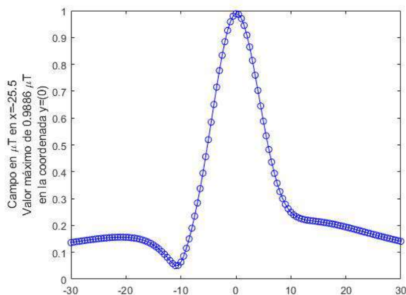
Figura 8: Representación del campo a 1 metro vallado en sentido SUR.
