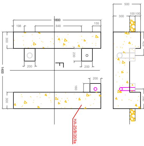
DETALLE - I
