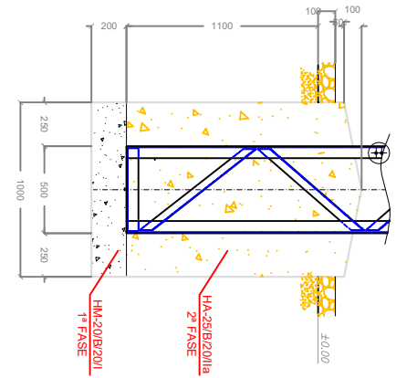
DETALLE - D
