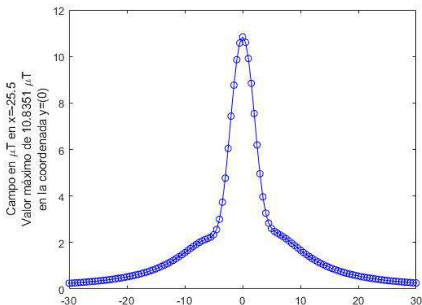
Figura 7: Representación del campo a 1 metro vallado en sentido NORTE.
