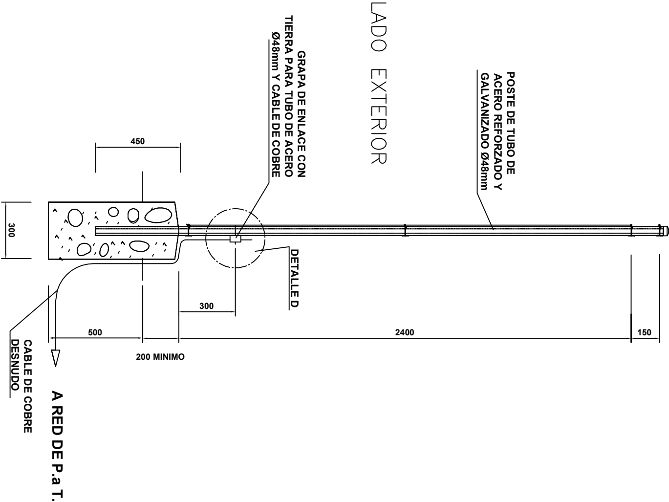
SECCION DETALLE DE P.a.T.
