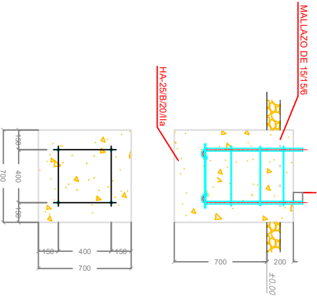
DETALLE - A
