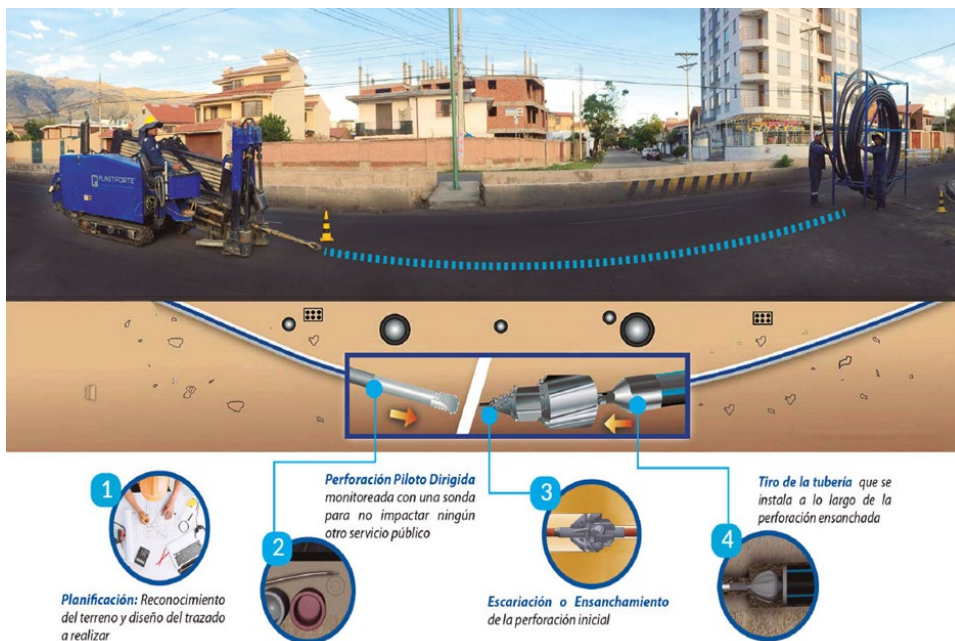
FIGURA 7: perforación dirigida
