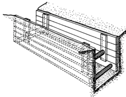
ENTIBACIÓN CUJADA
