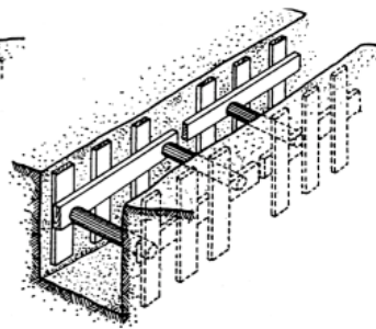
ENTIBACIÓN SEMICUJADA
