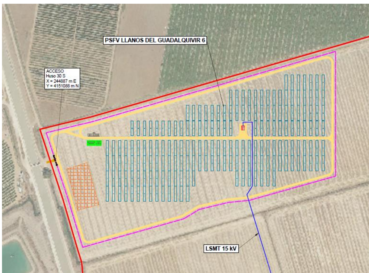
Figura 3. Accesos a la Planta Solar FV
