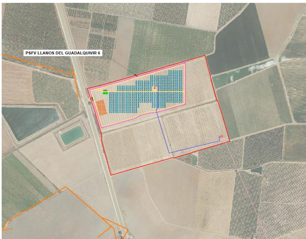
Figura 10. Localización línea eléctrica
