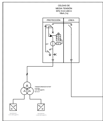
SKID MT PSFV Llanos del Guadalquivir 6
