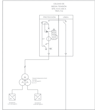
SKID MT PSFV Llanos del Guadalquivir 3 (Objeto de otro proyecto)
