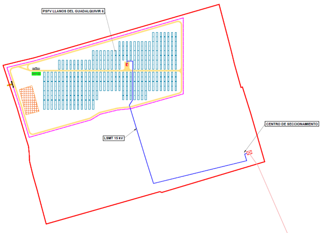
Figura 17: Planta Solar FV.
