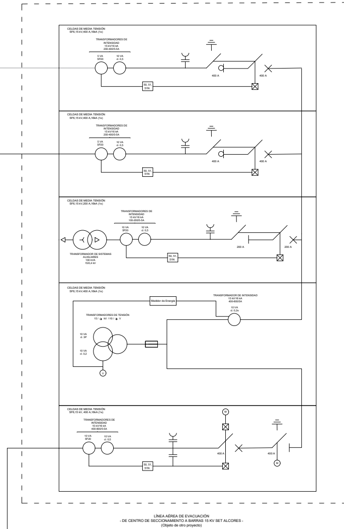
CENTRO DE SECCIONAMIENTO (Objeto de otro proyecto)
