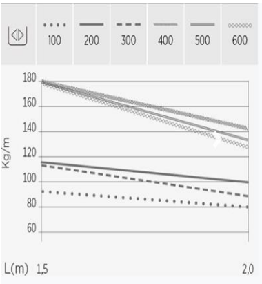
Imagen 1:Diagrama de Cargas Bandejas.
