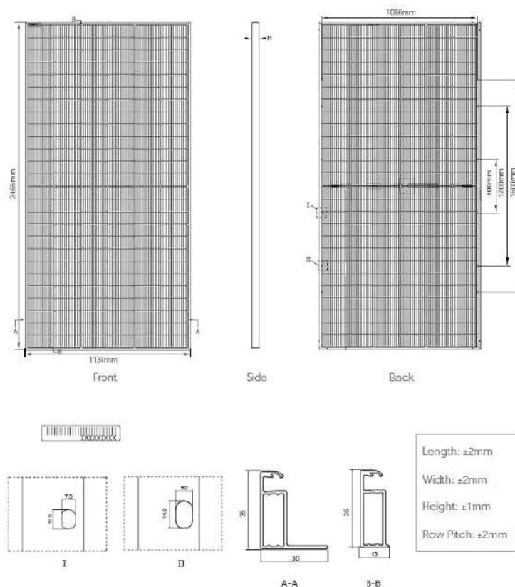
Figura 2.2. Dimensiones del módulo.
