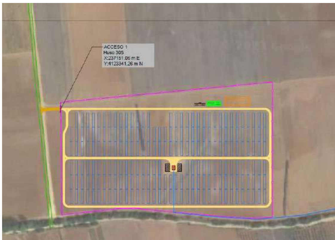
Figura 2.1. Acceso principal a la Planta Solar.
