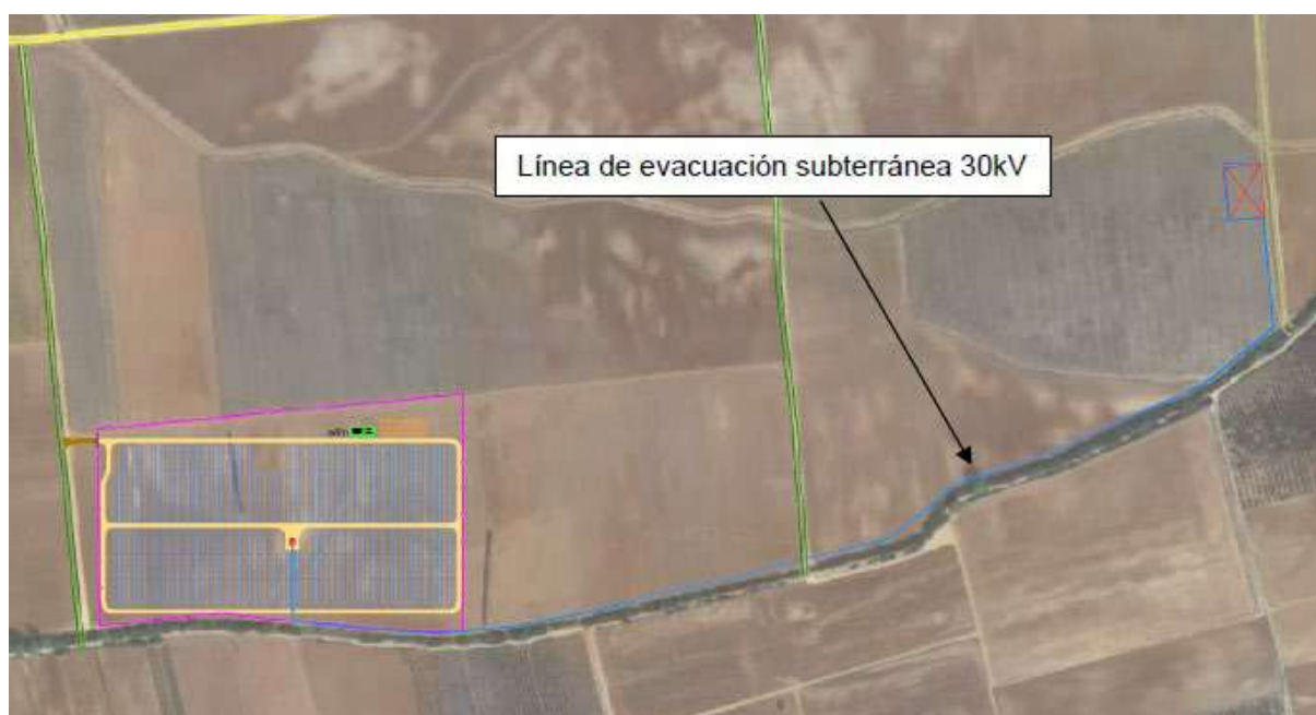
Figura 2.4. Disposición de la LSMT a 30 kV.
