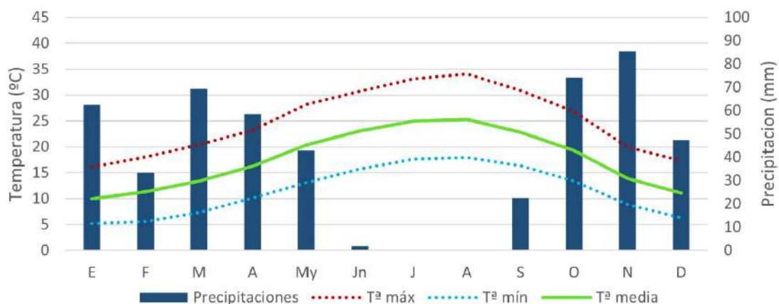
Figura 3.4. Diagrama termopluiométrico histórico en el entorno del Proyecto (periodo 2011-2021).
