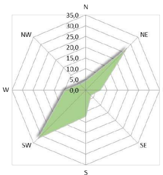
Figura 3.8. Rosa de los vientos en el entorno del Proyecto elaborada a lo largo del periodo 2011 – 2021.
