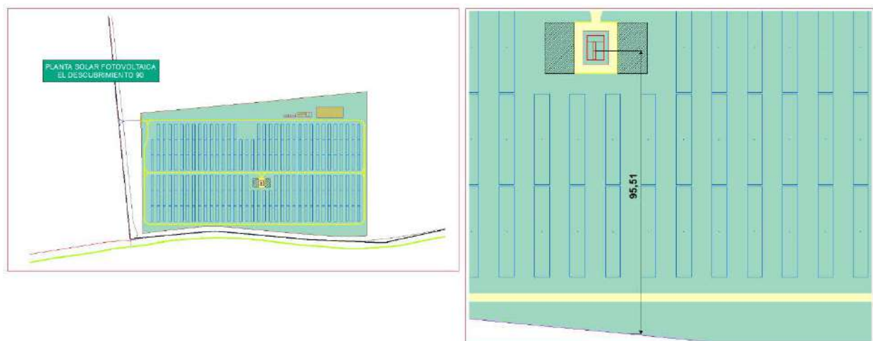
Figura 2.3. Ubicación de la estación de potencia dentro de la parcela de la Planta solar "El Descubrimiento 90".
