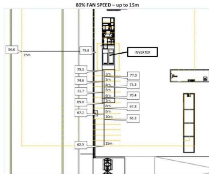
Figura 2.2. Datos de emisión sonora alrededor de la estación de potencia. Fuente: Ficha técnica adjunta.
