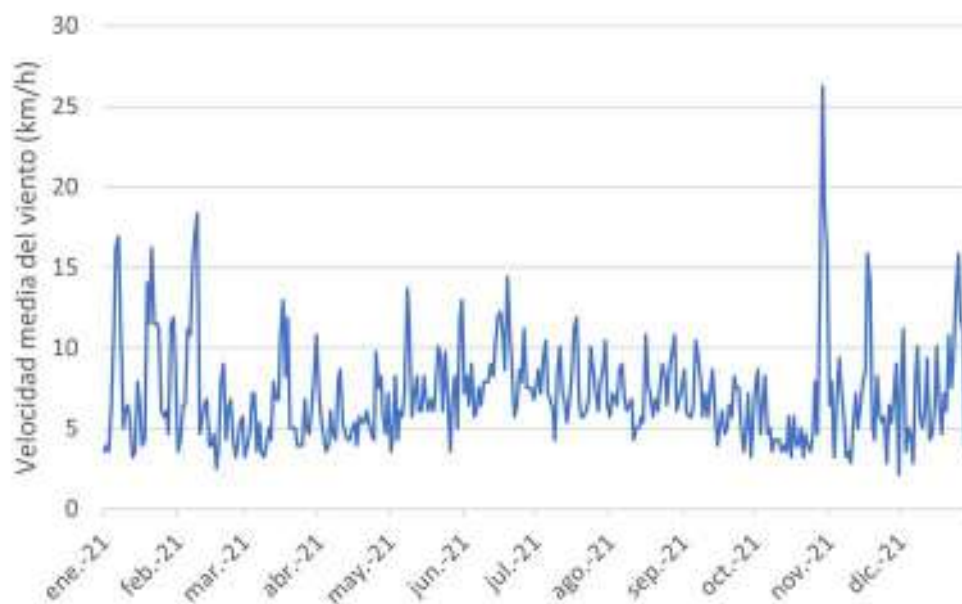
Figura 3.7. Velocidad media máxima del viento (km/h) en el entorno del Proyecto (año 2021).
