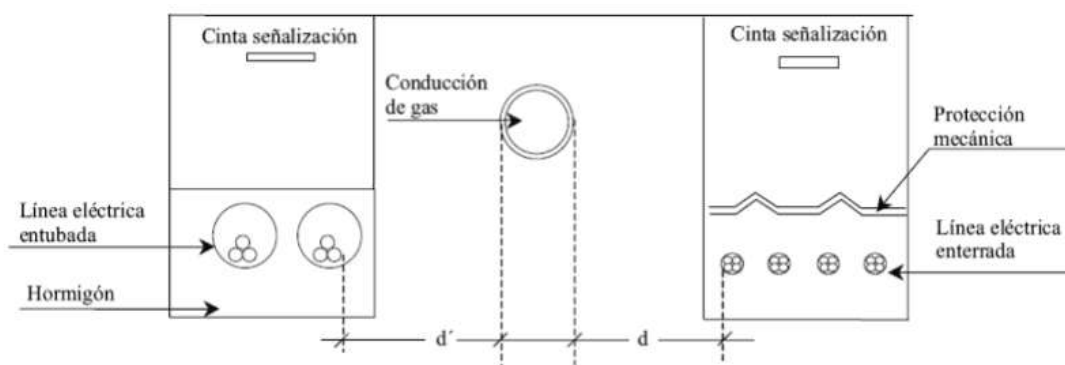
Figura 30: Detalles de paralelismo y conducciones (ITC-LAT 06).
