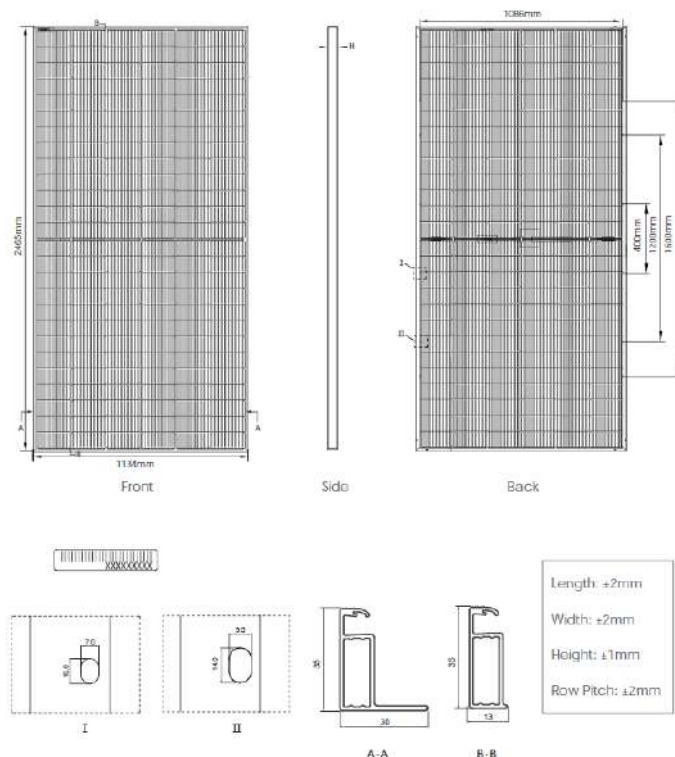
Figura 21: Dimensiones del Módulo.
