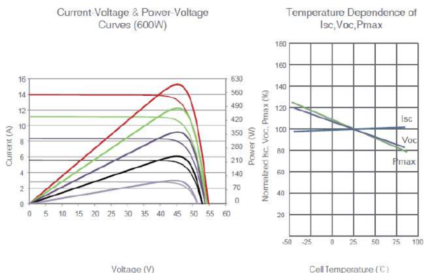
Figura 22: Curvas Características JKM600N-78HL4.
