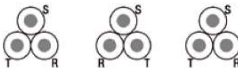
Figura 25: Colocación de cables en tresbolillo.
