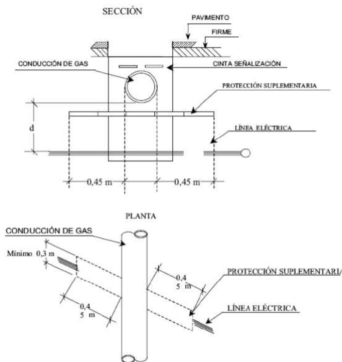
Figura 28: Detalles de cruzamiento y conducciones (ITC-LAT 06).
