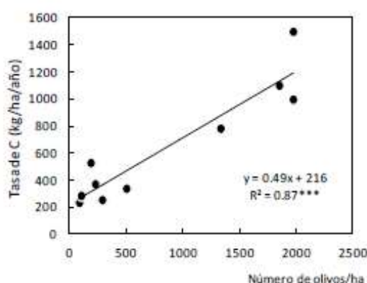
Figura 2. Modelo predictivo de la tasa anual de acumulación de carbono en olivar, en función del número de árboles /hectárea
