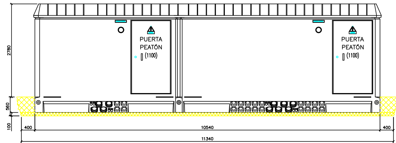
VISTA DELANTERA
