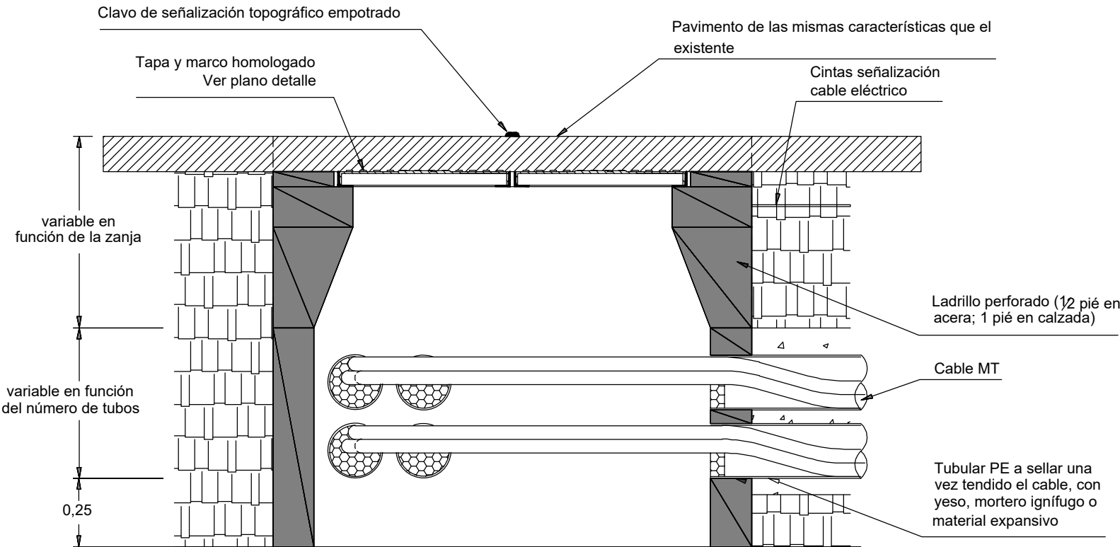
SECCIÓN A-A'
