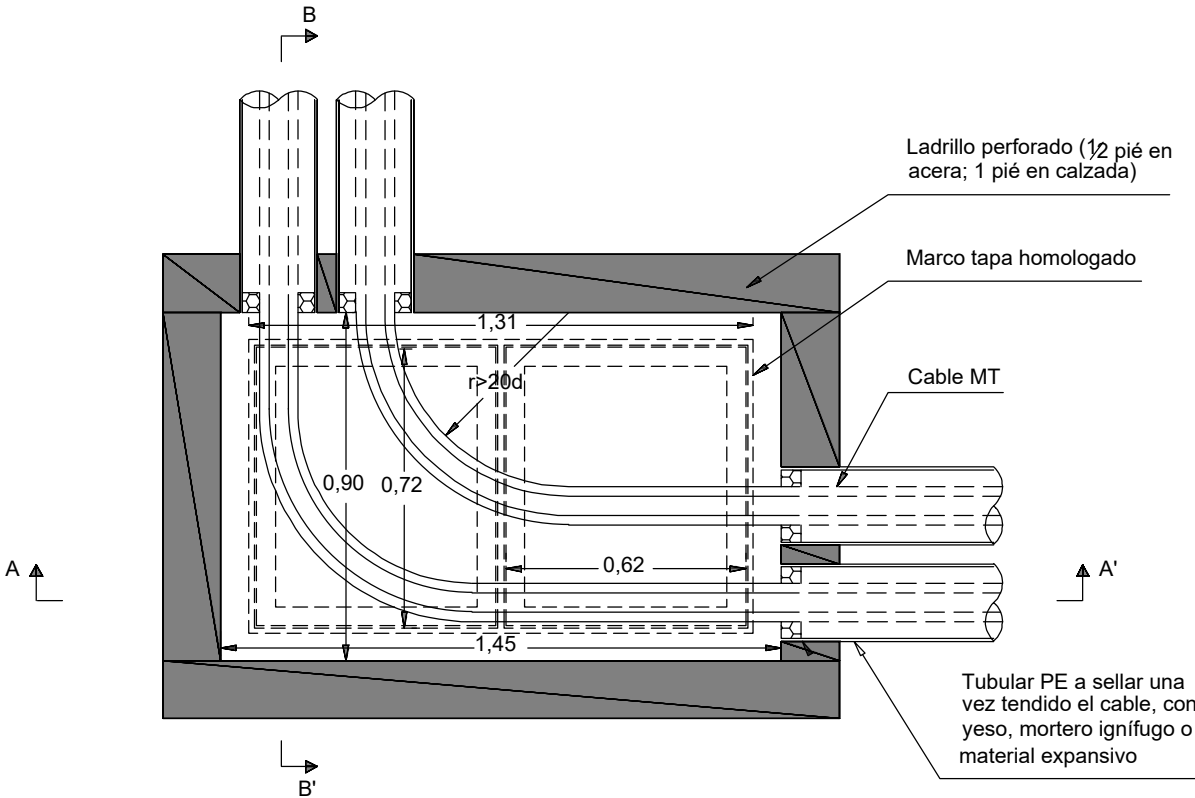
PLANTA
