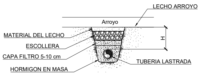
SECCION A-A. LASTRADO CONTINUO
