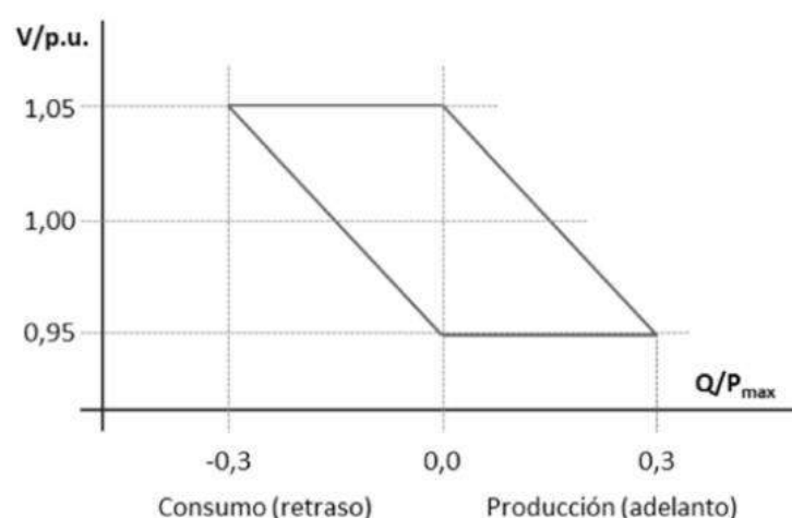
Ilustración 8: Diagrama U-Q/P de un módulo de generación de electricidad síncrono tipo C cuando P_{max} < 15 MW.
