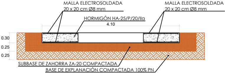
SECCIÓN B-B'
