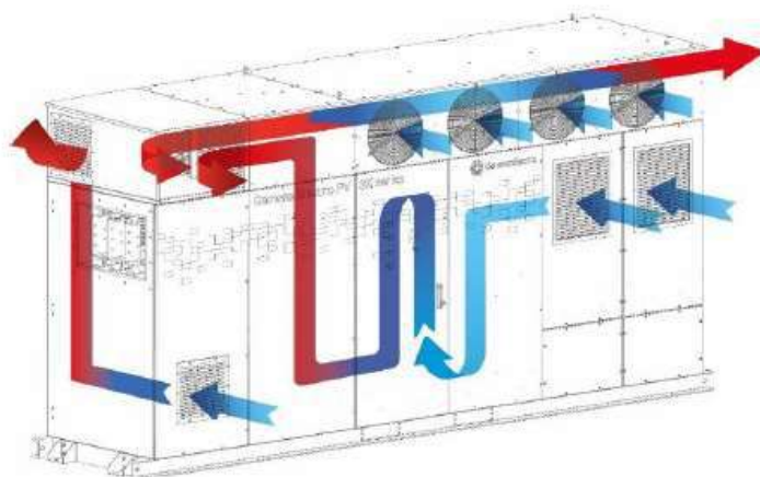
Ilustración 4: Flujos de aire en el PV 3X Gamesa Electric
