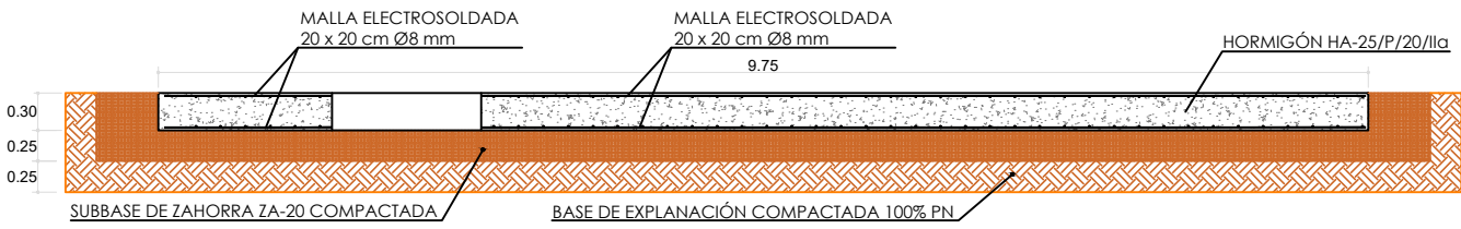
SECCIÓN A-A'
