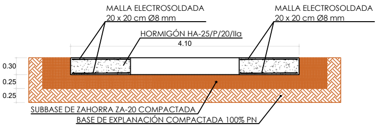
SECCIÓN B-B'
