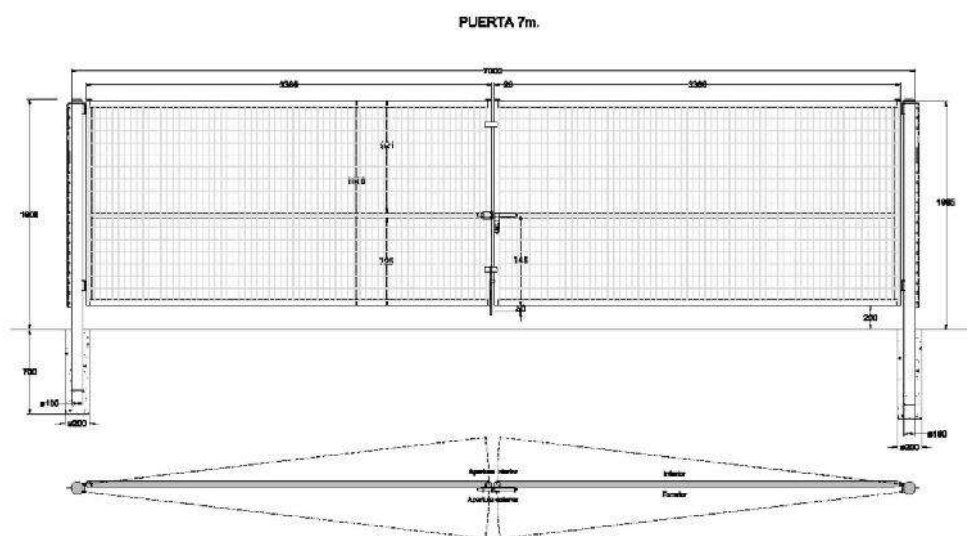
Ilustración 15: Plano de la puerta de acceso.
