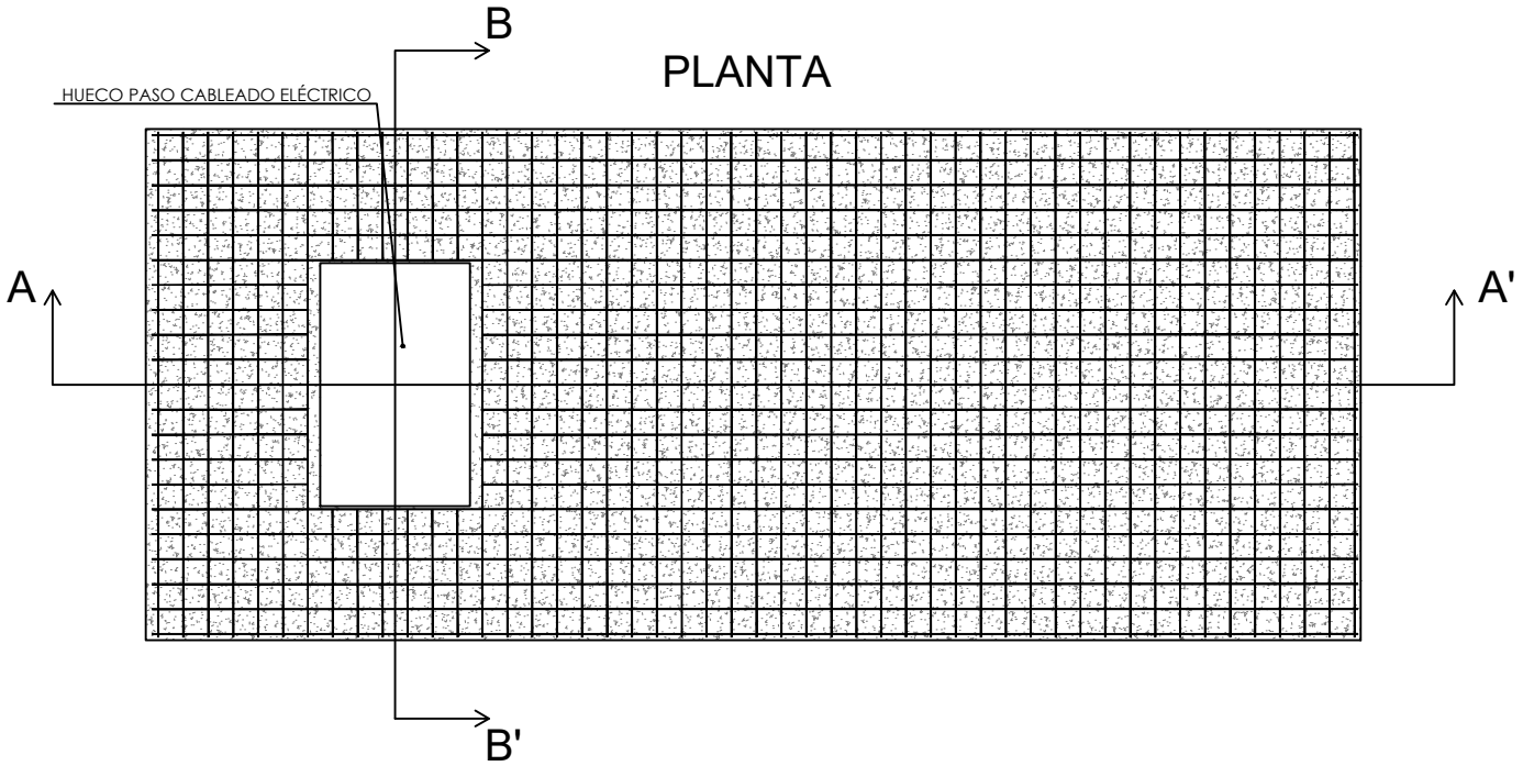
CIMENTACIÓN STATCOM
