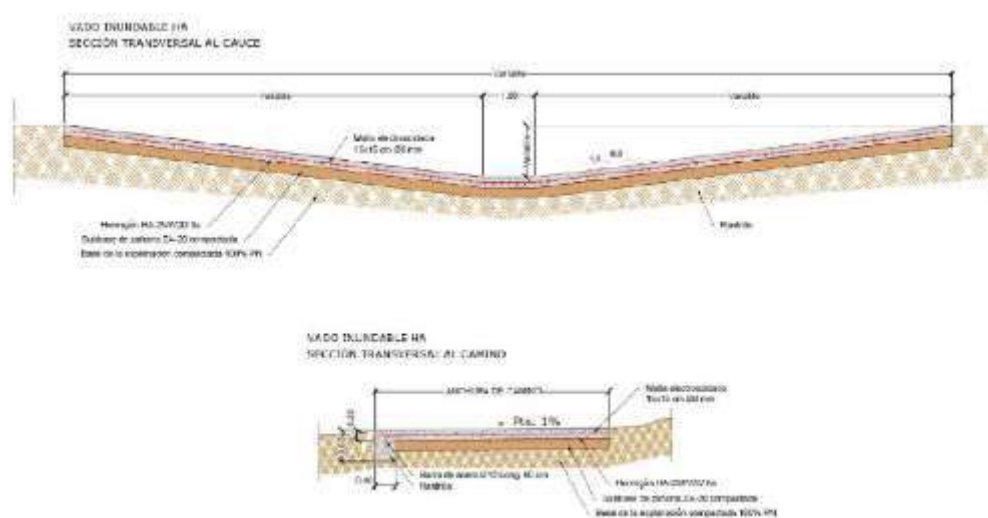
Ilustración 12: Acondicionamiento de vado existente.
