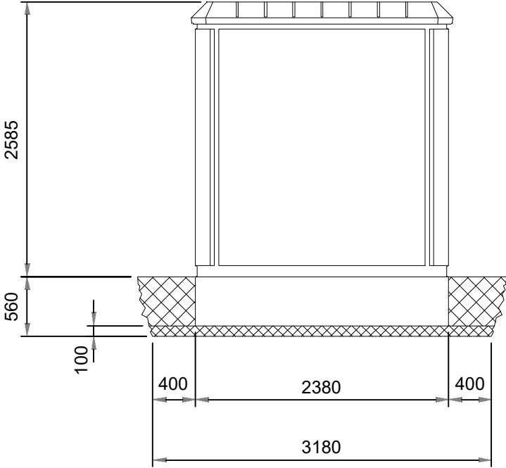
VISTA LATERAL
