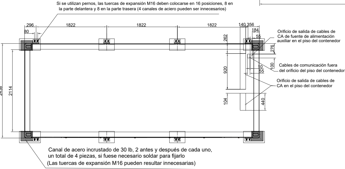
Sección A-A
